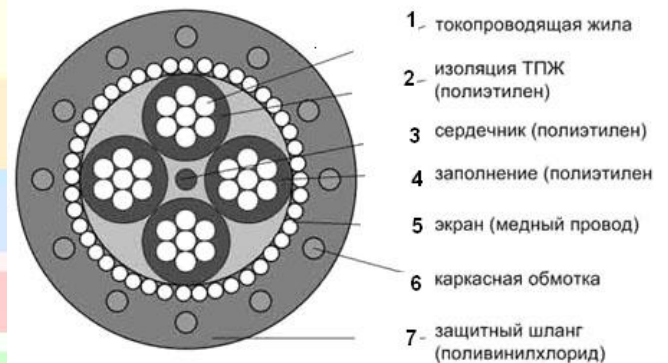
Устройство кабеля П-296
