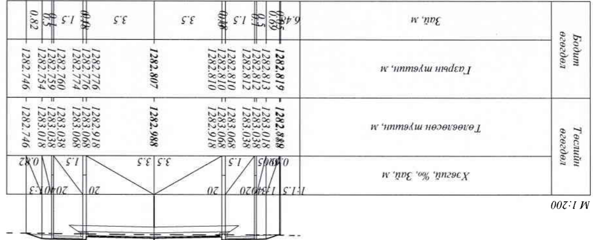
PK 7+20.000
