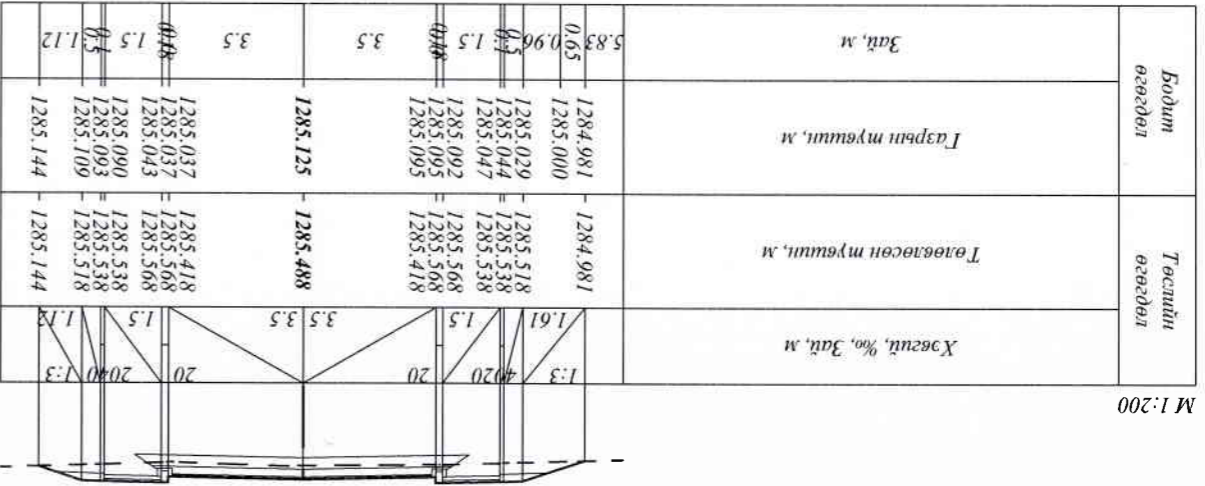
PK 9+40.000
