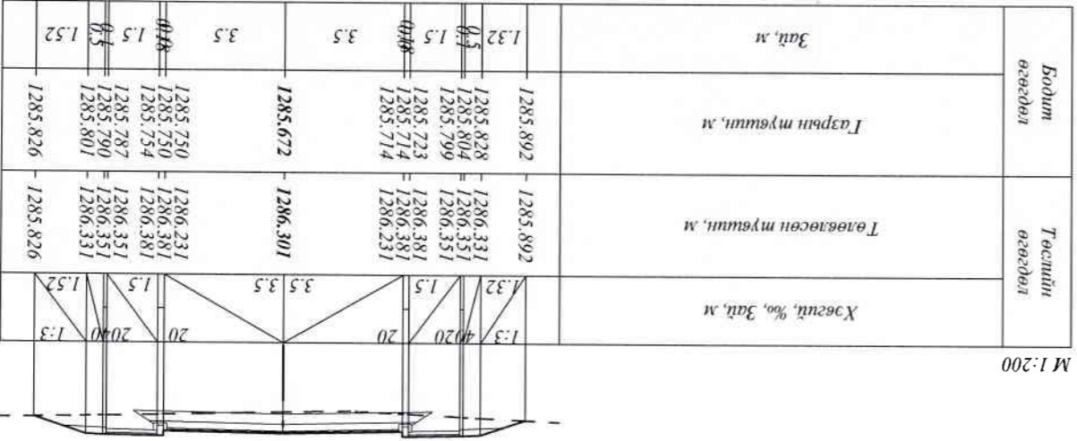
PK 10+20.000
