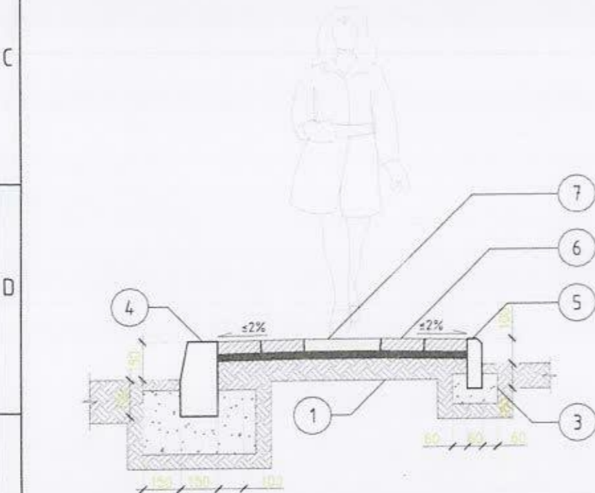
ЗАМЫН ЭРГЭЛТИЙН ЖИШЭЭ ЗУРАГ
