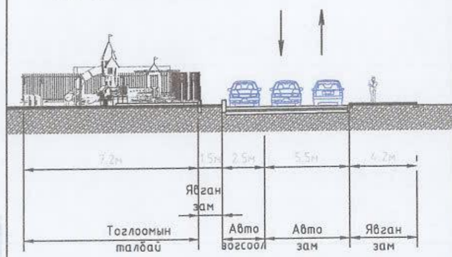
ЗАМ ТАЛБАЙН ОГТЛОЛ 1-1
