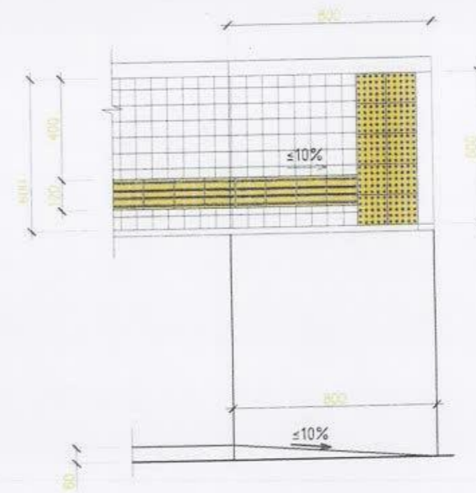
ЯВГАН ЗАМЫН ӨНГӨТ ХАВТАНГЫН ӨРӨЛТИЙН ЖИШЭЭ ЗУРАГ
