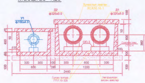
Сувгийн огтлол 1-1 масштаб 1:20
