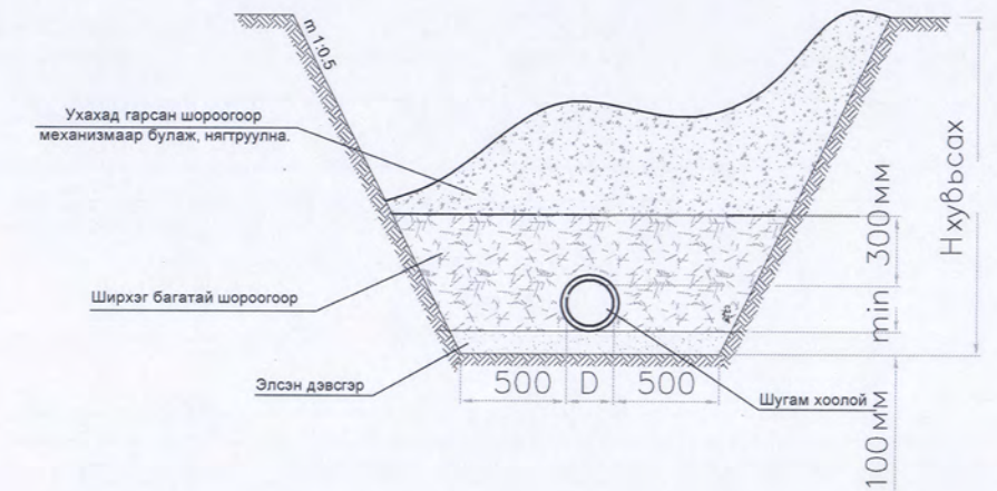
СУВГИЙН ОГТЛОЛ / Төрөл 3 /
