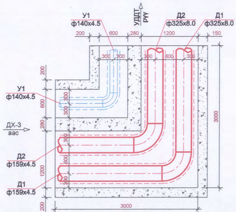
Эргэлтийн өнцөг ЭӨ-1-ийн байгуулалт масштаб 1:40
