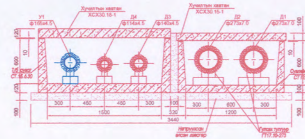
Сувгийн огтлол 2-2 масштаб 1:20
