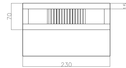
дээрээс харсан байдал
