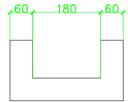
Ус зайлуулах сувгийн тэвш
