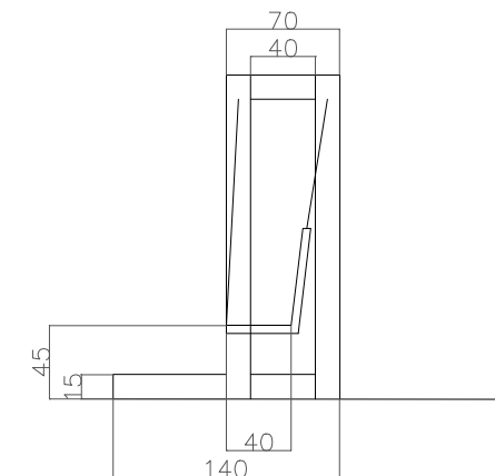
хажуугаас харсан хэсэг
