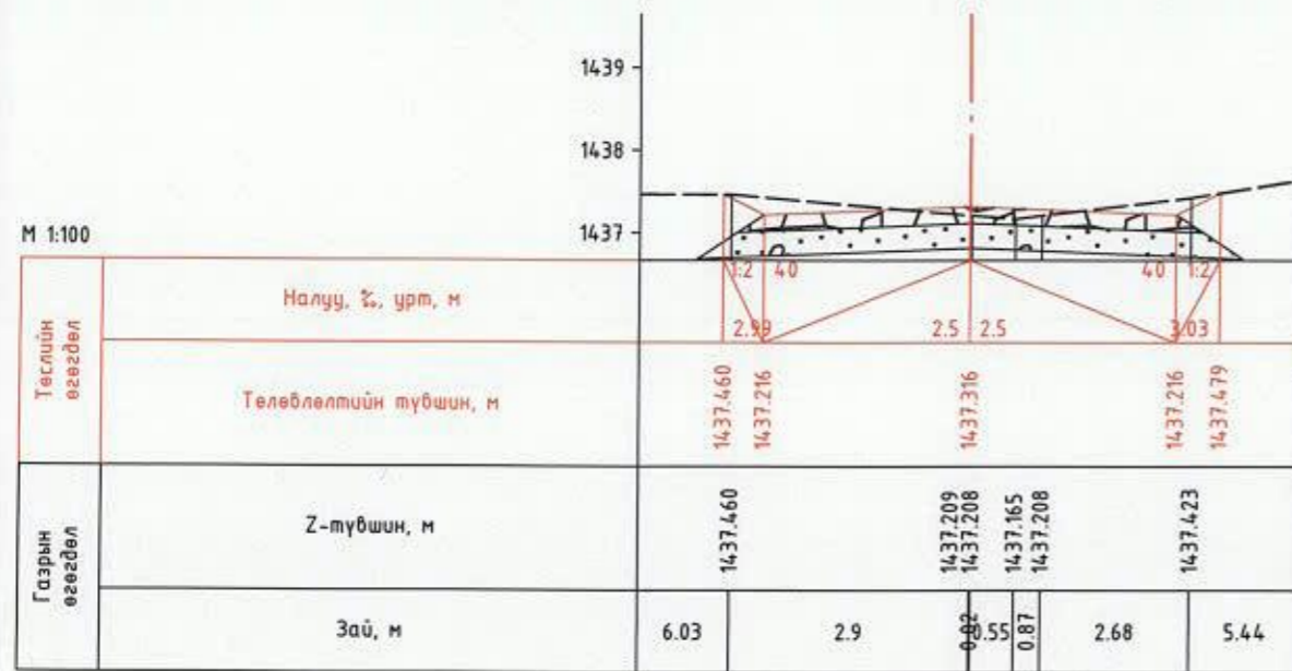
ПК 0+520.00
