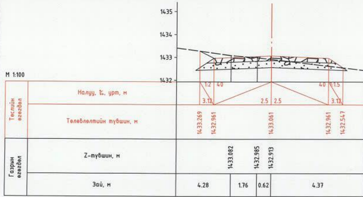
ПК 0+480.00
