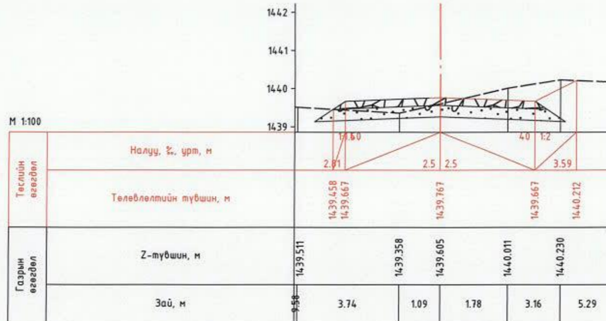
ПК 0+540.00
