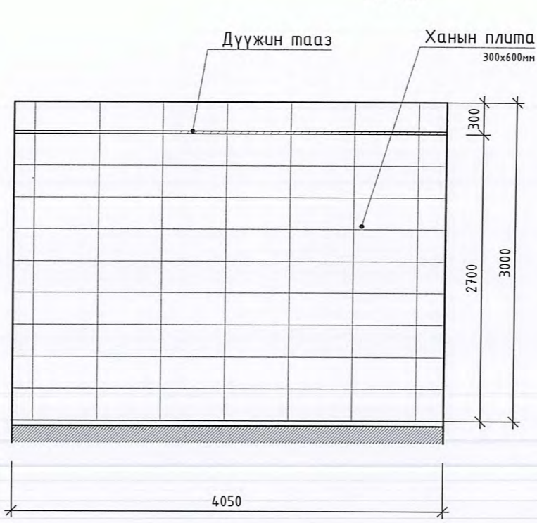
Ханын дэлгээс Х-2 M1 : 50
