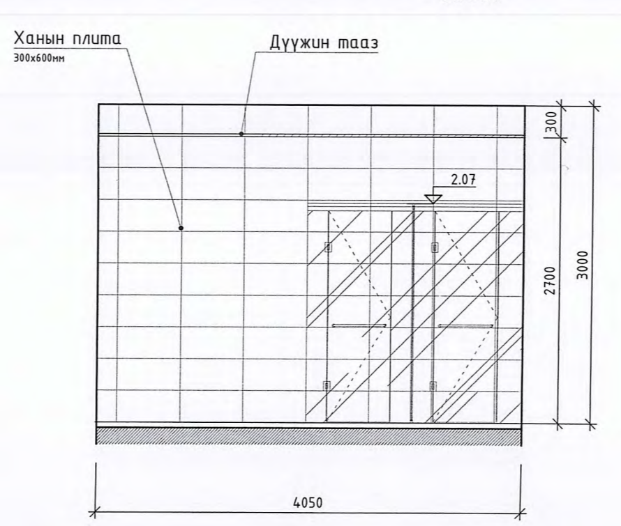
Ханын дэлгээс Х-4 M1 : 50
