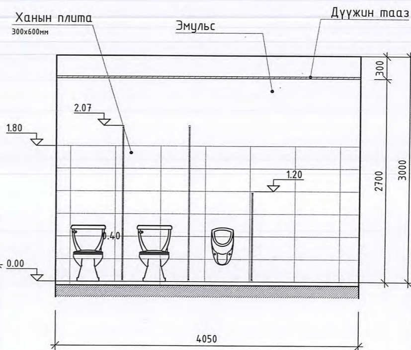
Ханын дэлгээс Х-2 M1 : 50
