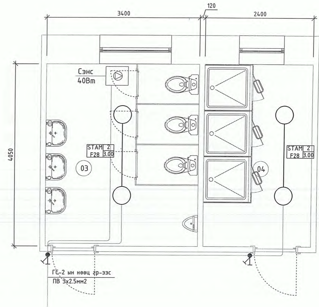
2-р давхрын өөрчлөлтийн дотор гэрэлтүүлгийн хэсэгчилсэн байгуулалт-2
