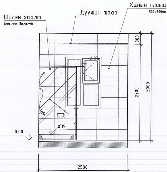
Ханын дэлгээс Х-1 М1 : 50
