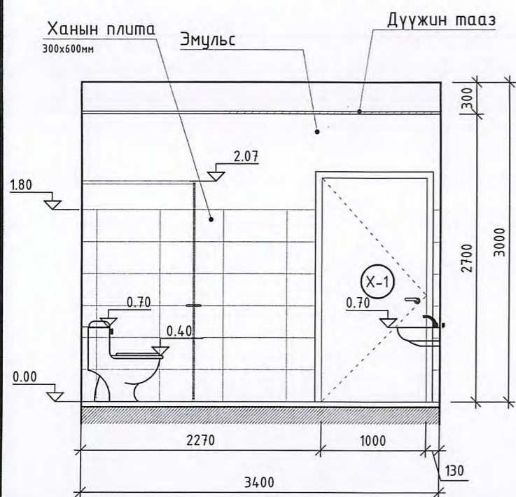
Ханын дэлгээс Х-3 M1 : 50
