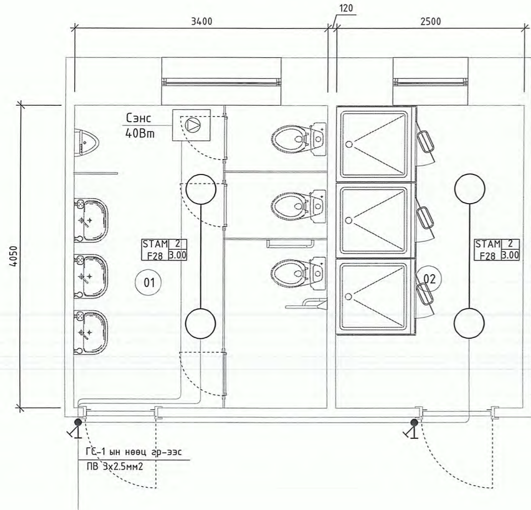
1-р давхрын өөрчлөлтийн дотор гэрэлтүүлгийн хэсэгчилсэн байгуулалт-1
