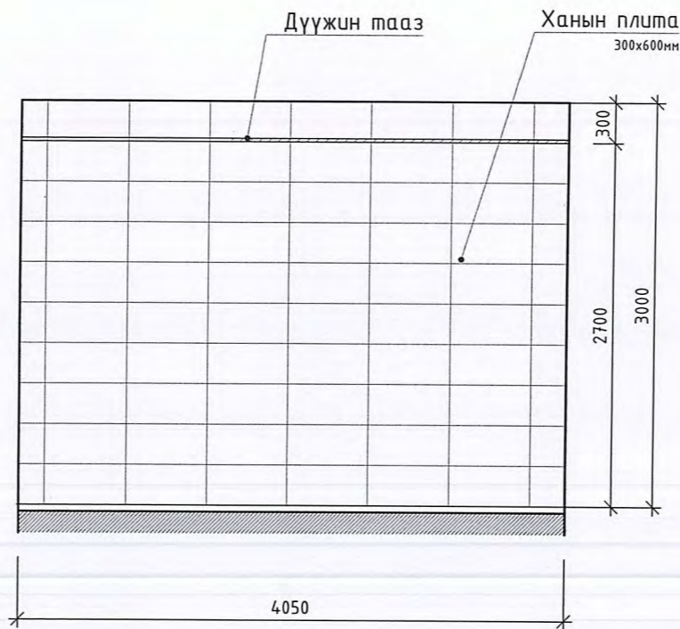
Ханын дэлгээс Х-2 М1 : 50
