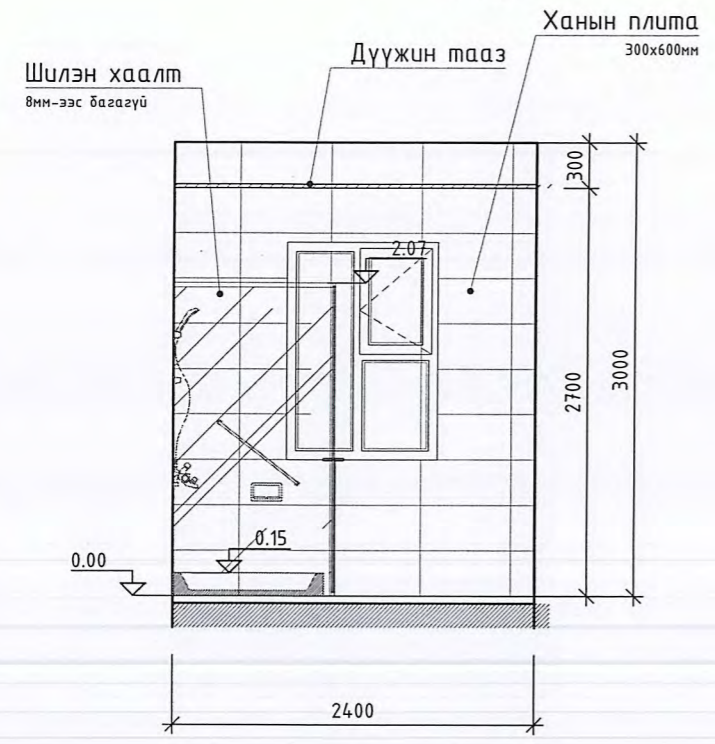
Ханын дэлгээс Х-1 M1 : 50
