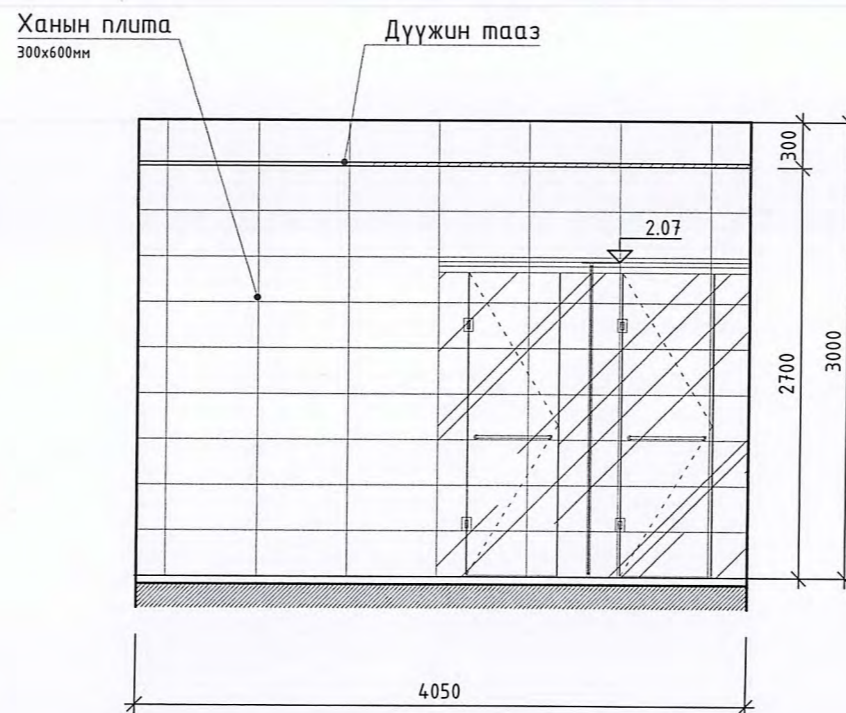
Ханын дэлгээс Х-4 М1 : 50
