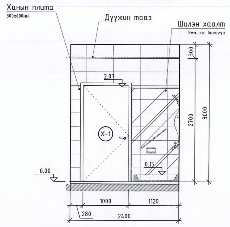
Ханын дэлгээс Х-3 M1 : 50
