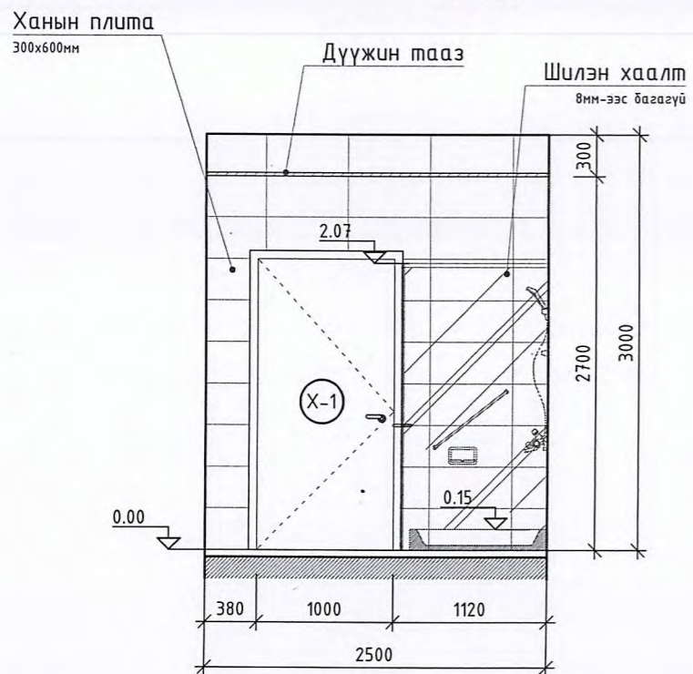
Ханын дэлгээс Х-3 М1 : 50
