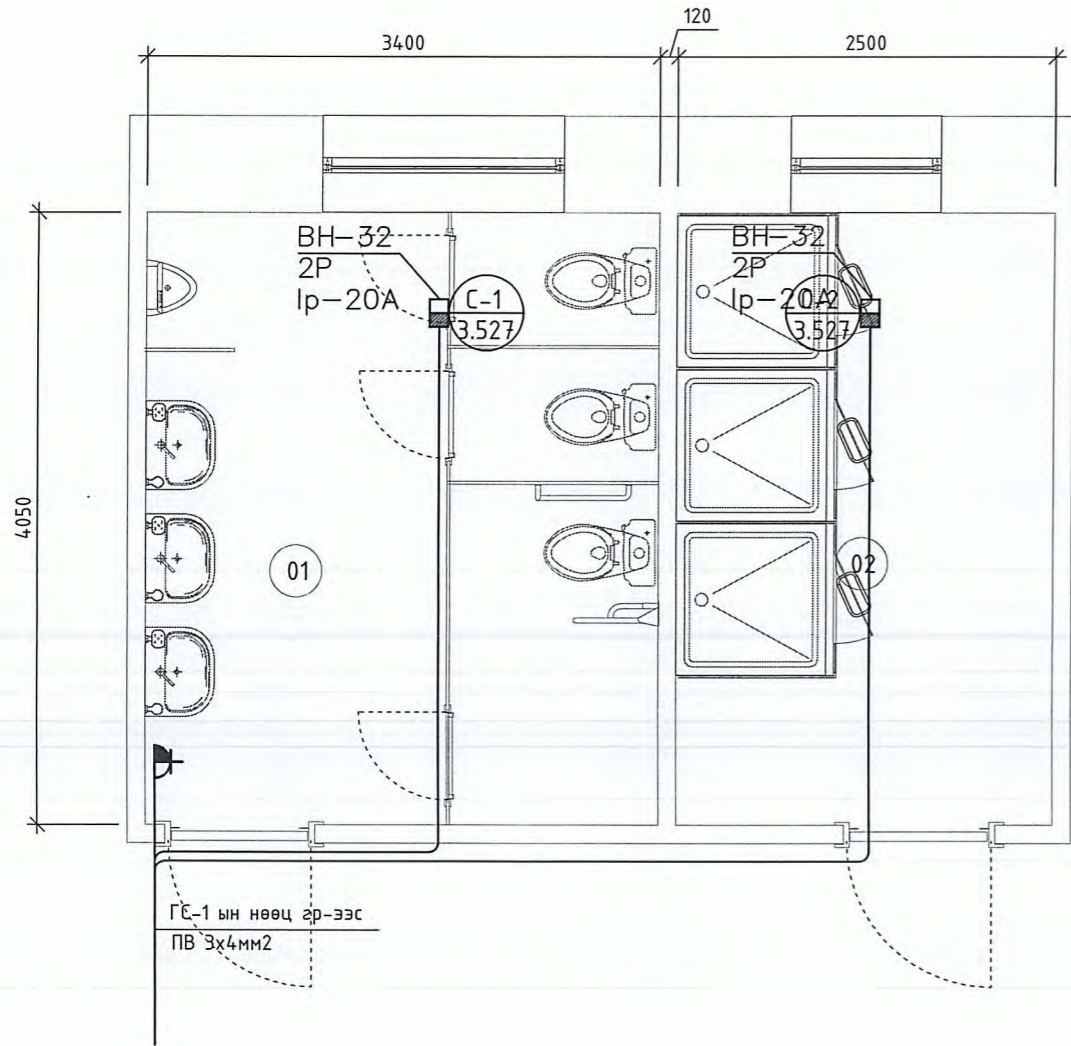
1-р давхрын өөрчлөлтийн хэсэгчилсэн байгуулалт-1
