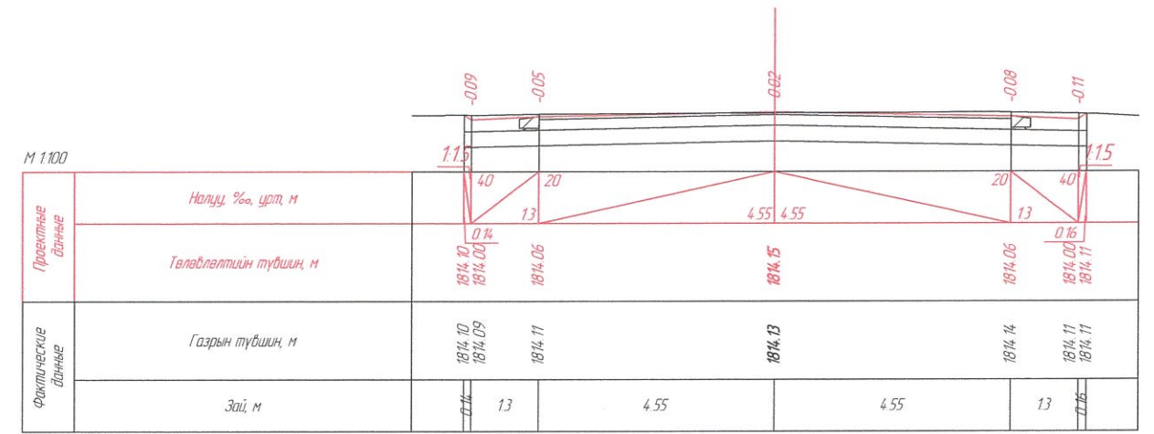
ПК 1-17.54
