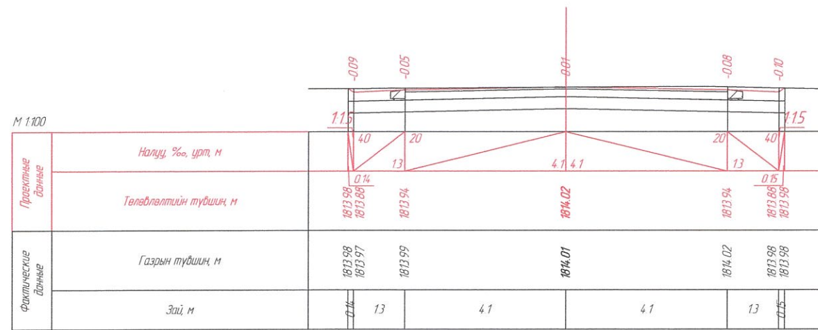
ПК 1-10.00
