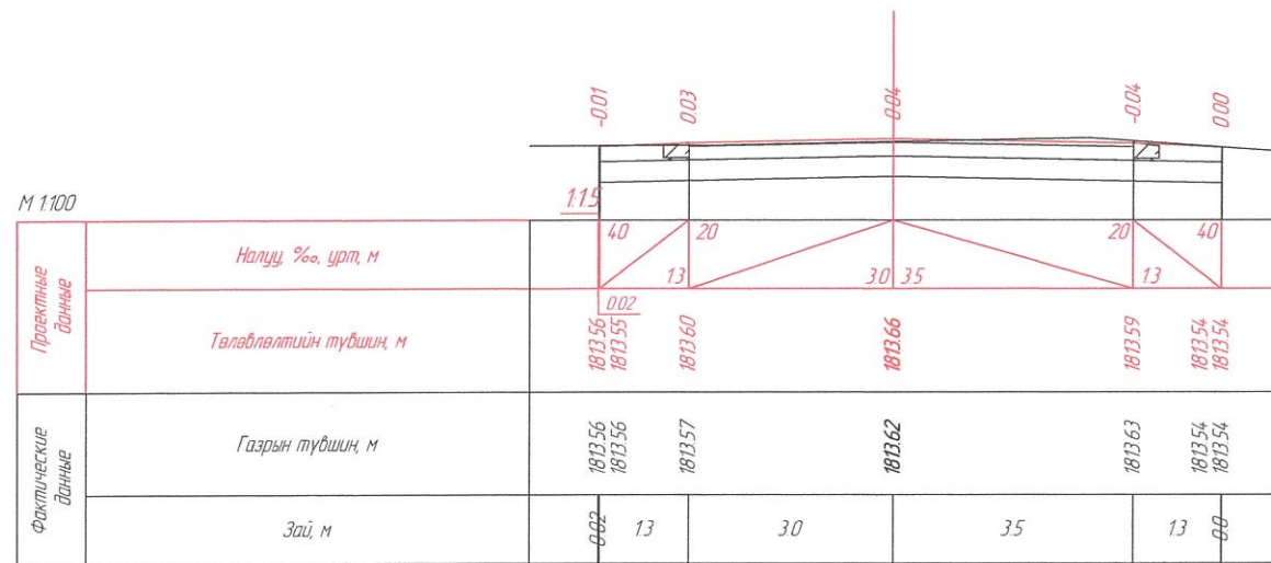
ПК 0+90.00
