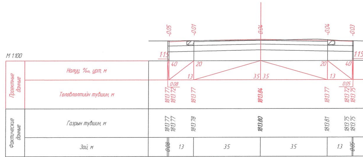
ПК 1+00.00
