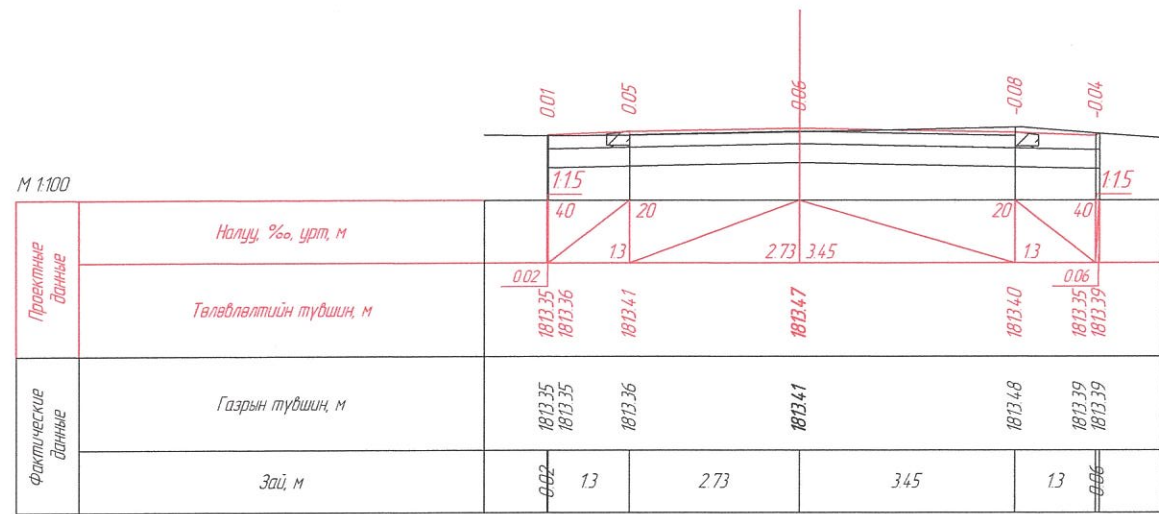
ПК 0+80.10
