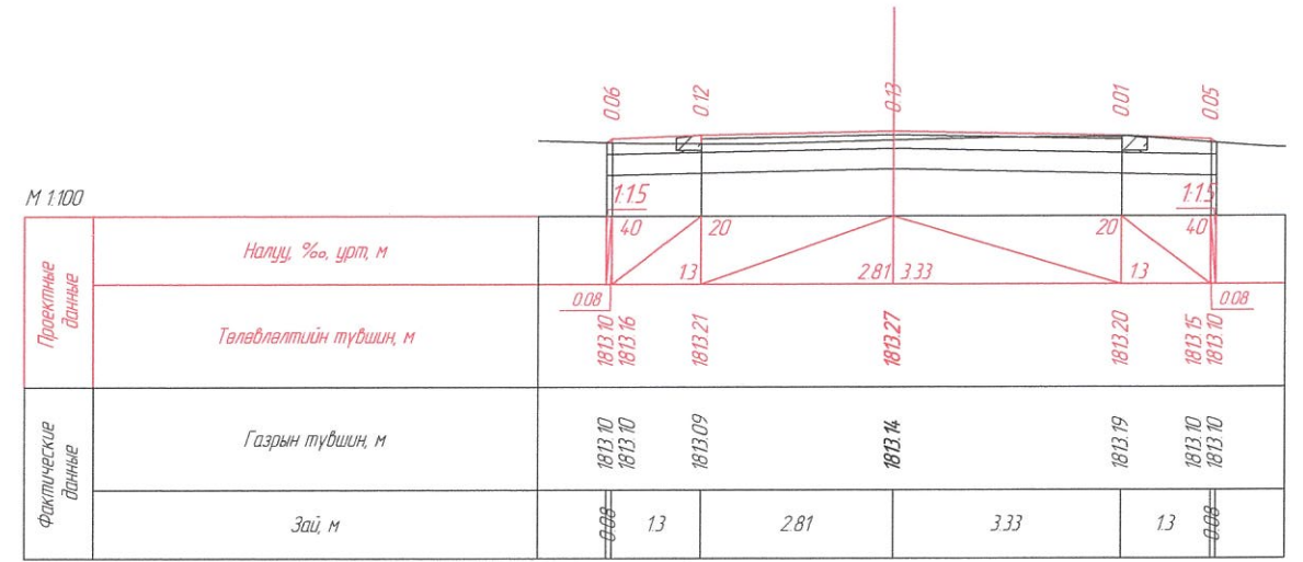
ПК 0+70.00
