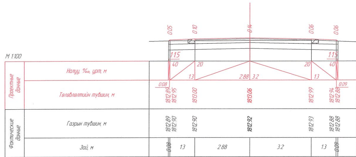
ПК 0+60.00
