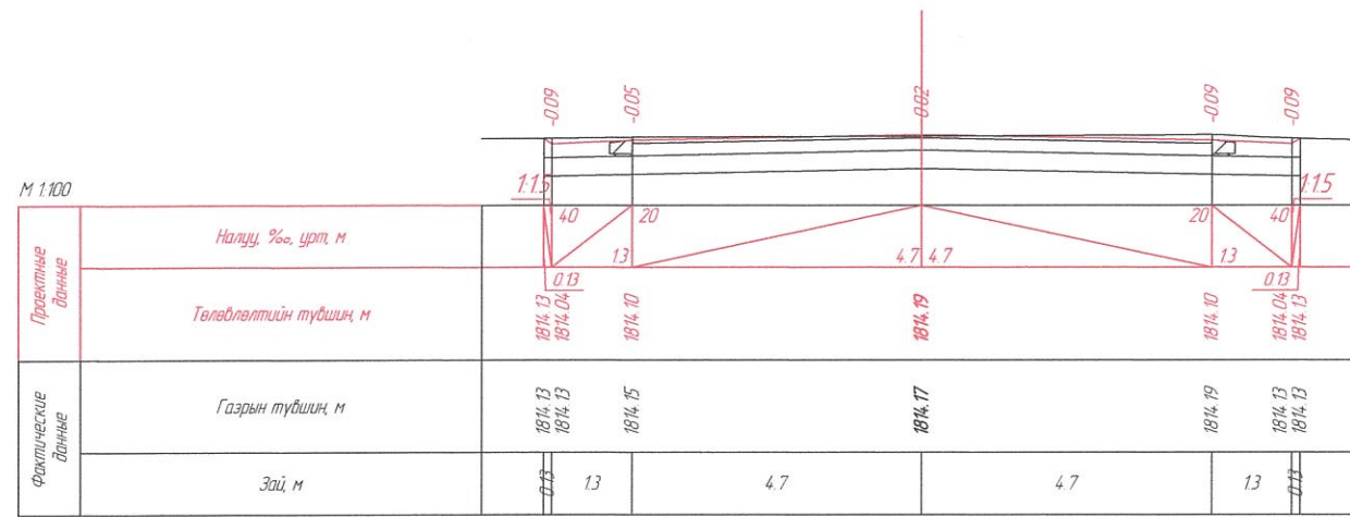
ПК 1-20.00
