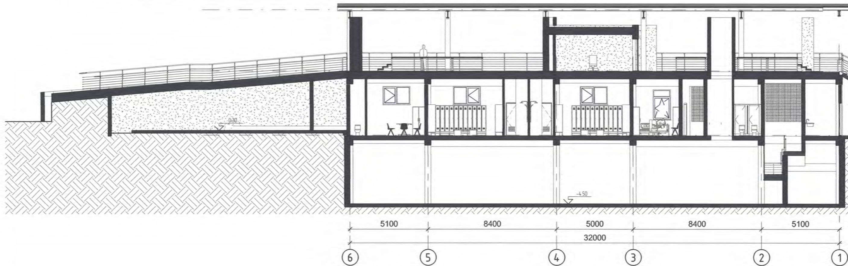
ОГТЛОЛ 3-3 1 : 150
