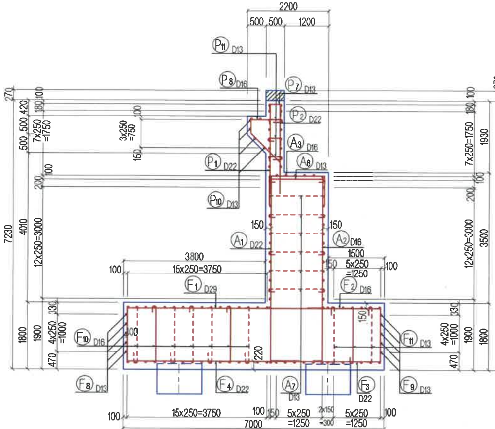
ХӨНДЛӨН ОГТЛОЛ 8-8
