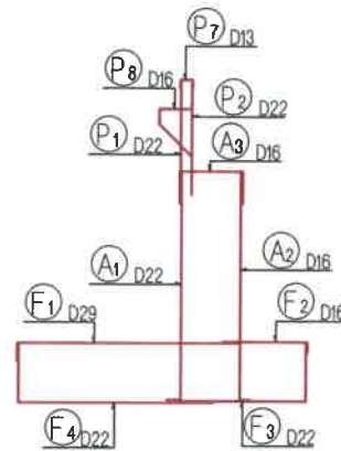
АРМАТУРЫН БАЙРЛАЛ
