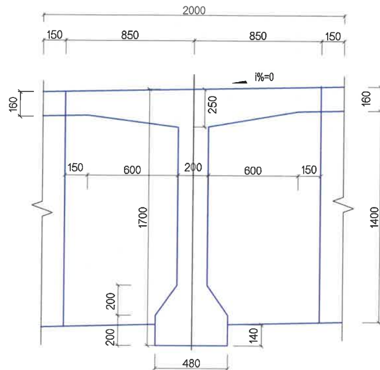
ЗАВСРЫН ДАМ НУРУУНЫ ХӨНДЛӨН ОГТЛОЛ (ДАМ НУРУУНЫ ГОЛД)
