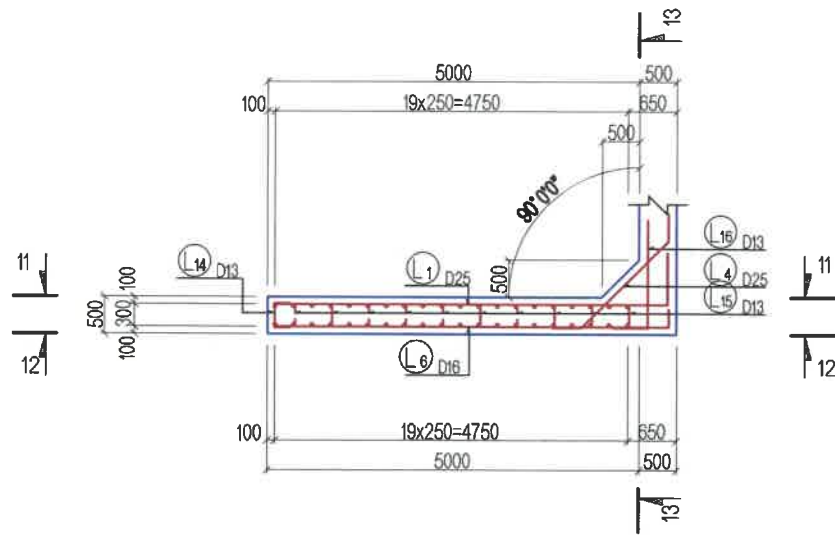
ДАЛАВЧНЫ АРМАТУРЫН БАЙГУУЛАЛТ
