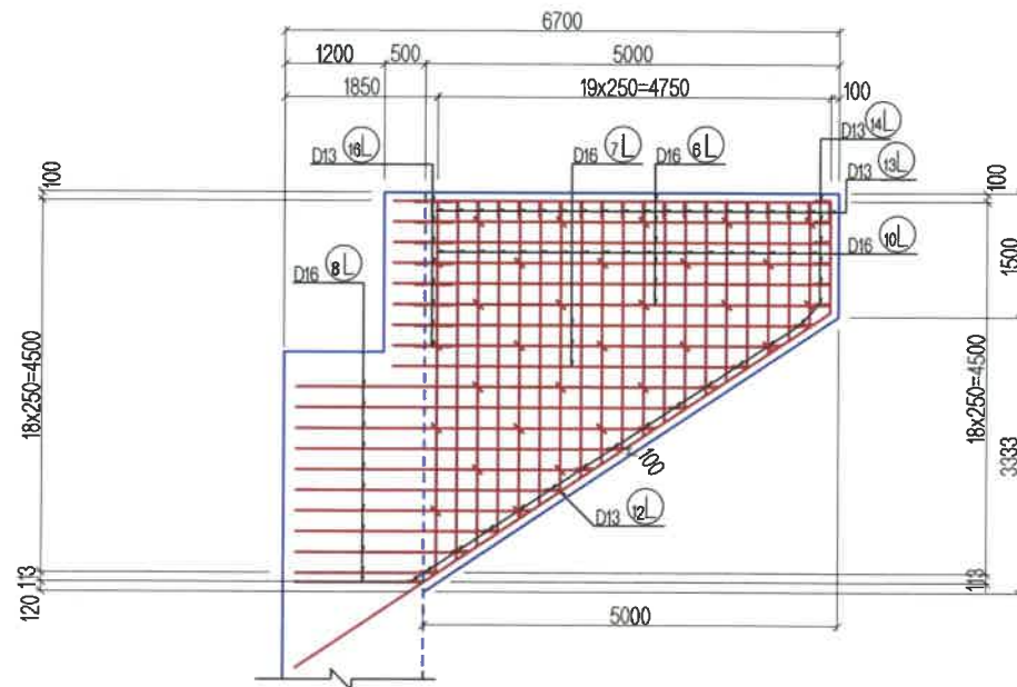
ГАДНА ТАЛ 11-11
