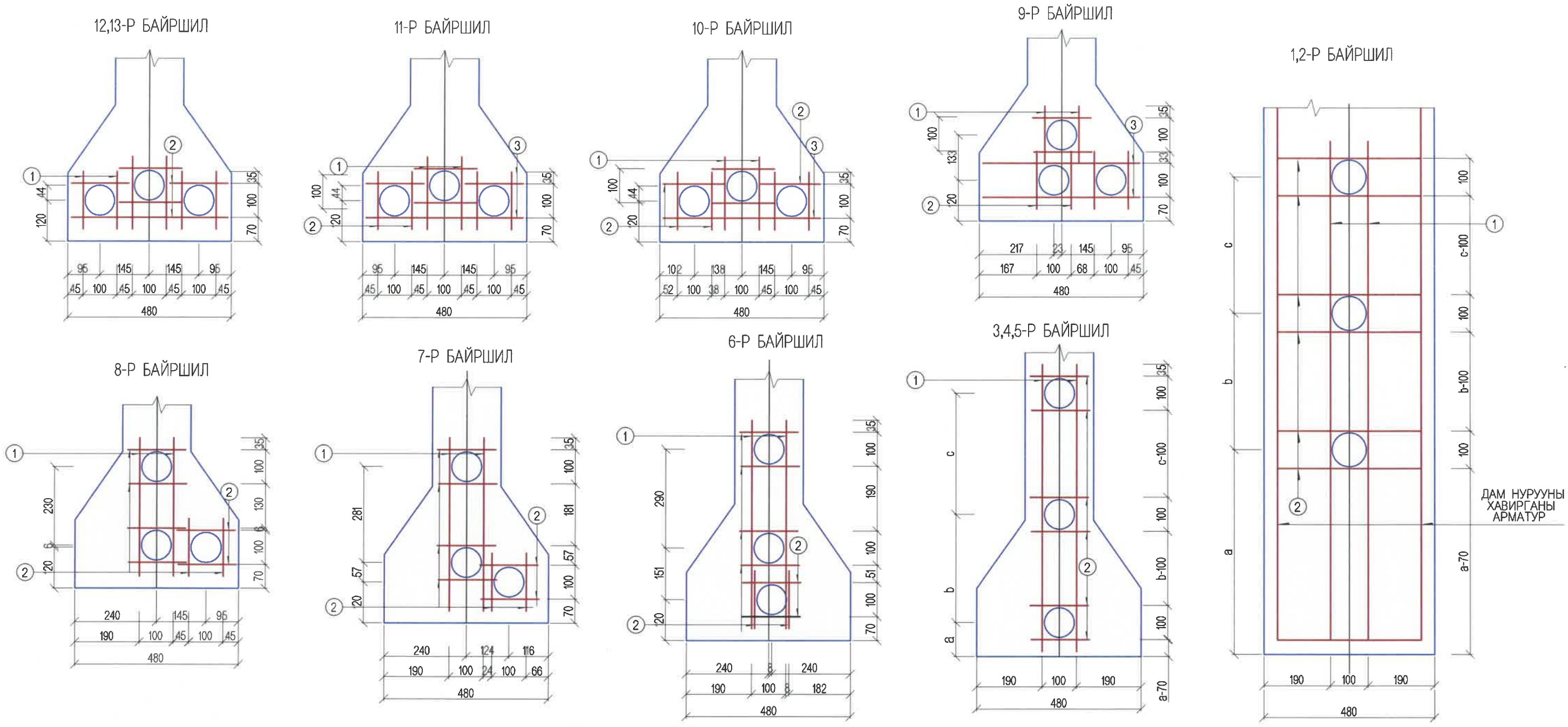
НЭГ ДАМ НУРУУНД ОРОХ АРМАТУРЫН ТОО ХЭМЖЭЭ
