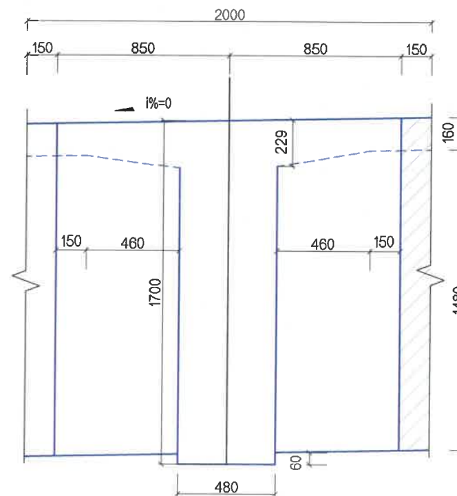
ЗАВСРЫН ДАМ НУРУУНЫ ХӨНДЛӨН ОГТЛОЛ (ЗААДАСНЫ ХАРАЛДАА)
