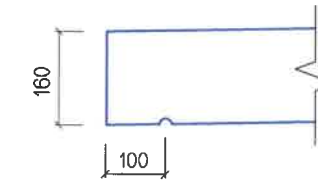
ДЕТАЛЬ А ЗАХЫН ДАМ НУРУУНЫ УСНЫ ХОВИЛ
