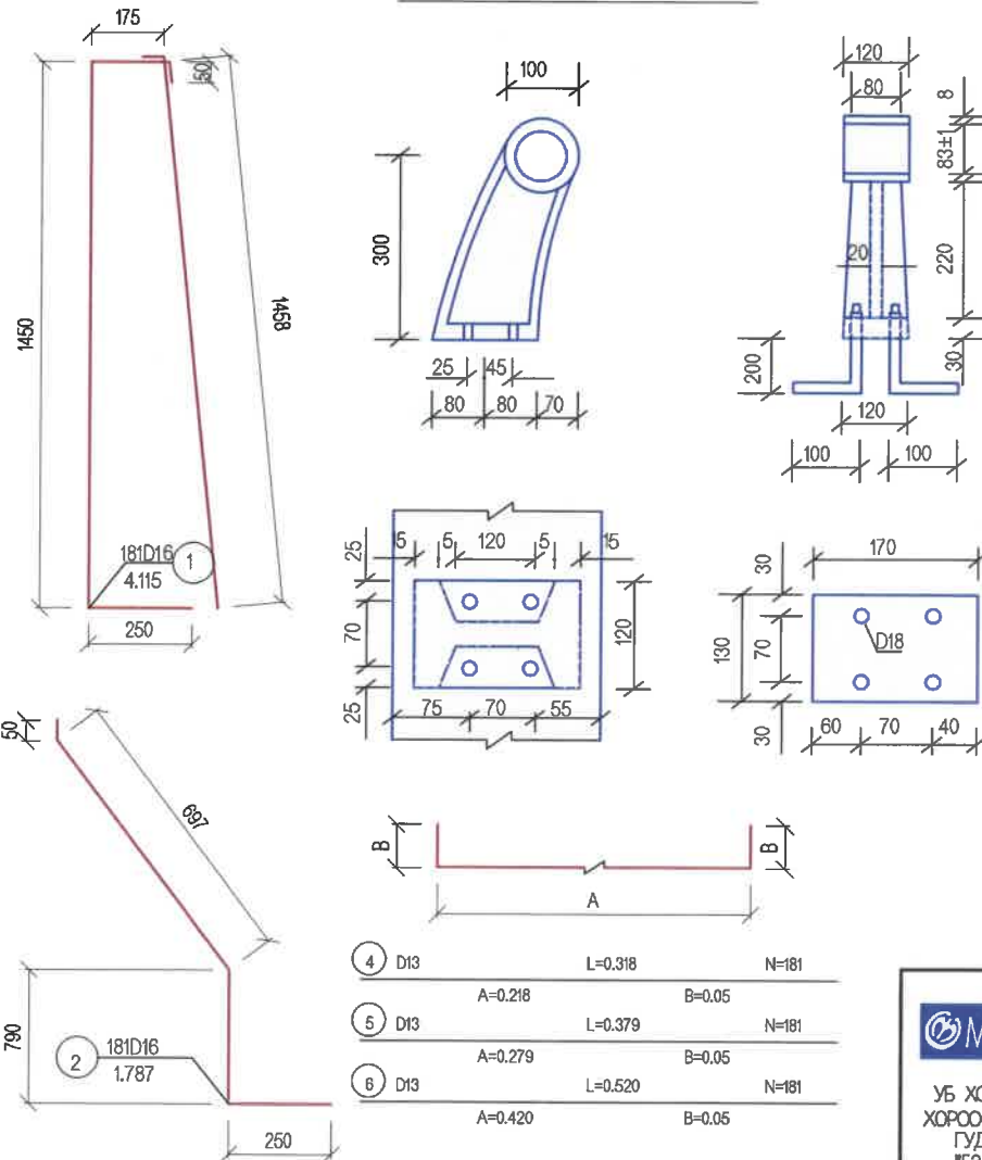
ХАМГААЛАЛТЫН ХАШЛАГА
