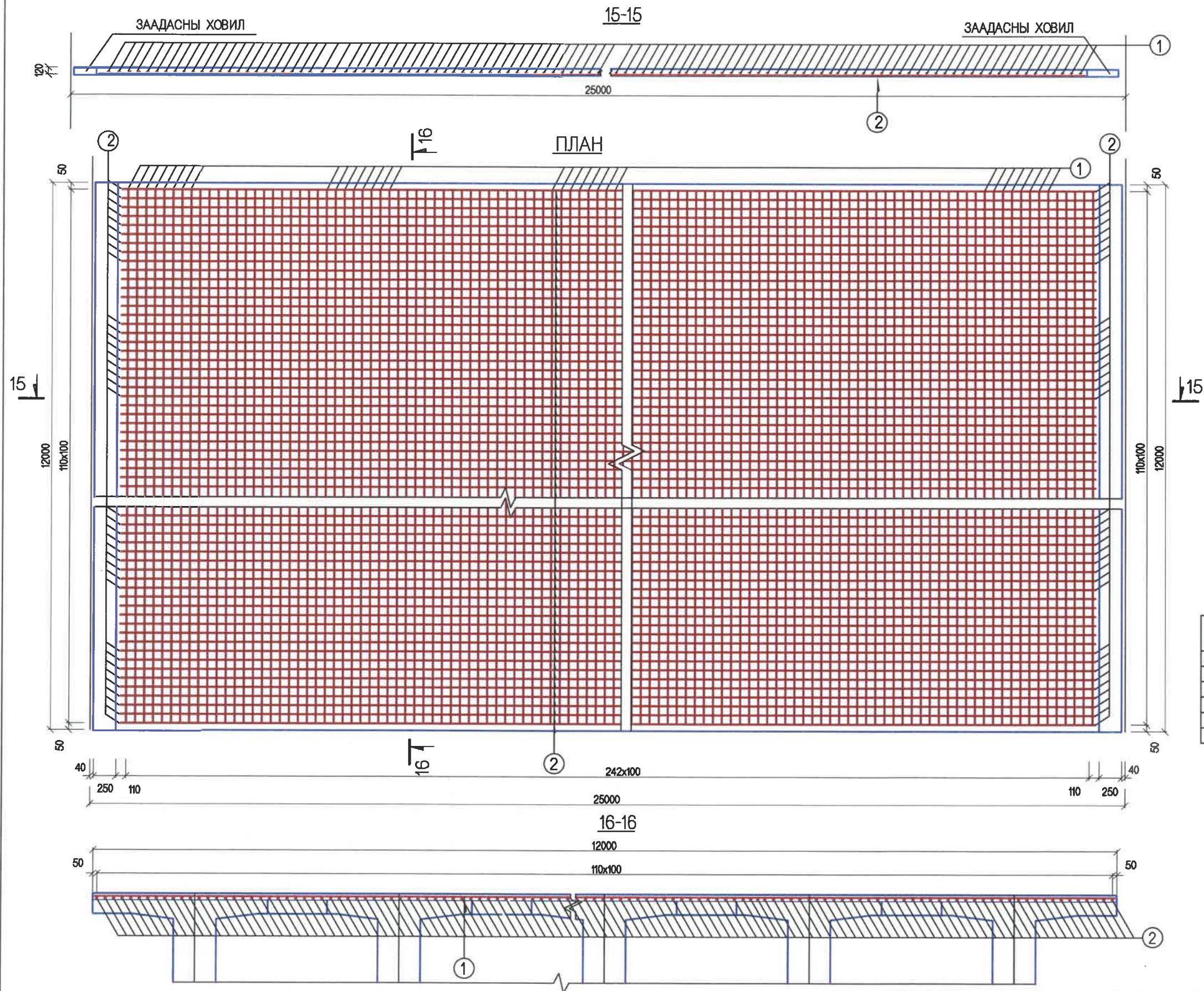
ДАМ НУРУУНЫ ДЭЭД ХАВТАНГИЙН АЖЛЫН ТОО ХЭМЖЭЭ
