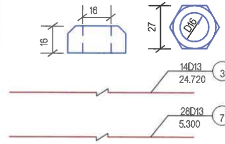
БООЛТ
