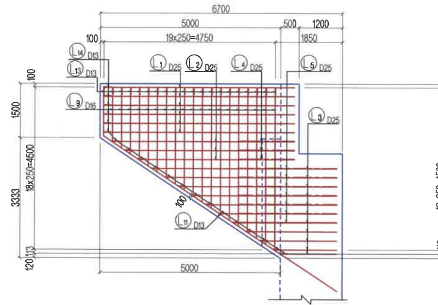
ДОТОР ТАЛ 12-12
