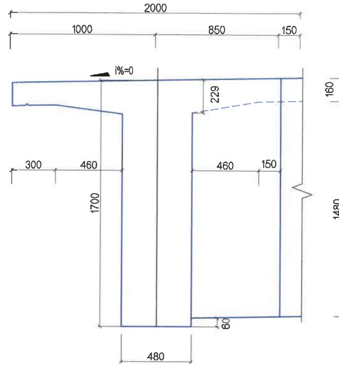
ЗАВСРЫН ДАМ НУРУУНЫ ХӨНДЛӨН ОГТЛОЛ (ЗААДАСНЫ ХАРАЛДАА)
