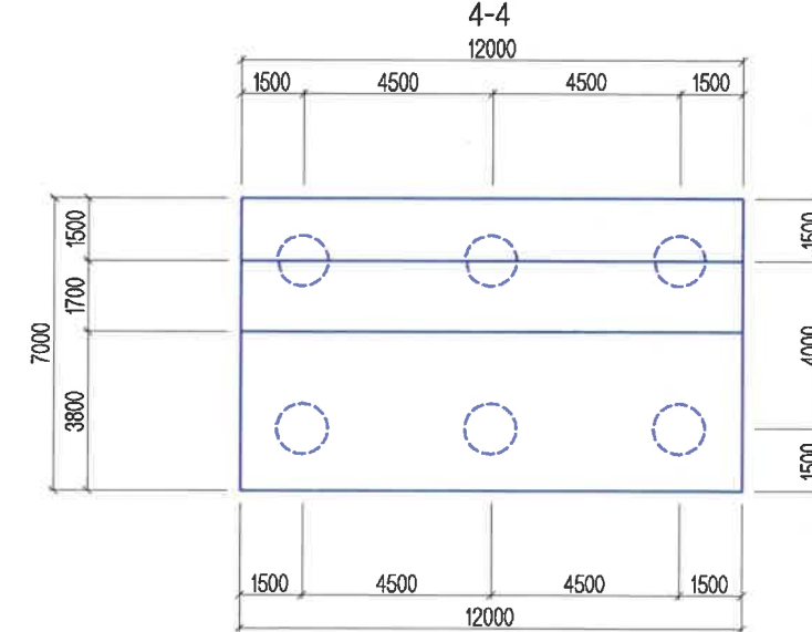
ЁРООЛЫН ПЛАН
