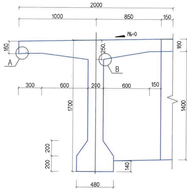
ЗАВСРЫН ДАМ НУРУУНЫ ХӨНДЛӨН ОГТЛОЛ (ДАМ НУРУУНЫ ГОЛД)
