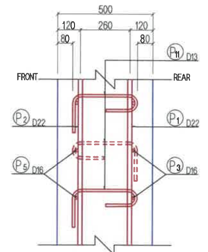
АР ХАНАНЫ ДЕТАЛЬ
