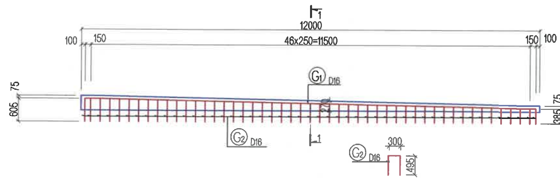
АРМАТУРЫН ХҮСНЭГТ
