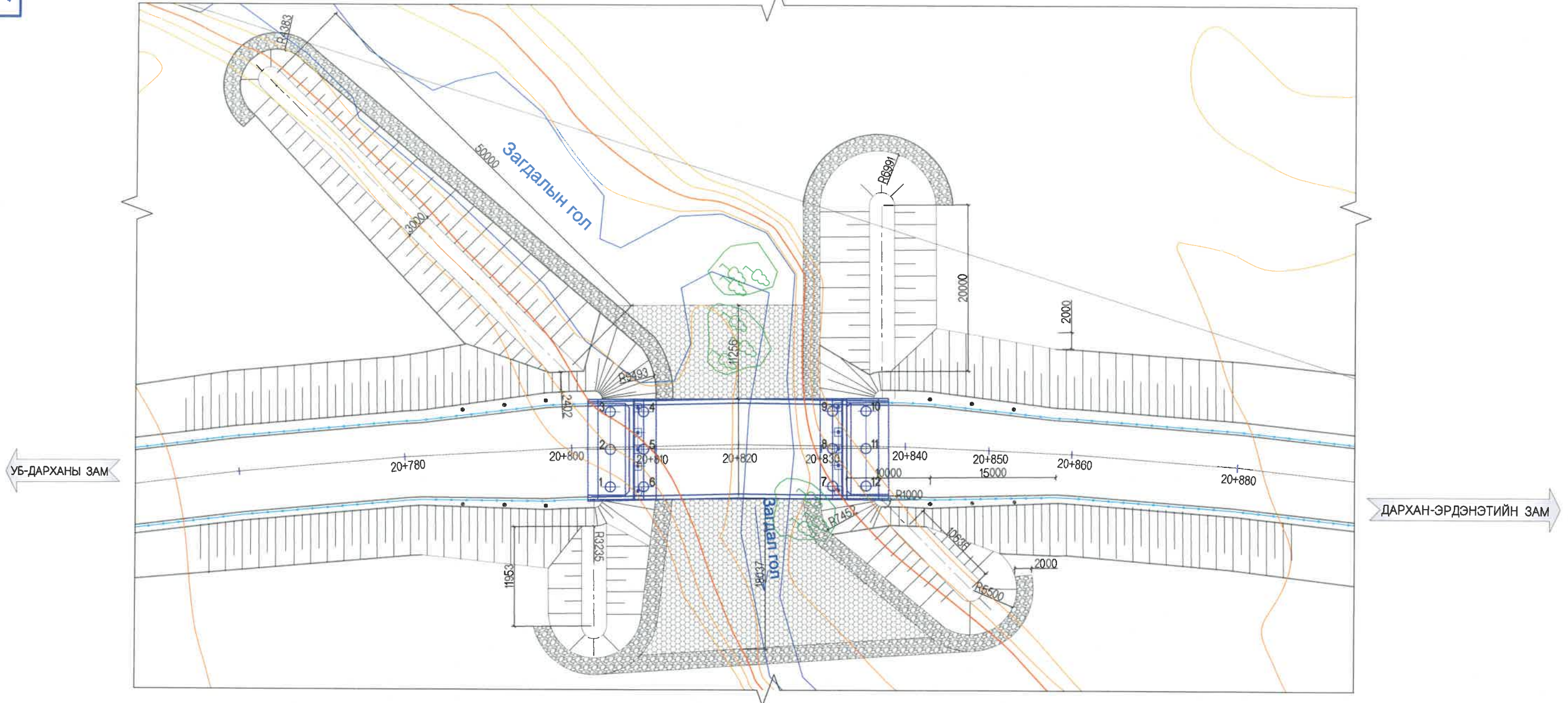
ГҮҮРИЙН ШОН ТУЛГУУРЫГ БАЙРЛУУЛАХ КООРДИНАТ
