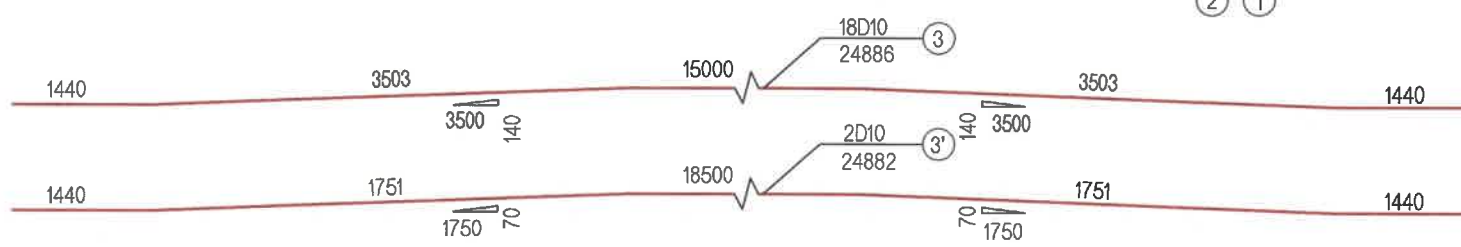
ДАМ НУРУУНЫ ХАВИРГАНЫ АРМАТУРЫН ТОО ХЭМЖЭЭ
