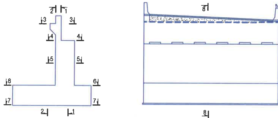
ОГТЛОЛЫН БАЙРЛАЛ
