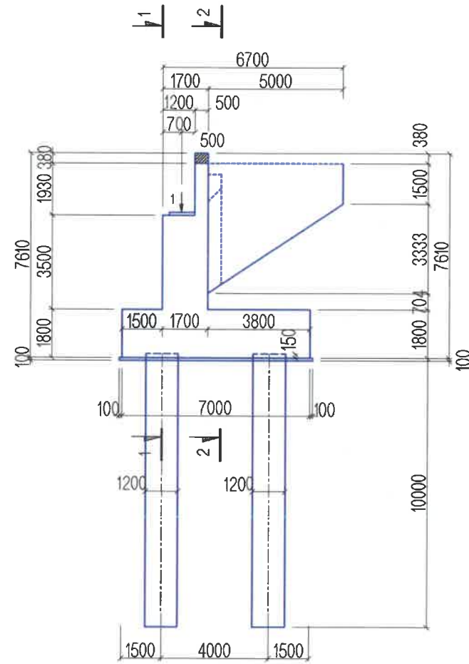
БАРУУН ТАЛ 6-6
