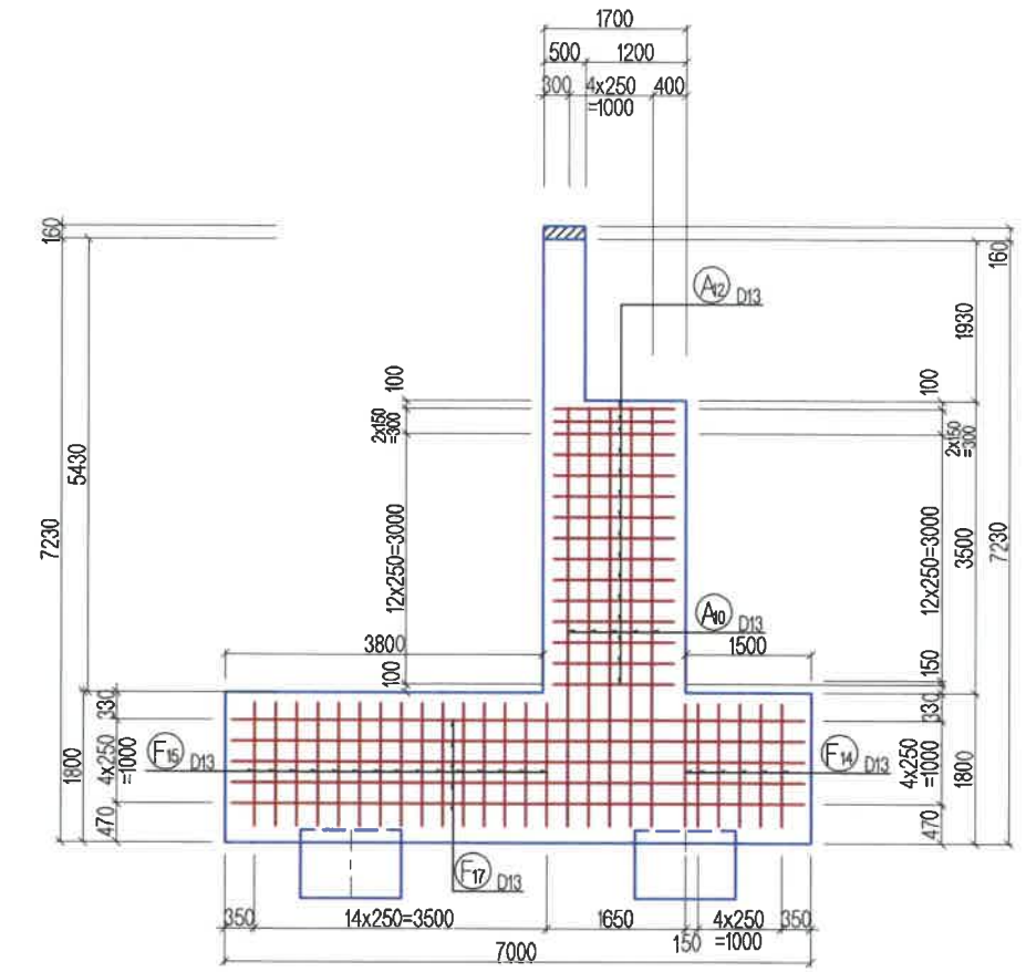
ЗҮҮН ТАЛ
