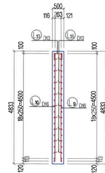
ХӨНДЛӨН ОГТЛОЛ 13-13
