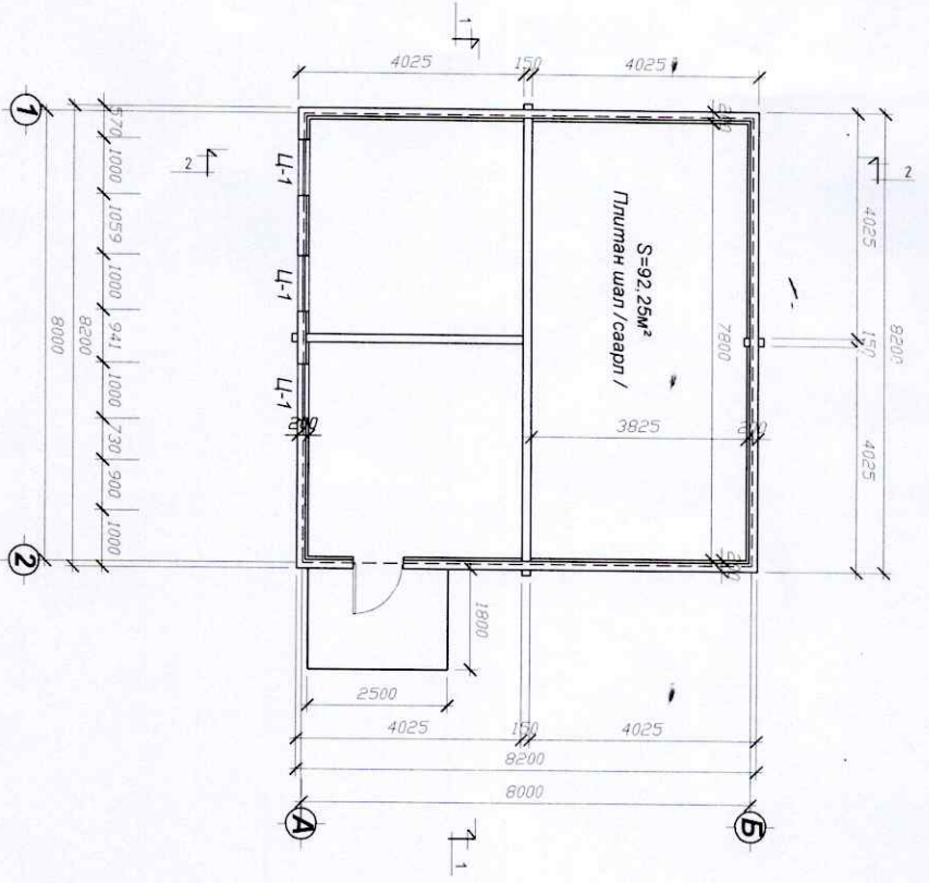
Хэсэглэл-А М1:25
