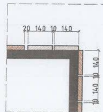
ХЭСЭГЛЭЛ 1 М1:12.5
