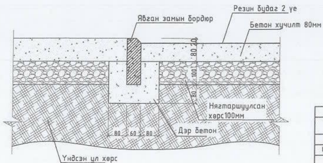
ОГТЛОЛ М1:10
