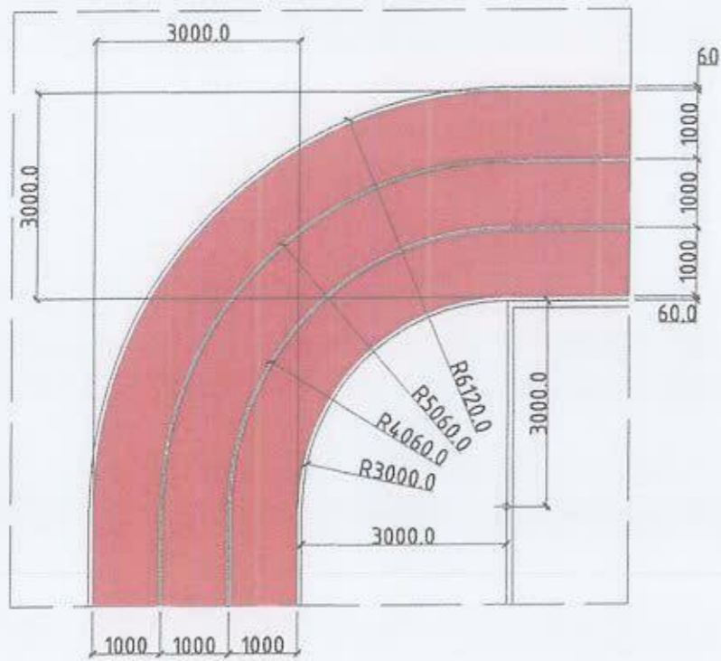
ХЭСЭГЛЭЛ М1:100
