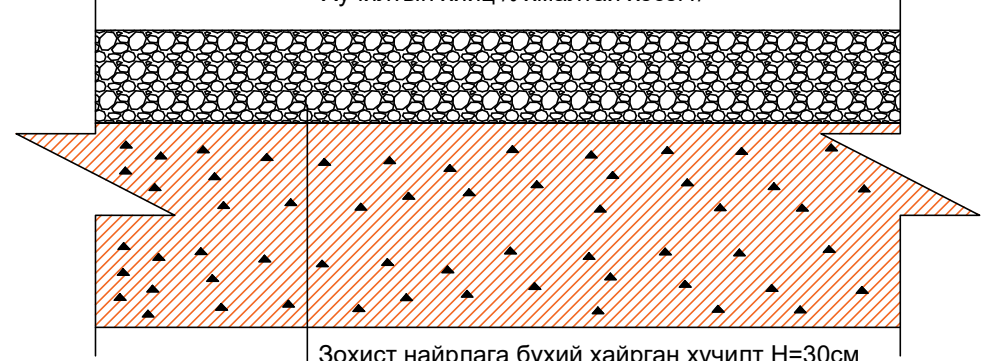
Хучилтын хийц /Ухмалтай хэсэгт/
