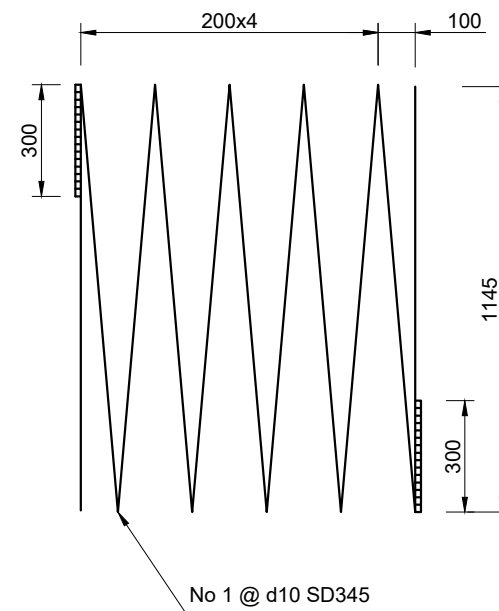
огтлол В - В SECTION B - B
