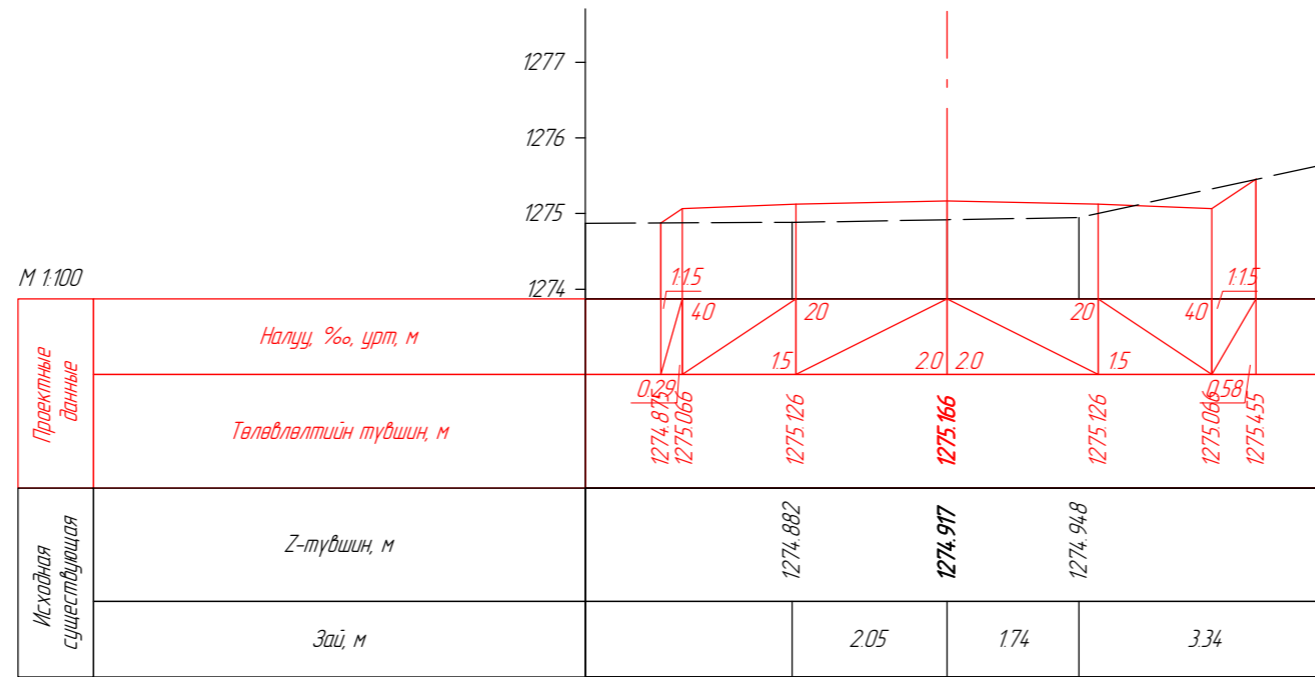
ПК 0+109.91
