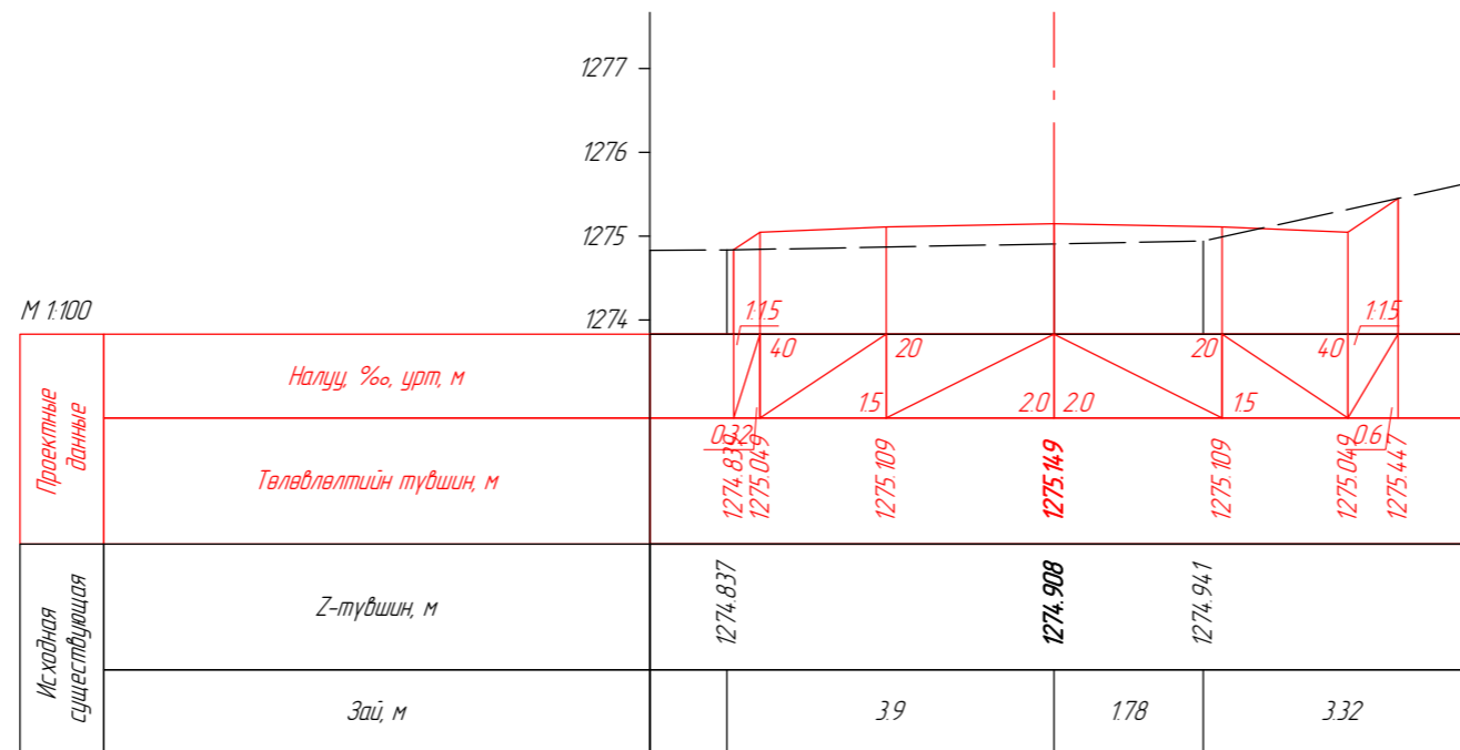
ПК 0+111.04
