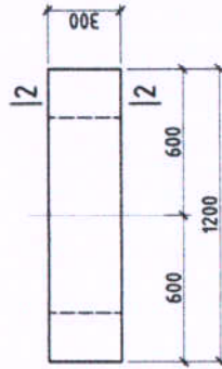
ТБТ-1 М1:25
