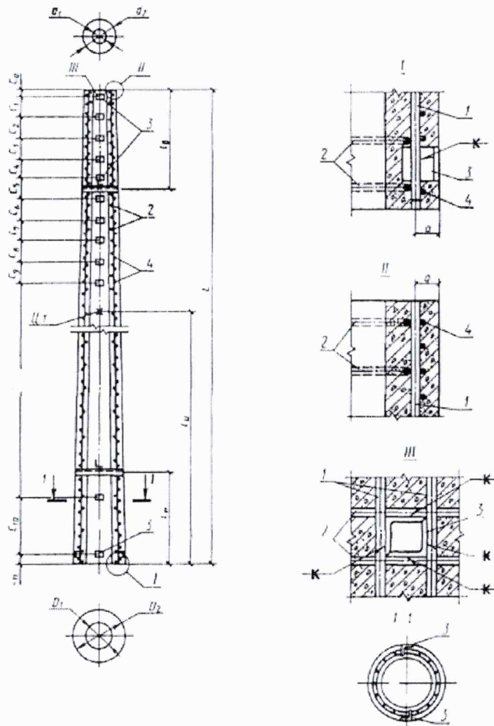
Төмөрбетон конусан шонгийн бэхэлгээний хийцийн хэмжээс, мм
