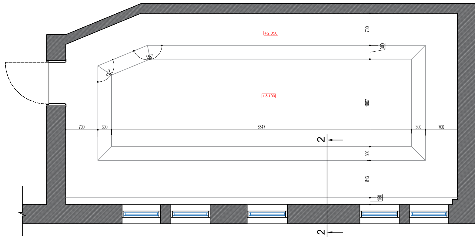
Таазны хэсэглэл
