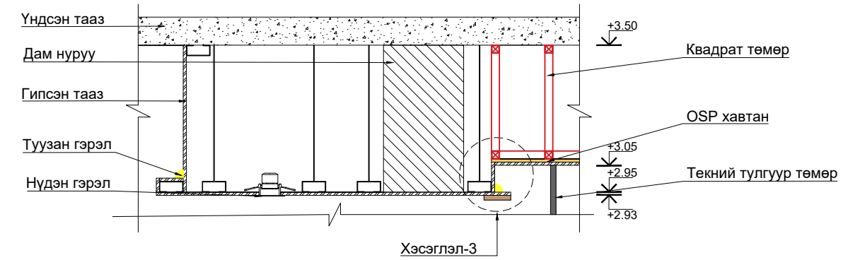
Хэсэглэл-3 /M1:20/
