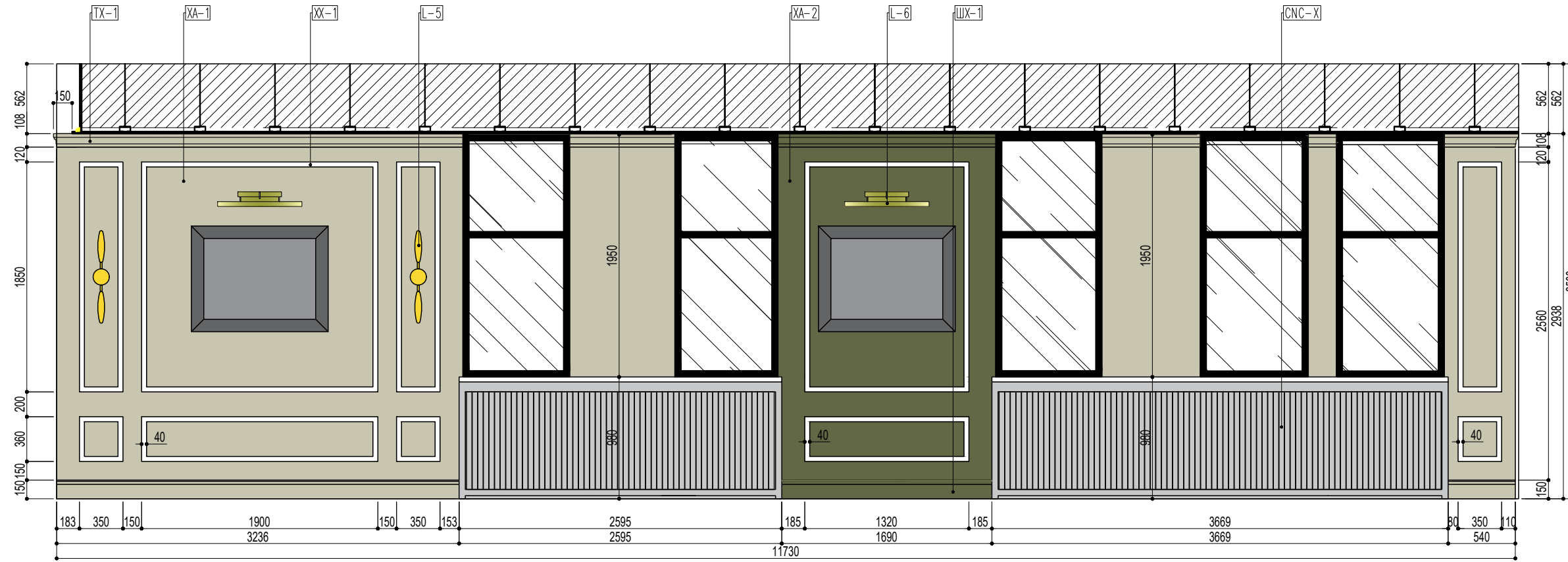
А ХАНАНЫ ДЭЛГЭЭС М1:40
