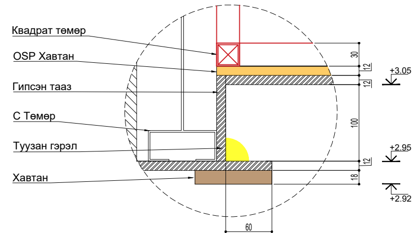
Хэсэглэл-3 /M1:20/
