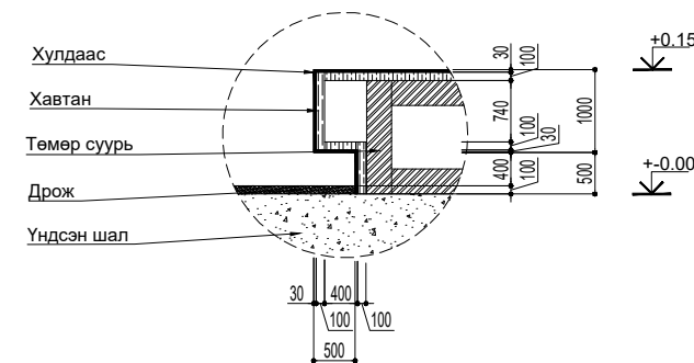
Хэсэглэл-1 /M1:10/
