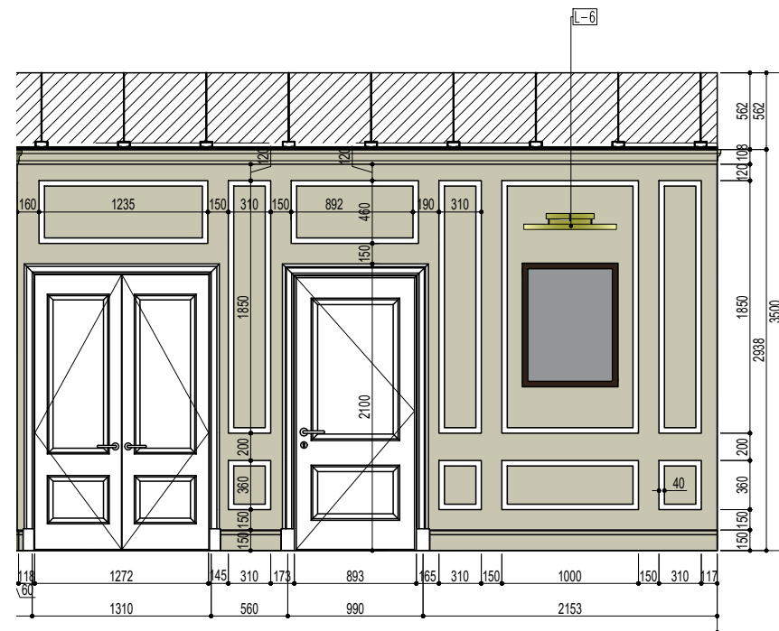
В ХАНАНЫ ДЭЛГЭЭС М1:50
