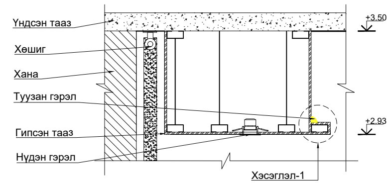
Хэсэглэл-1 /M1:20/
