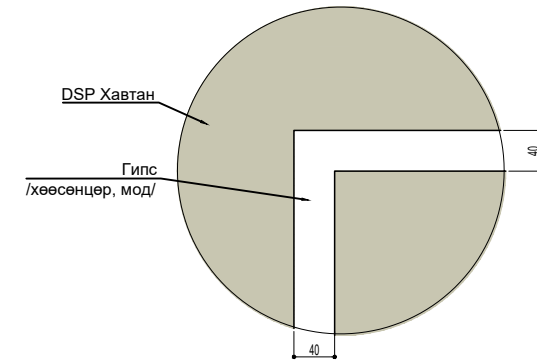
ХЭСЭГЛЭЛ 1-2 М1:10
