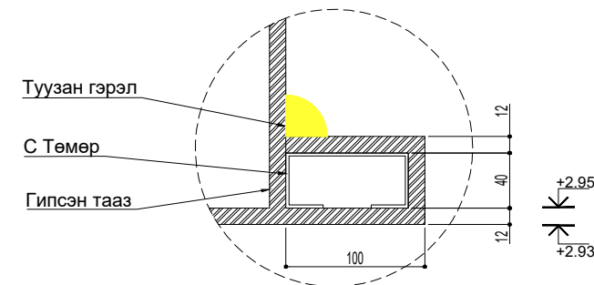
Хэсэглэл-1 /M1:20/
