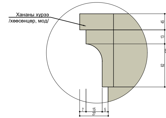
ХЭСЭГЛЭЛ 1-2 М1:10
