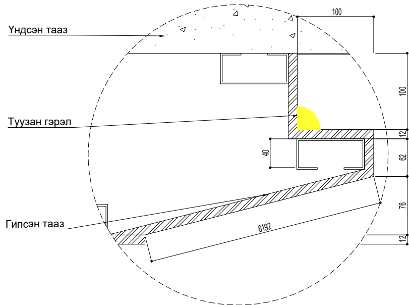
Хэсэглэл-2 /M1:20/
