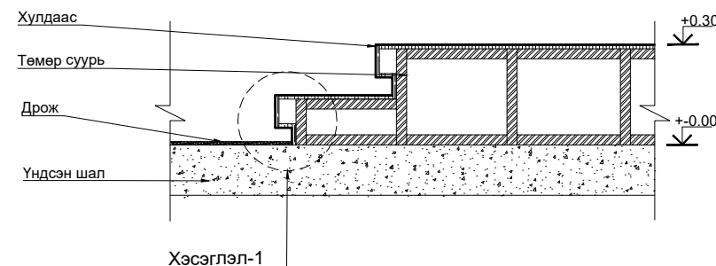
1-1 Огтлол /M1:20/
