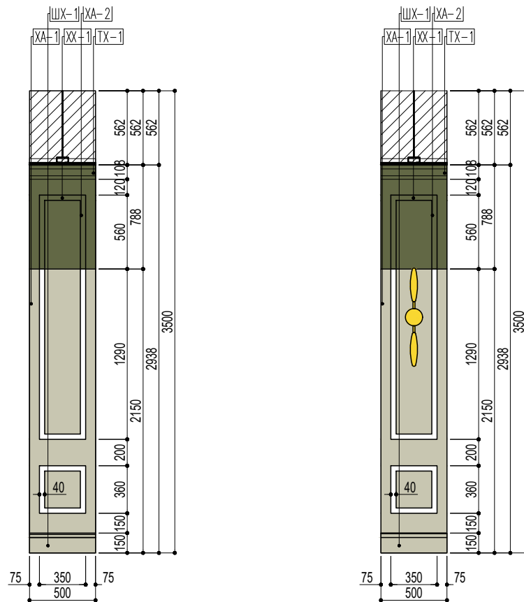
БАГАНЫ ДЭЛГЭЭС М1:40
