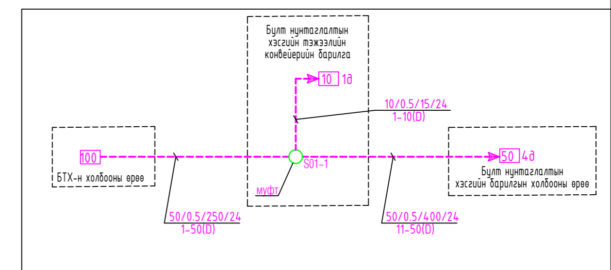
Физик кабелийн тархалтын бүдүүвч
