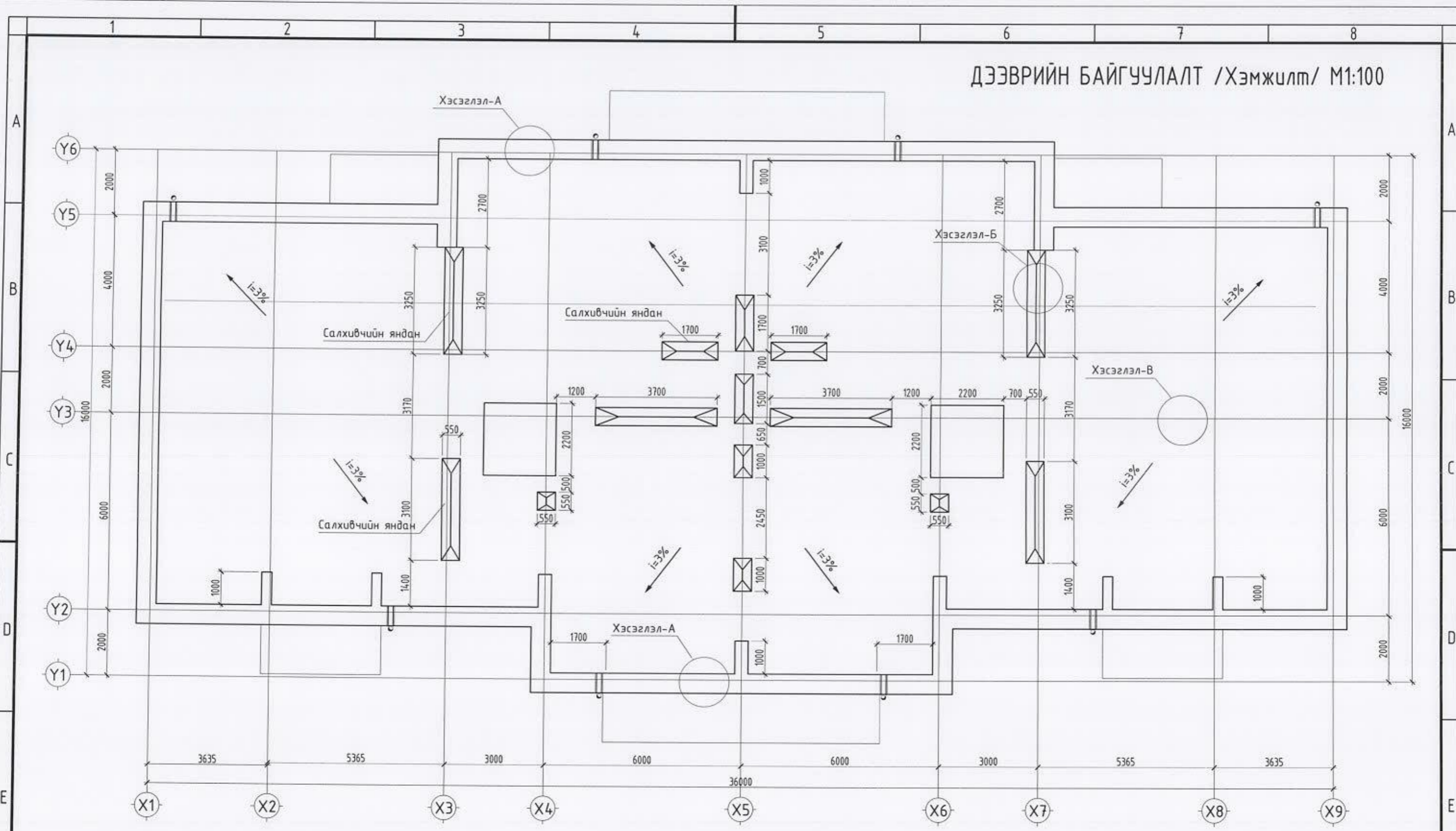
Салхивчийн яндан
