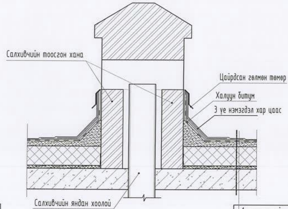
ХЭСЭГЛЭЛ-Б М1:25
