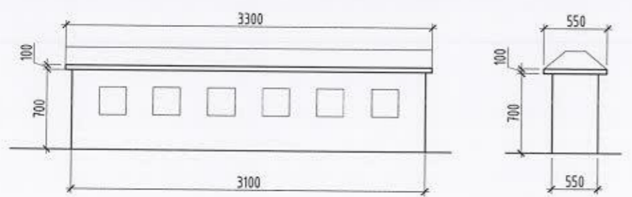
Салхивчийн яндан
