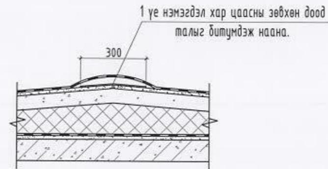
ХЭСЭГЛЭЛ-В М1:25
