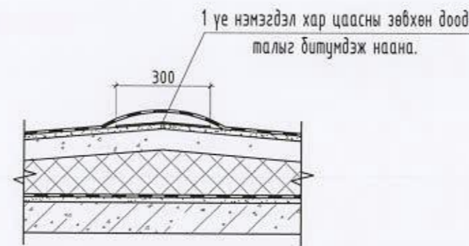
ХЭСЭГЛЭЛ-В М1:25
