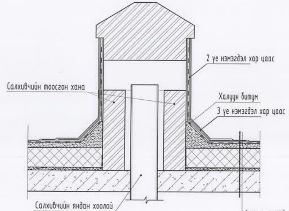
ХЭСЭГЛЭЛ-Б М1:25
