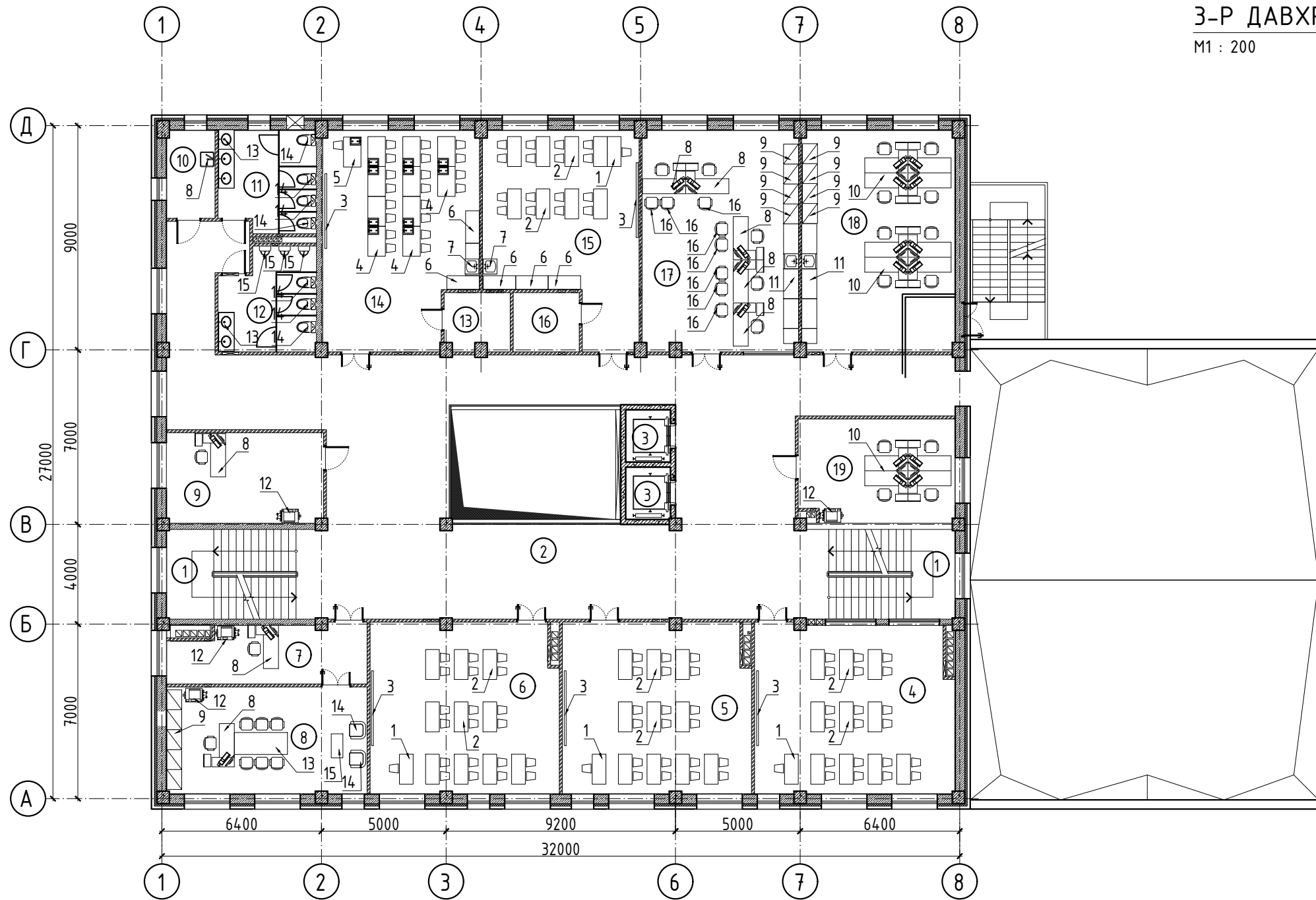
ТАВИЛГА, ТОНОГ ТӨХӨӨРӨМЖИЙН ТОДОРХОЙЛОЛТ
