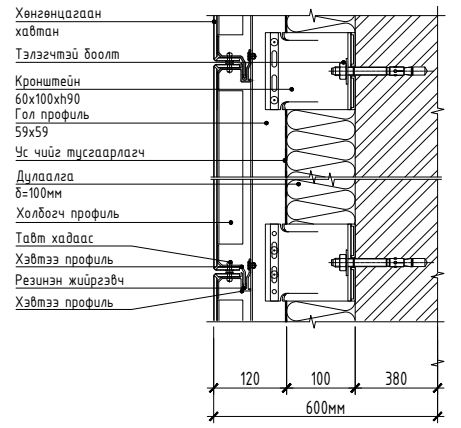
ГАДНА ХАНЫН ХЭСЭГЛЭЛ M1:10
