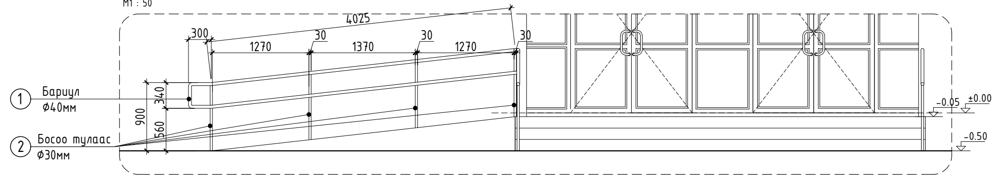
ОГТЛОЛ А-А M1 : 50
