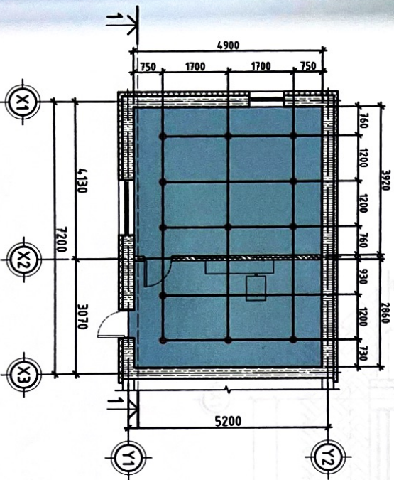
Тээвэрний байгуулалт М1:100
