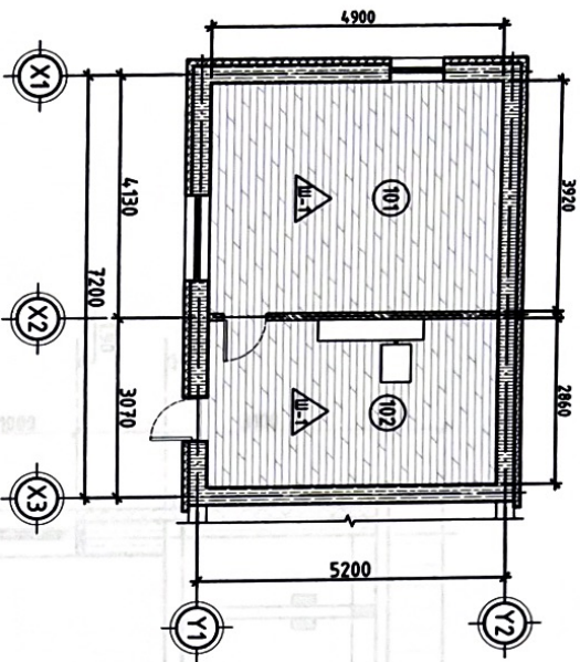
Шалны байгуулалт М1:100
