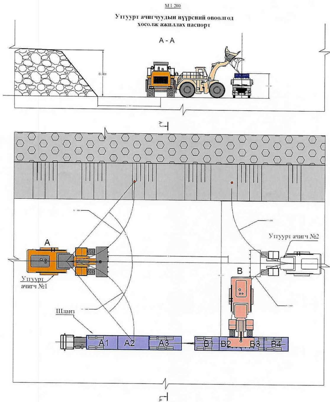
Зураг.2 Утгуурт ачигчуудын нүүрсний овоолгод хосолж ажиллах паспорт
