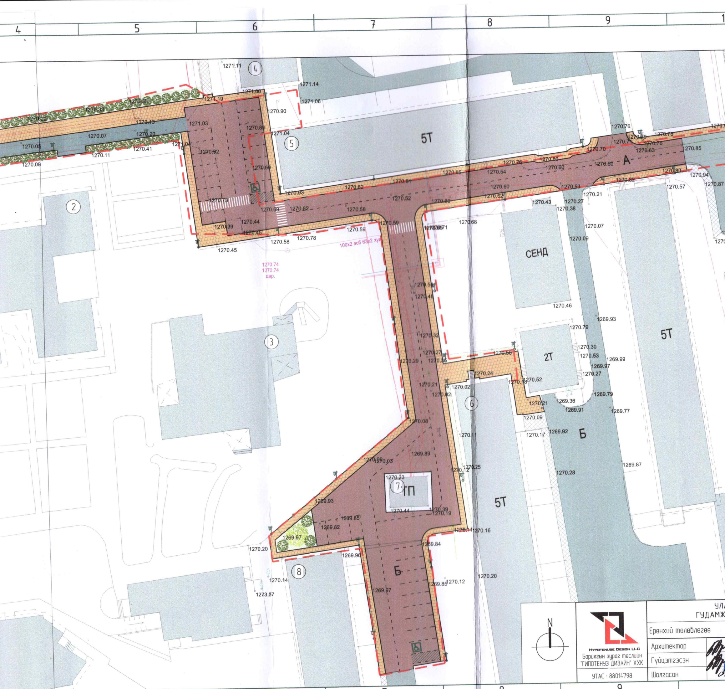
БАЙРШЛЫН СХЕМ М1:2000
