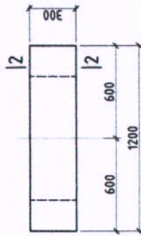
ТБТ-1 М1:25
