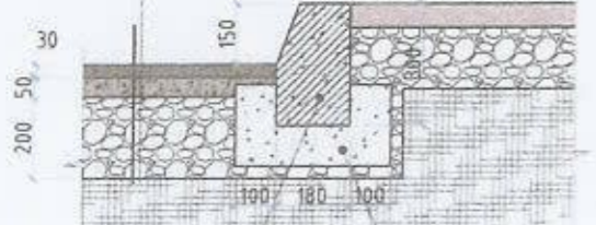
Явган замын бордюр Дэр бетон
