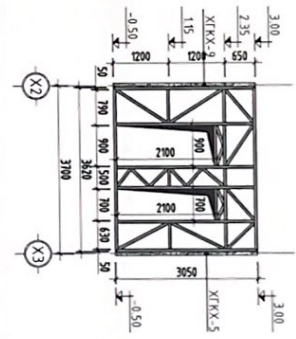
ХӨНГӨН ГАН КАРКАСАН ХАНА "ХТКХ-10" М1:100
