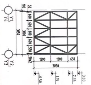
ХӨНГӨН ГАН КАРКАСАН ХАНА "ХТКХ-9" М1:100
