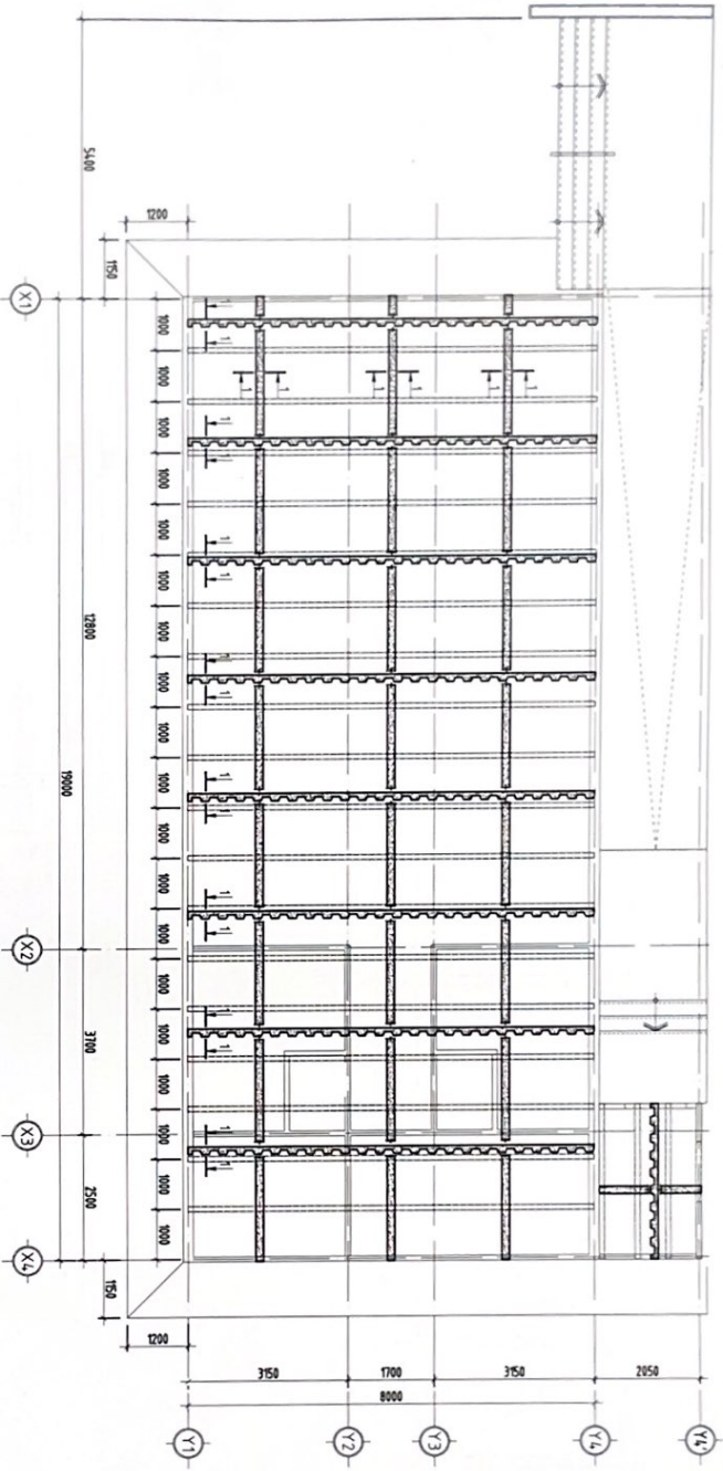
Зуг заг даацын ган хүчдэсний байгуулалтын схем М1:200
