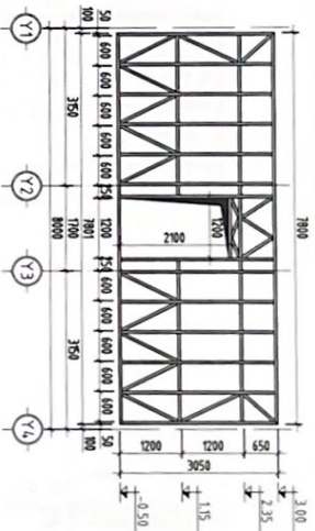
ХӨНГӨН ГАН КАРКАСАН ХАНА "ХТКХ-5" М1:100
