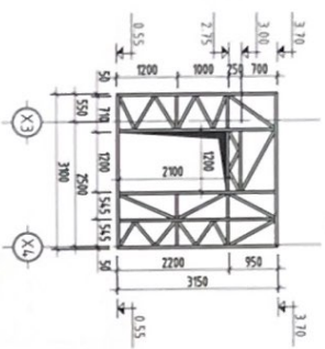
ХӨНГӨН ГАН КАРКАСАН ХАНА "ХТКХ-8" М1:100
