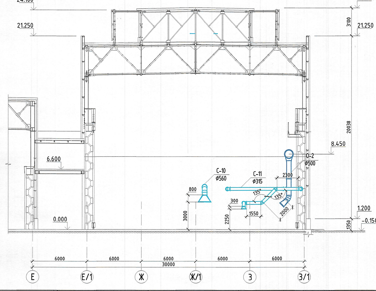
ОГТЛОЛ 3-3 М1:200
