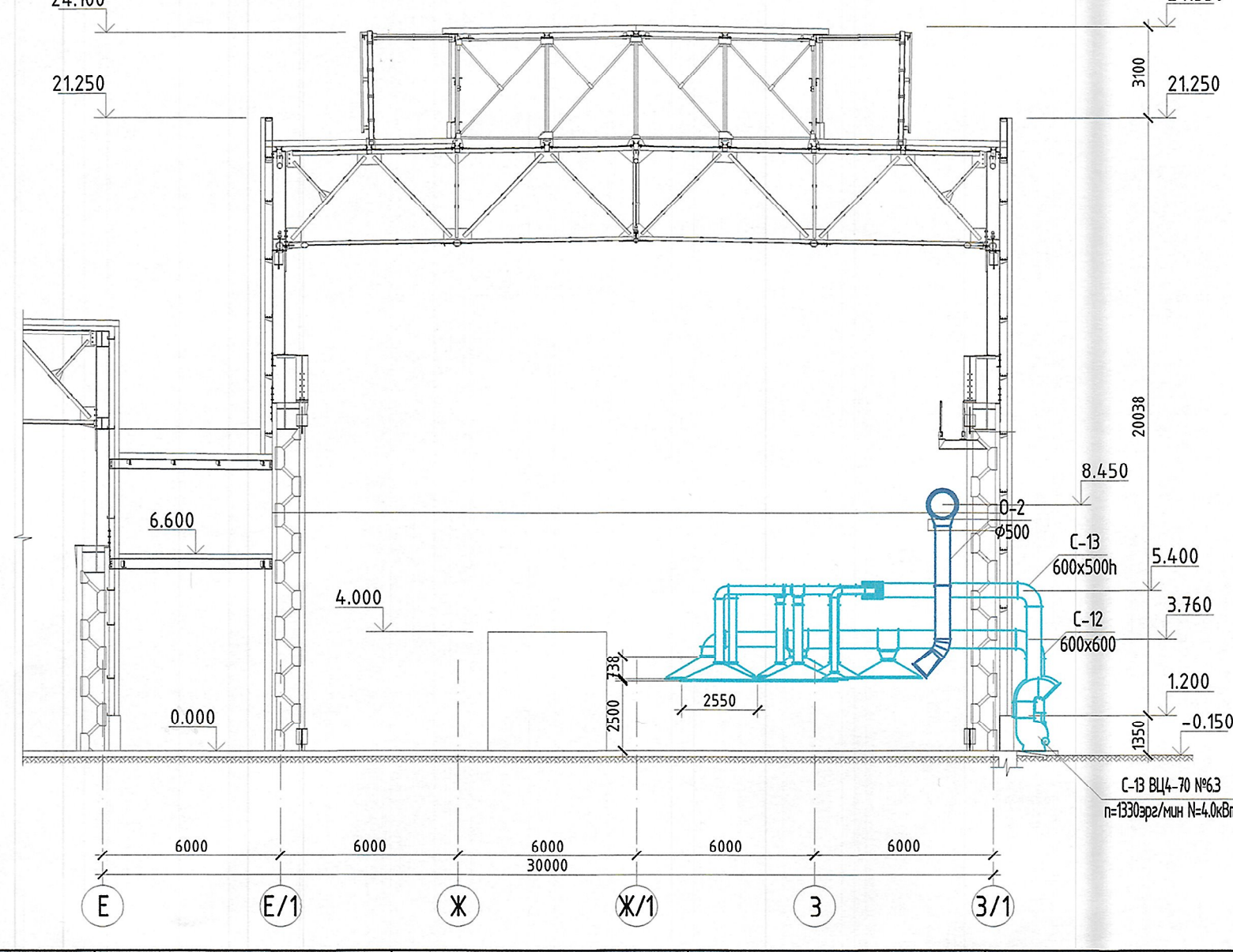
ОГТЛОЛ 4-4 М1:200
