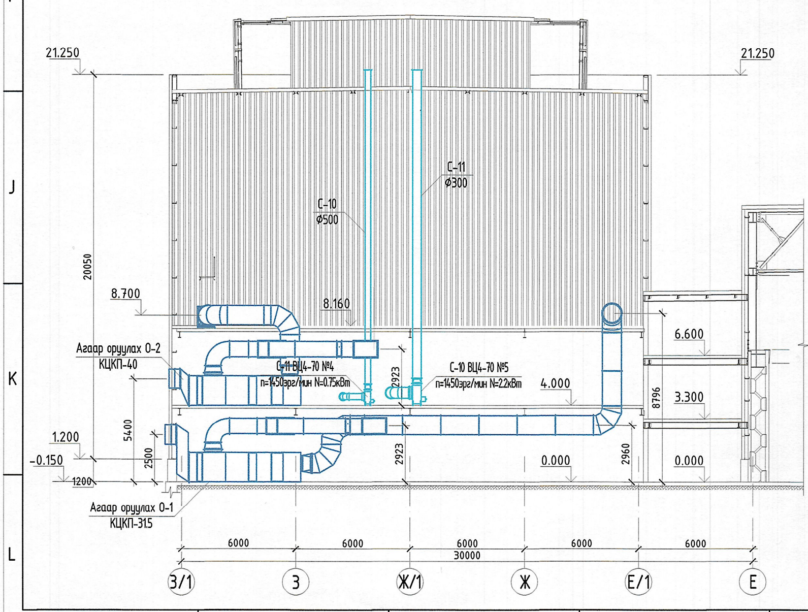
ОГТЛОЛ 2-2 М1:200
