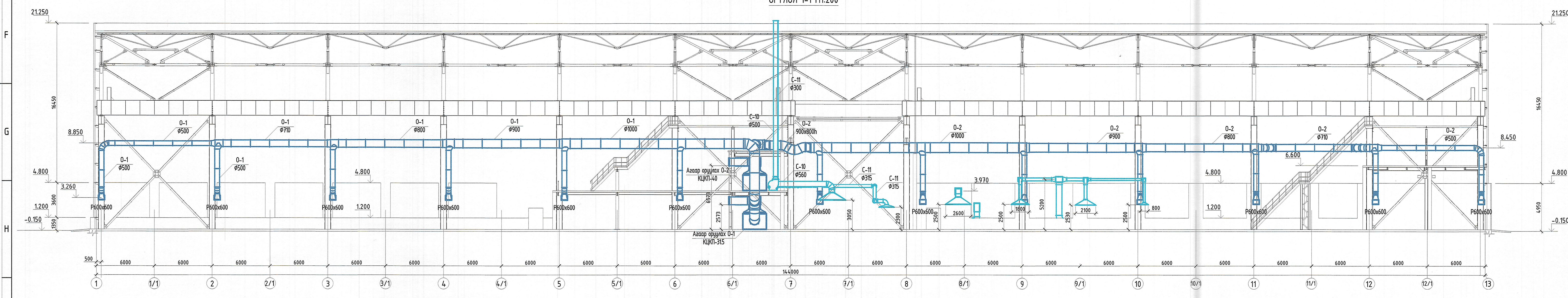
ОГТЛОЛ 2-2 М1:200
