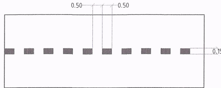
1.7 Чулзвар дээрх хөдөлгөөний эгнээний хилийг тэмдэглэх L1=0.50; L2=0.50
