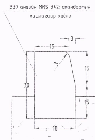
АВТО ЗАМЫН ХАШЛАГА SCALE 1:20
