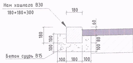
ЯВГАН ХҮНИЙ ЗАМЫН ГАРЦНЫ ХАШЛАГА SCALE 1:20
