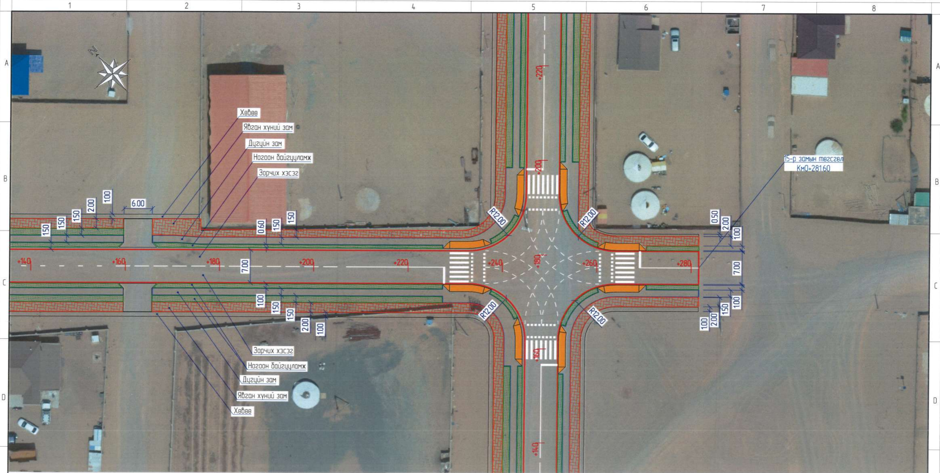
ЗАМЫН СХЕМ 15-р зам
