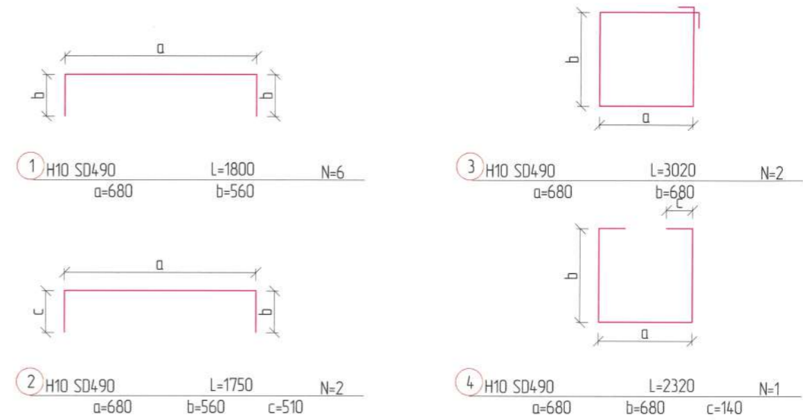
АРМАТУРЧЛАЛЫН ТҮҮВЭР
