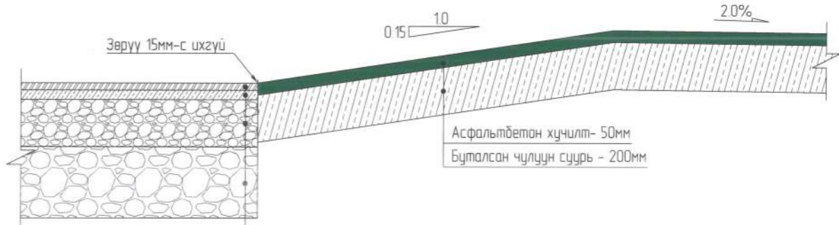
ОГТЛОЛ 2-2 М 1:20
