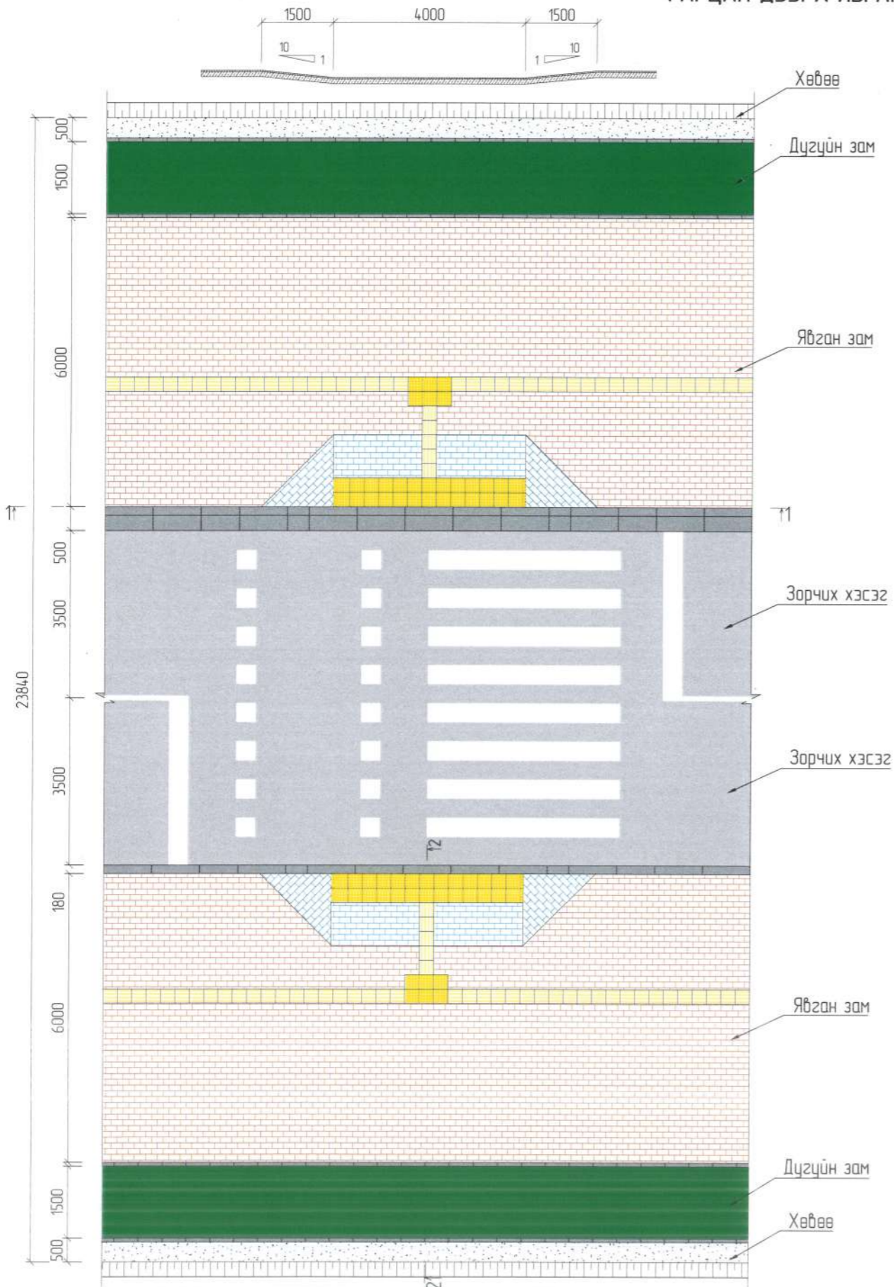
ОГТ/ЛОЛ 1-1
