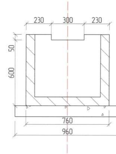
ОГТЛОЛ 2-2
