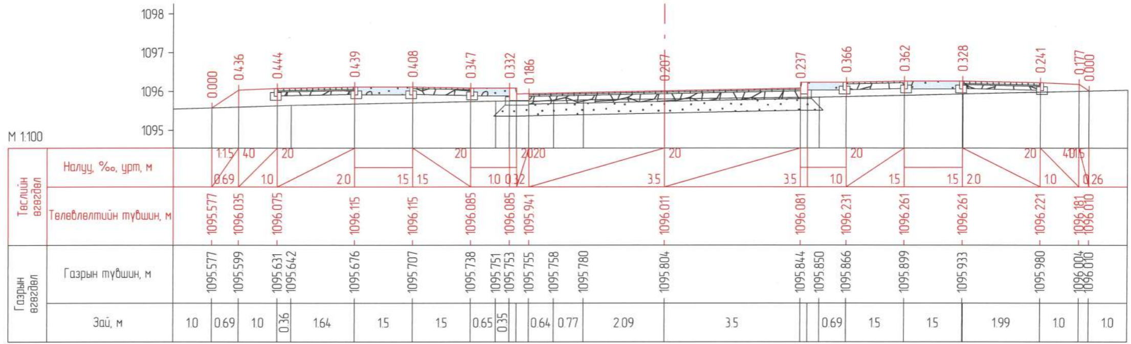
ПК 0+160.000
