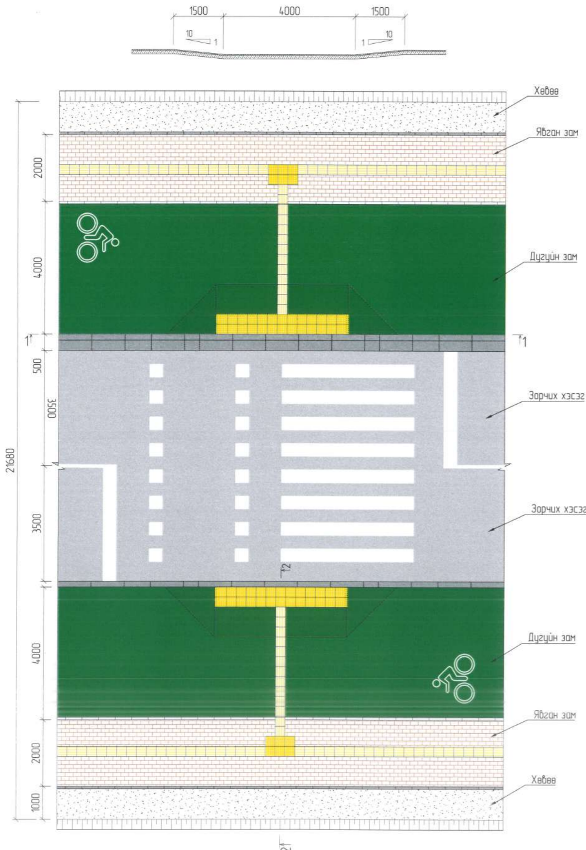
ОГТЛОЛ 1-1
