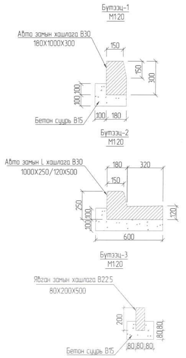
БЕТОН ХИЙЦ БҮТЭЭЦ
