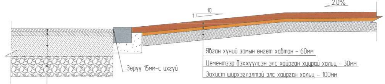
ОГТ/ЛОЛ 2-2 М 1:20
