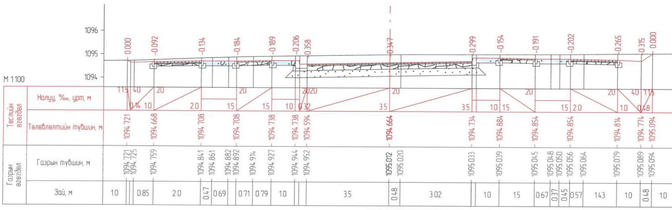
ПК 0+060.000
