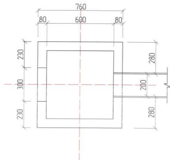
ПЛАН
