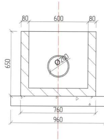
ОГТЛОЛ 1-1
