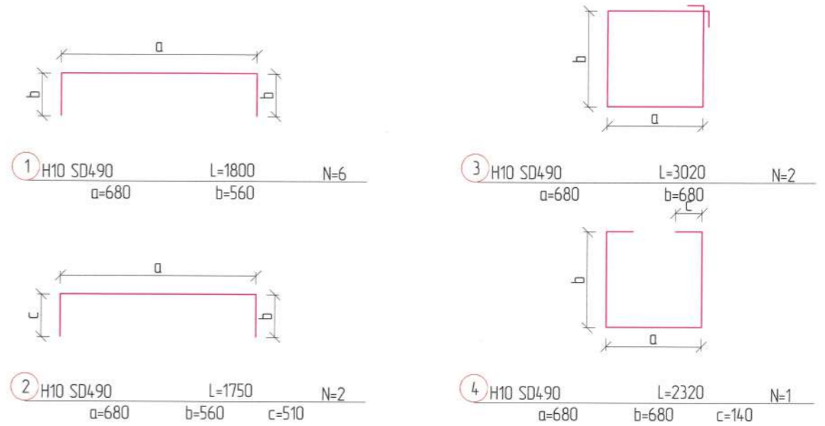
АРМАТУРЧЛАЛЫН ТҮҮВЭР
