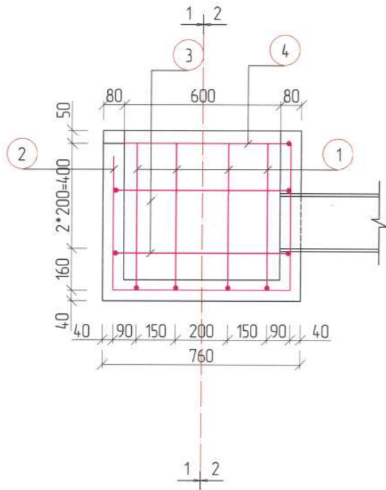
ХӨНДЛӨН ОГТЛОЛ
