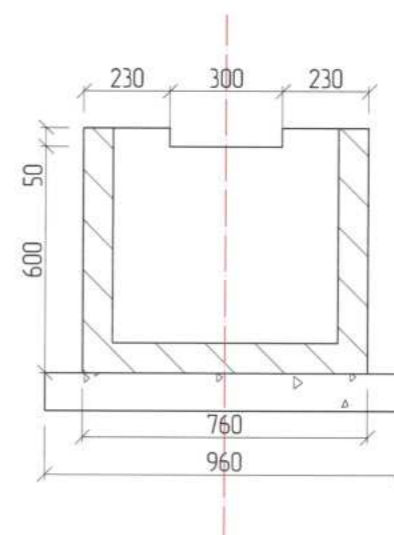
ОГТЛОЛ 2-2
