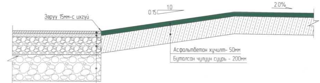
ОГТЛОЛ 2-2 М 1:20
