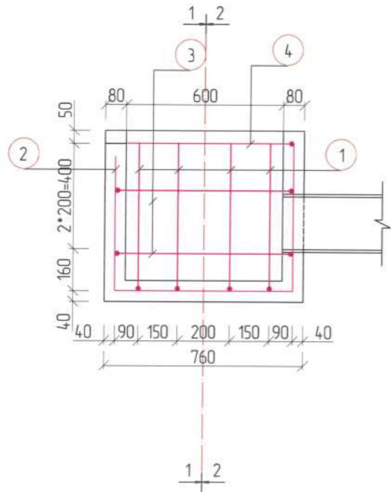
ХӨНДЛӨН ОГТЛОЛ
