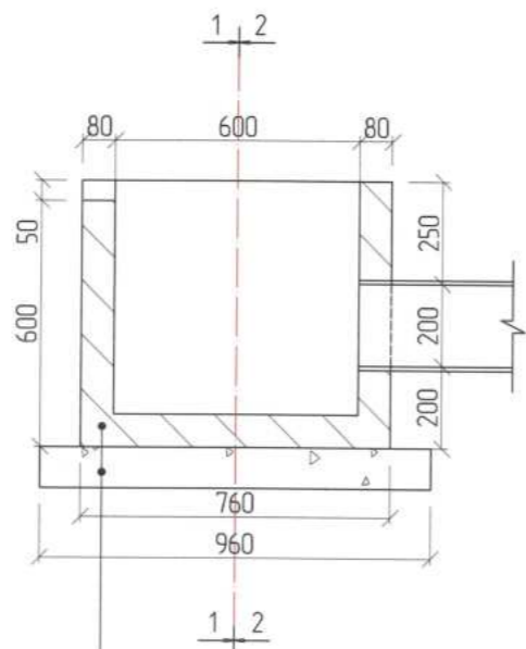
ХӨНДЛӨН ОГТЛОЛ
