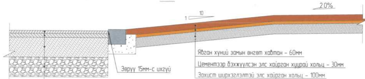
ОГТЛОЛ 2-2 М 1:20
