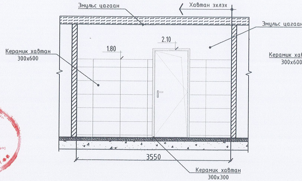
Ханын дэлгээс-В М1:100
