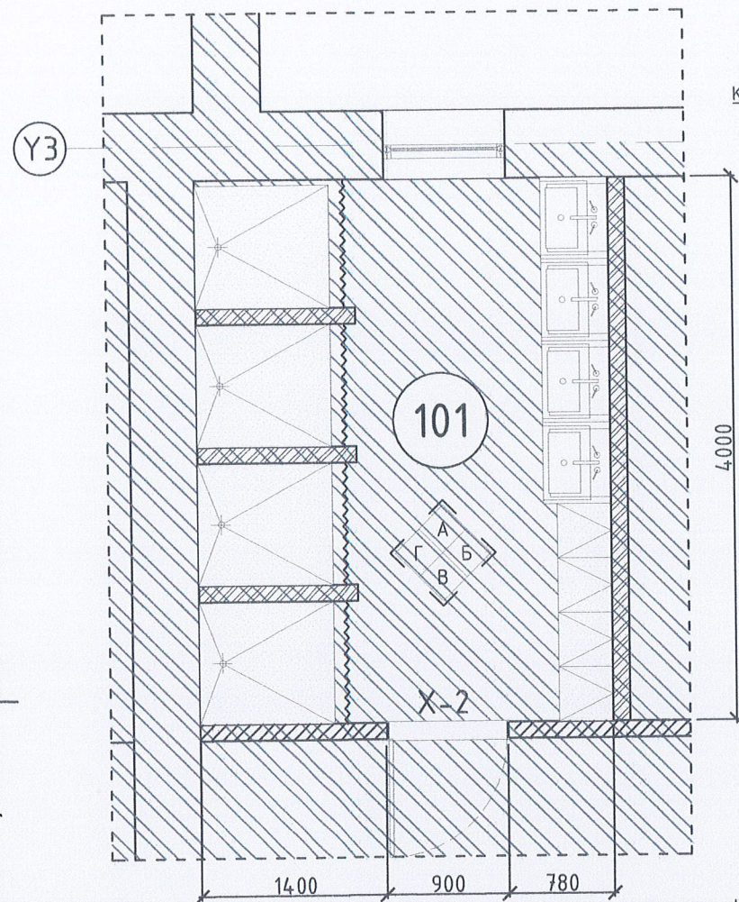
ХЭСЭГЧИЛСЭН БАЙГУУЛАЛТ-1 М1:100
