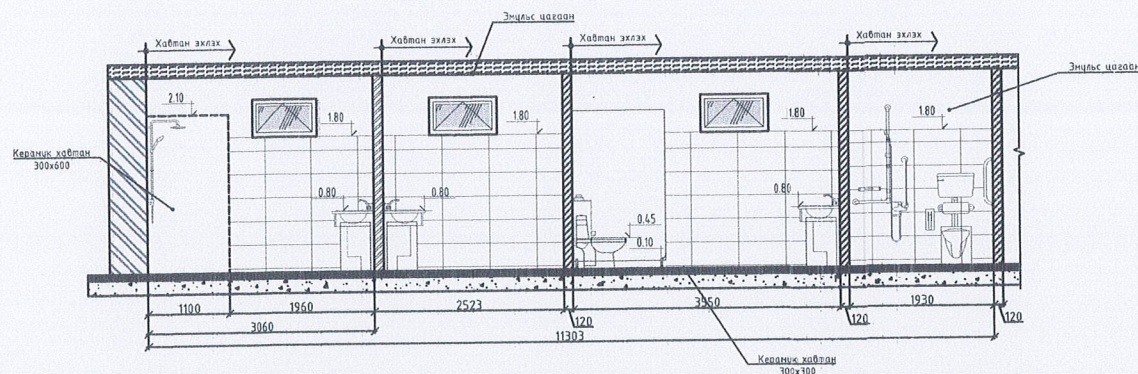
ОГТЛОЛ 1-1 M1:100
