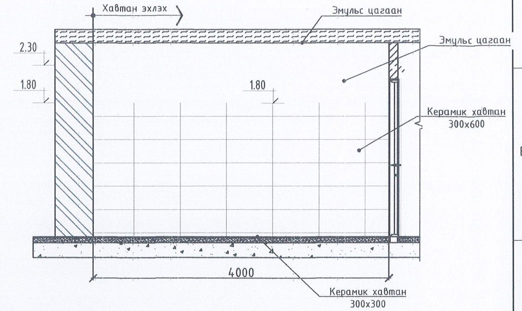
Ханын дэлгээс-Б M1:100
