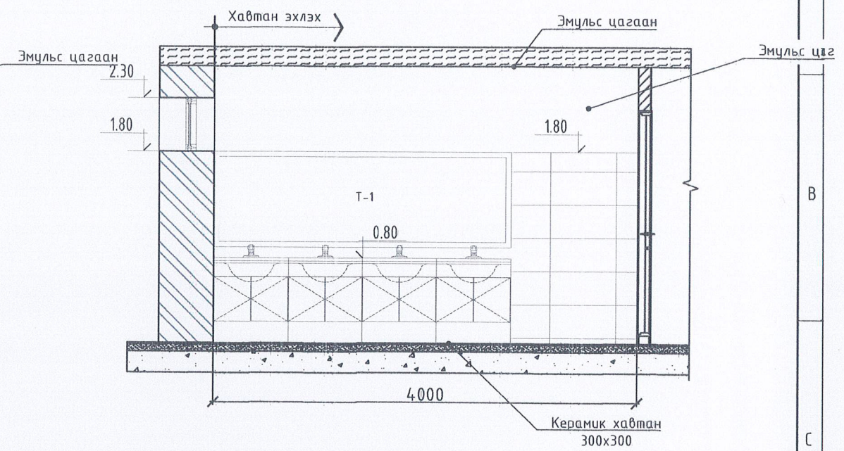
Ханын дэлгээс-Б М1:100
