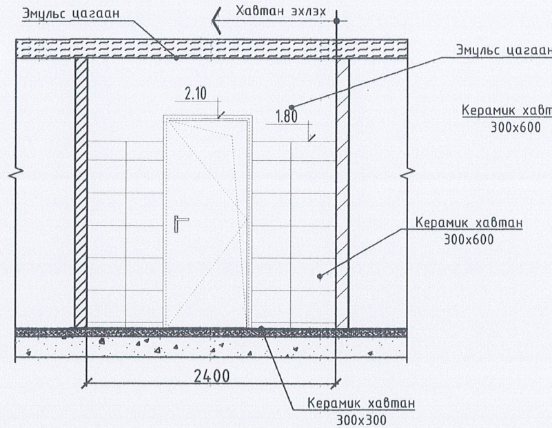
Ханын дэлгээс-В M1:100
