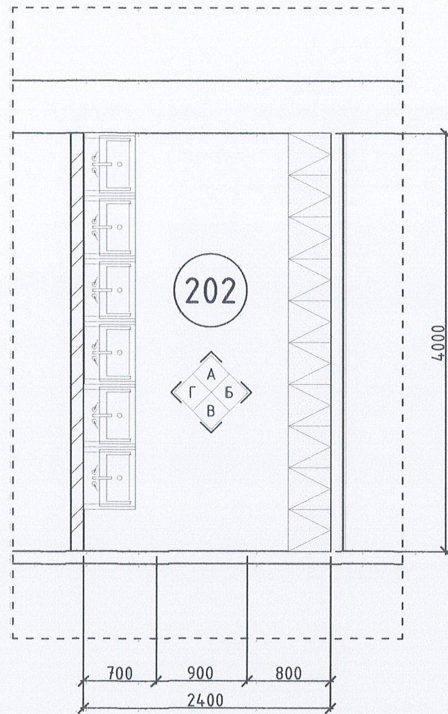
ХЭСЭГЧИЛСЭН БАЙГУУЛАЛТ-1 M1:100
