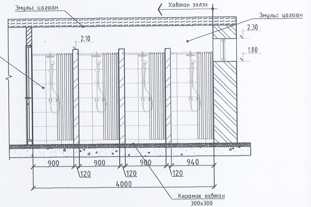
Ханын дэлгээс-Г М1:100
