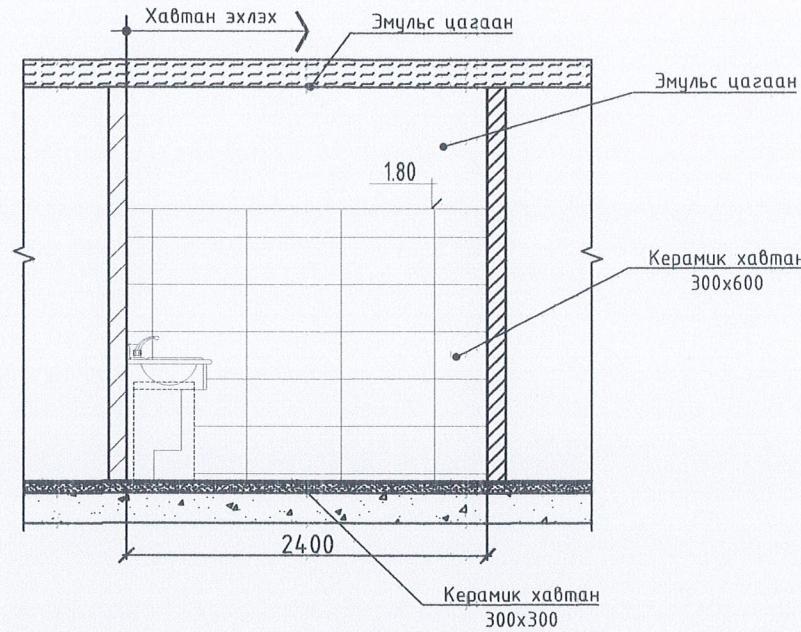
Ханын дэлгээс-А M1:100
