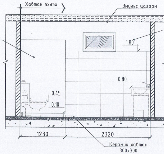
Ханын дэлгээс-А М1:100
