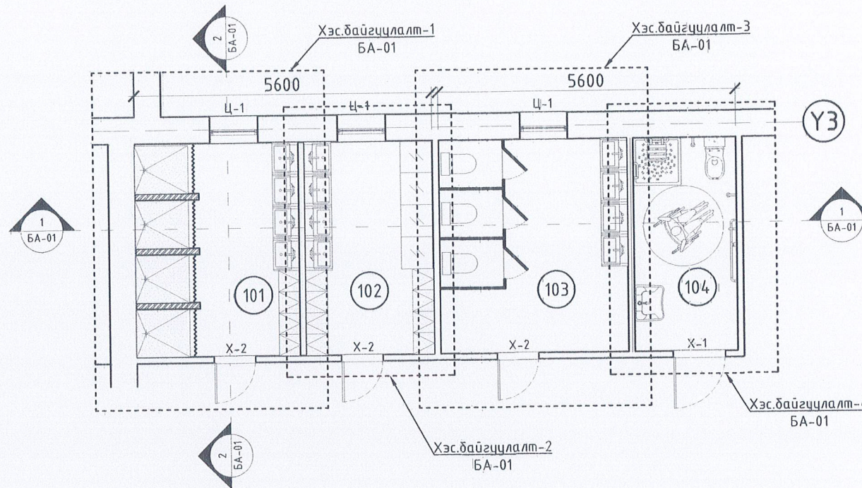
ӨӨРЧЛӨЛТИЙН БАЙГУУЛАЛТ M1:100
