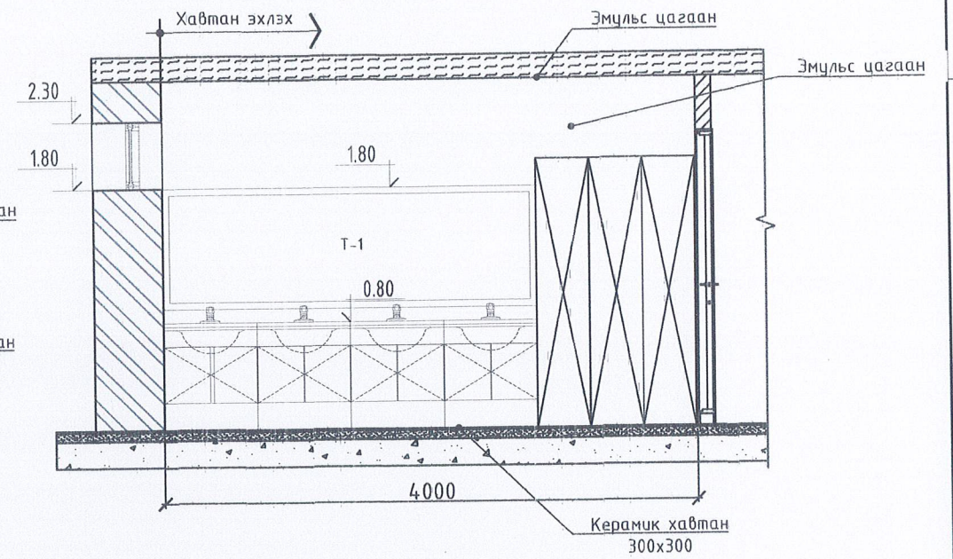
Ханын дэлгээс-Б М1:100
