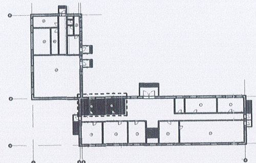
ТҮЛХҮҮР БАЙГУУЛАЛТ
