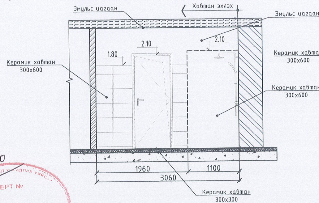
Ханын дэлгээс-В М1:100
