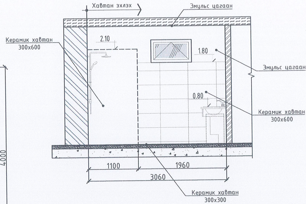
Ханын дэлгээс-А М1:100
