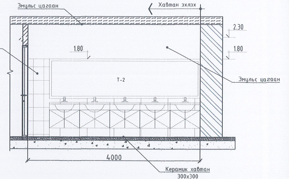
Ханын дэлгээс-Г M1:100
