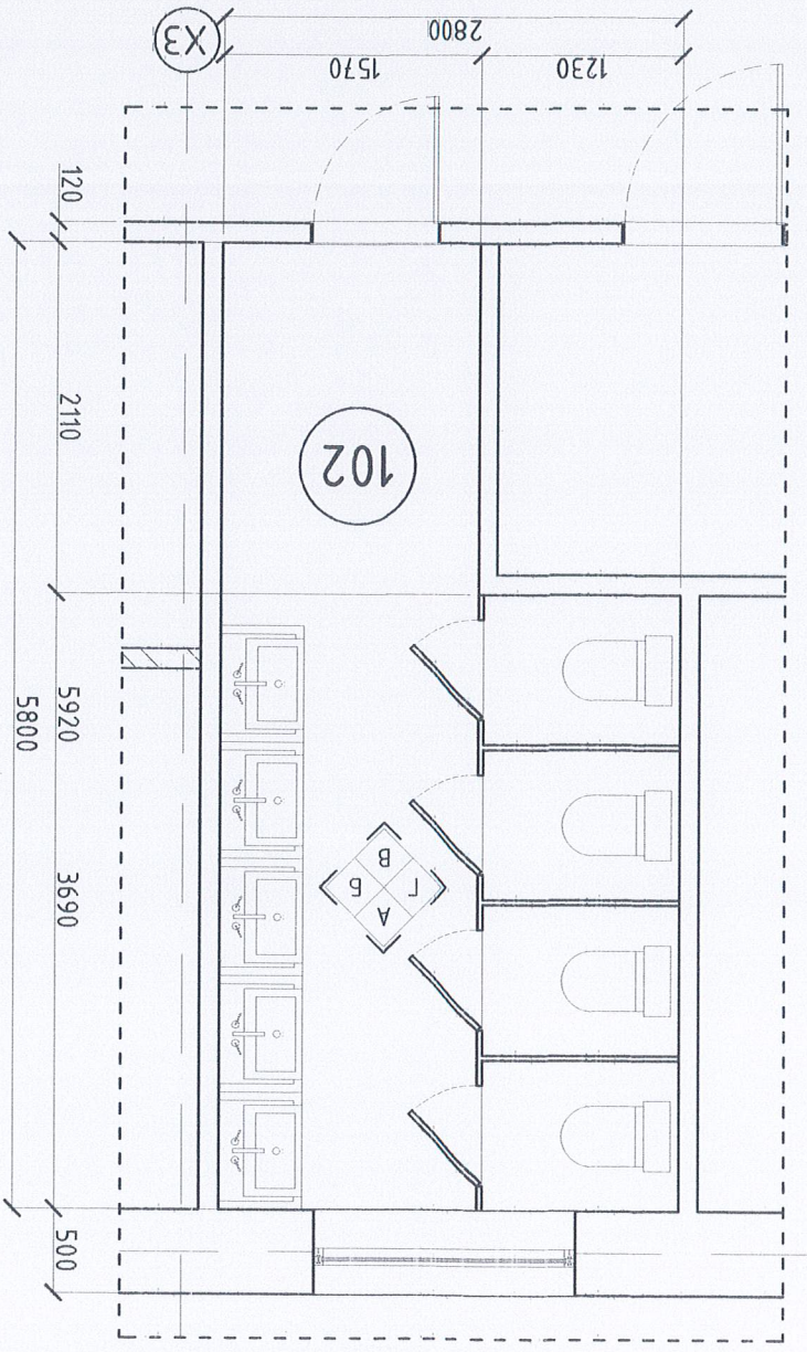
ХЭСЭГЧИЛСЭН БАЙГУУЛАЛТ-2 М1:100
