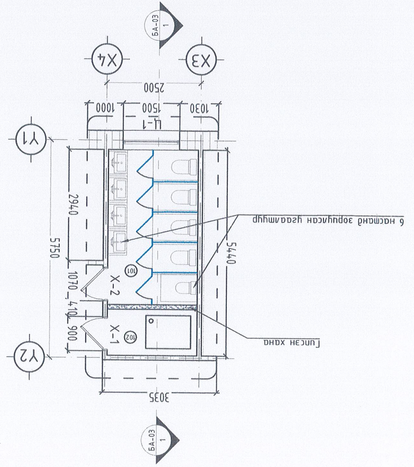
ӨӨРЧЛӨЛТИЙН БАЙГУУЛАЛТ М:100
