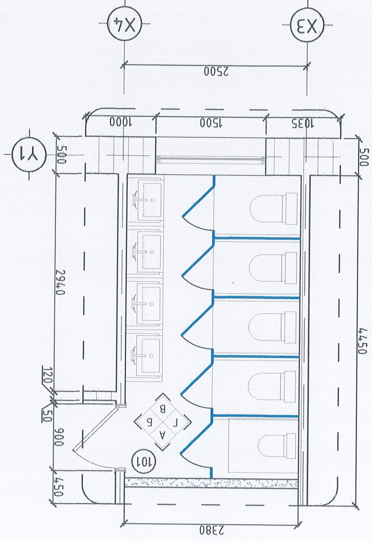
ХЭСЭГЧИЛСЭН БАЙГУУЛАЛТ-101 М:50
