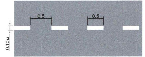
1.7 Уулзвар дээрх хөдөлгөөний эгнээг тэмдэглэх ( V < 60 км/цаг; L1 = 1.00 - 3.00 ; L2 = 3.00 - 9.00 ) ( L1 : L2 = 1 : 3 )
