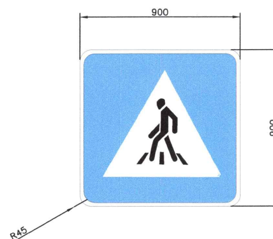
1.13 а Зохицуулдаггүй явган хүний гарц
