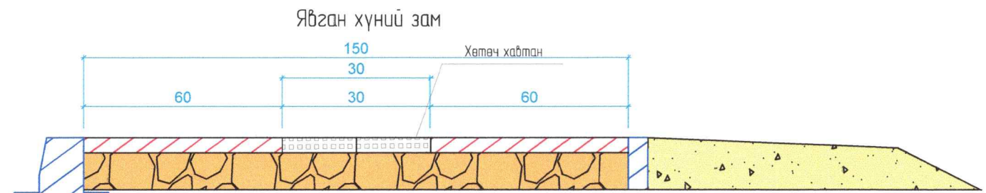
АНХААРУУЛГЫН ХАВТАН М110
