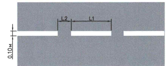
1.6 Үргэлжилсэн дагуу шугаман тэмдэглэлд ойртож байгааг тэмдэглэх ( V < 60 км/цаг; L1 = 3.00 - 6.00 ; L2 = 1.00 - 2.00 ) ( L1 : L2 = 3 : 1 )
