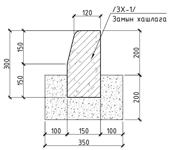
ОГТЛОЛ 1-1 АВТО ЗАМЫН ХАШЛАГА /ЗХ-1/ М1:10
