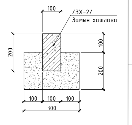
ОГТЛОЛ 2-2 ЯВГАН ЗАМЫН ХАШЛАГА /ЗХ-2/ М1:10
