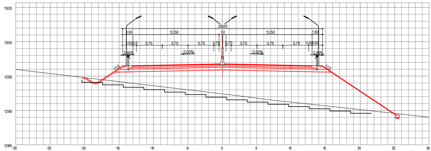
ЗАЙ / STA. 29+880.00
