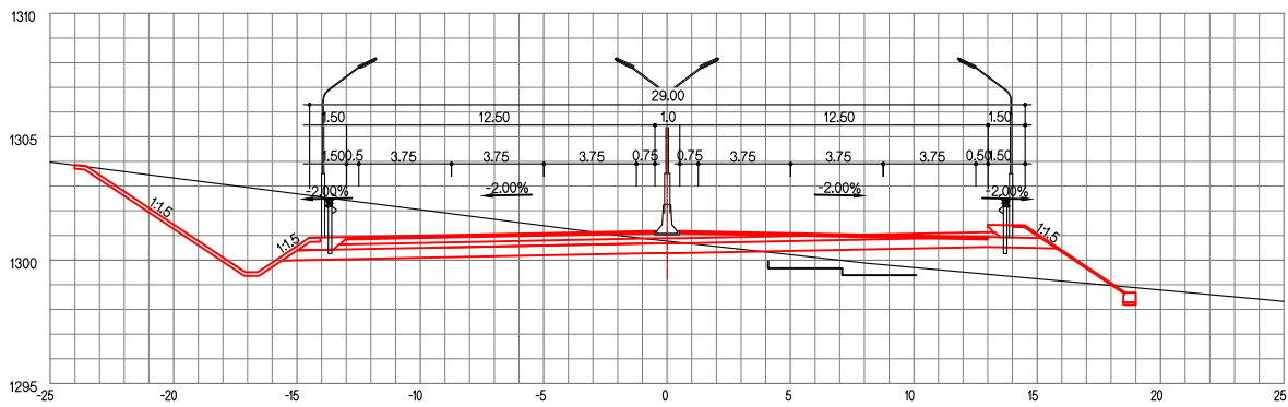
ЗАЙ / STA. 30+140.00
