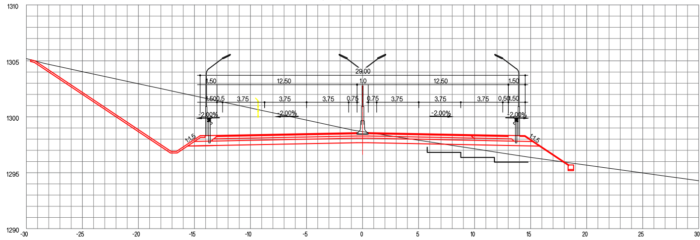
ЗАЙ / STA. 30+040.00
