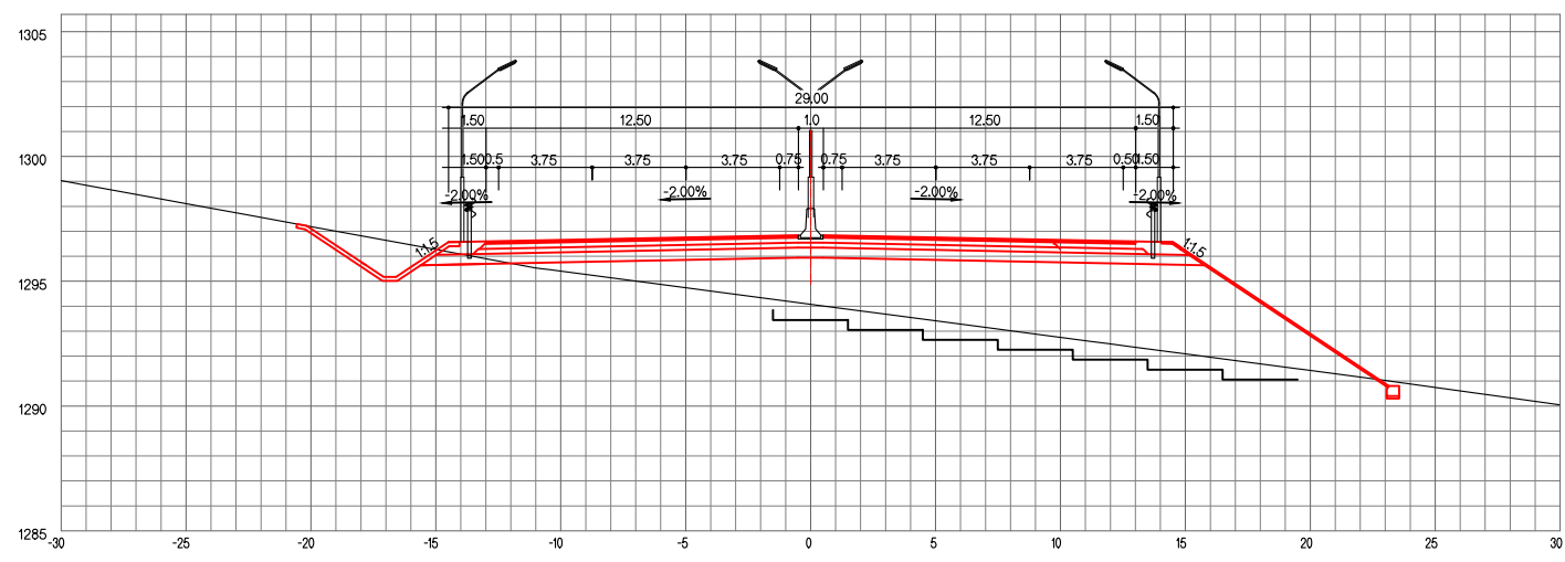
ЗАЙ / STA. 29+940.00
