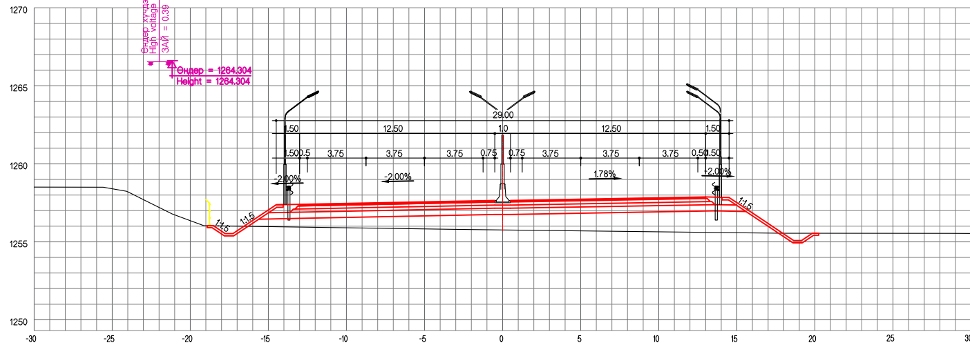
Зай / STA. 23+580.00
