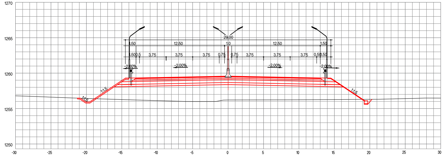
ЗАЙ / STA. 22+880.00
