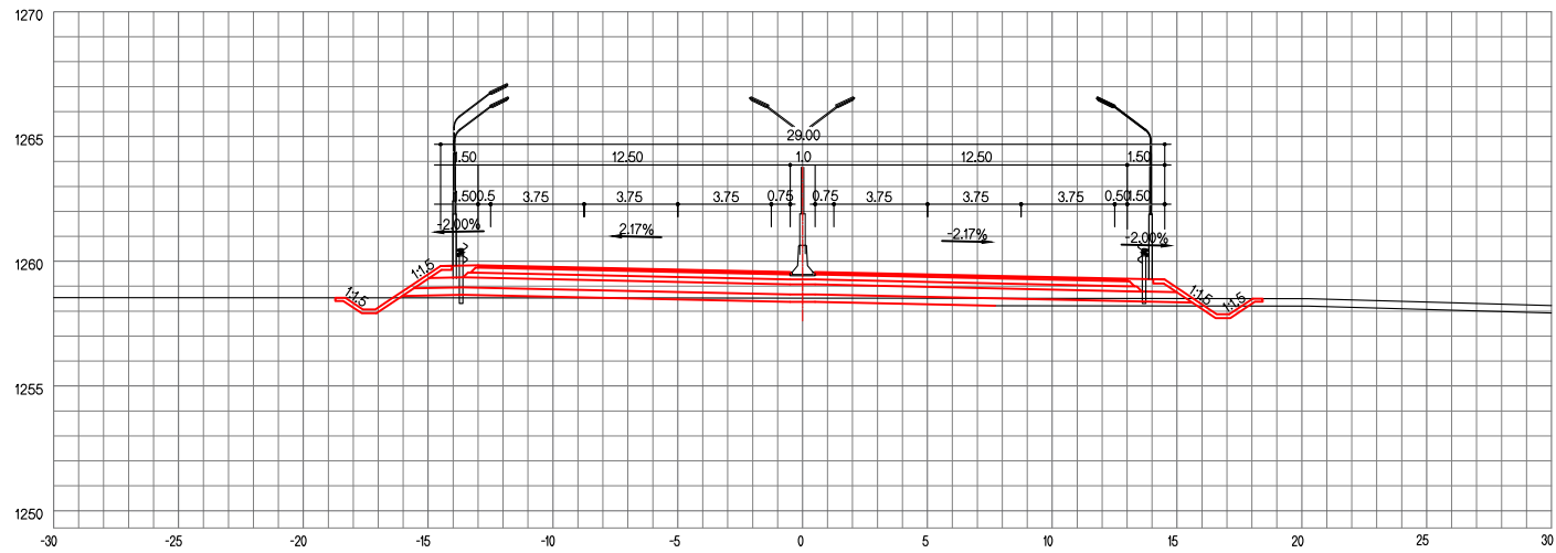
ЗАЙ / STA. 22+140.00
