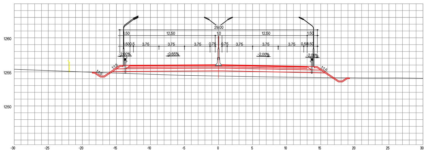
ЗАЙ / STA. 23+740.00
