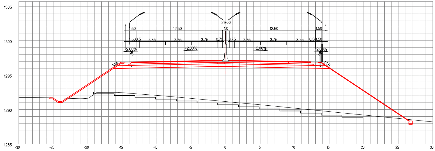
ЗАЙ / STA. 29+740.00
