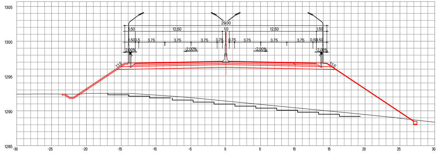
ЗАЙ / STA. 29+720.00
