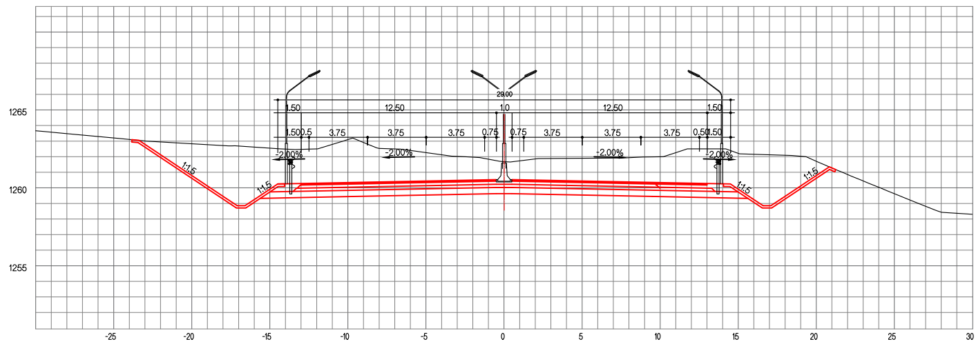
ЗАЙ / STA. 28+720.00
