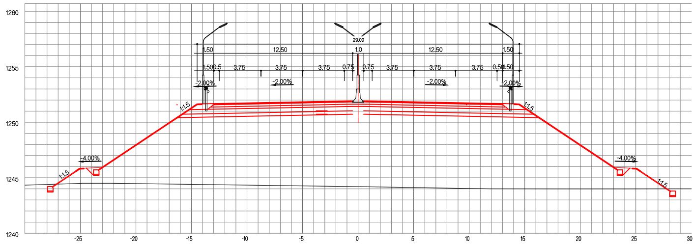
ЗАЙ / STA. 28+380.00
