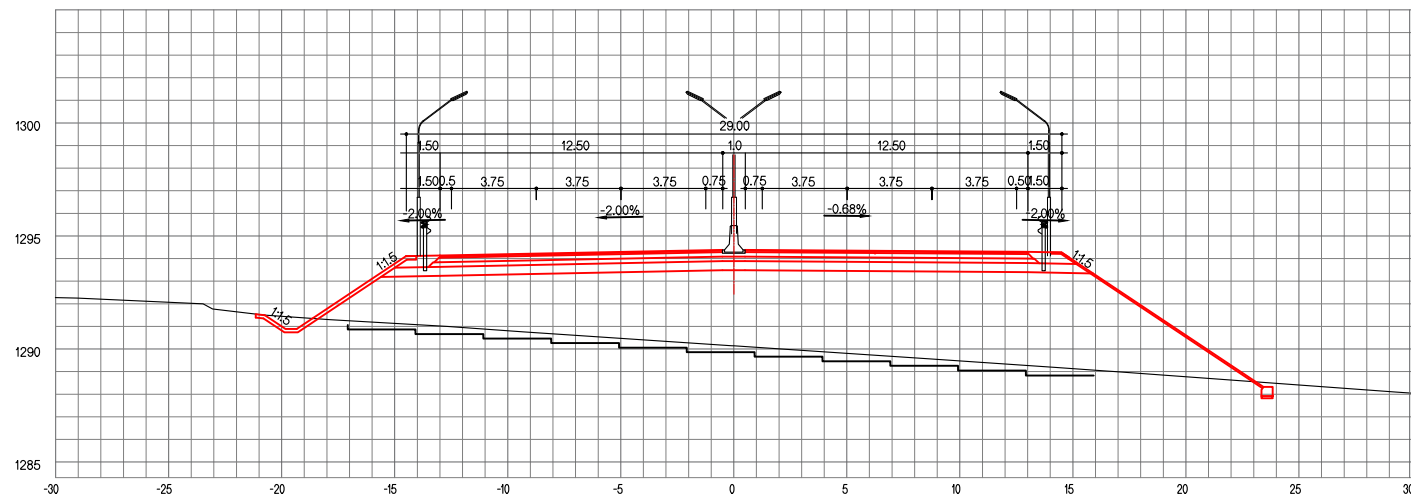
ЗАЙ / STA. 29+580.00
