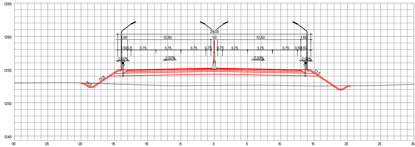
ЗАЙ / STA. 24+620.00
