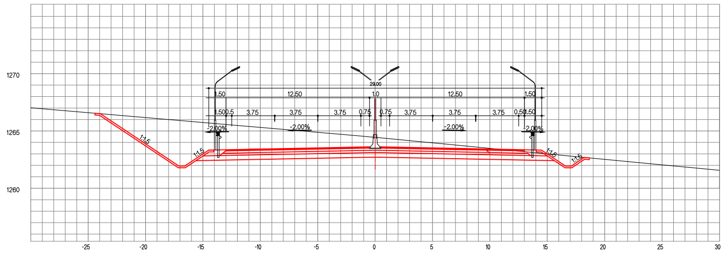
ЗАЙ / STA. 28+800.00
