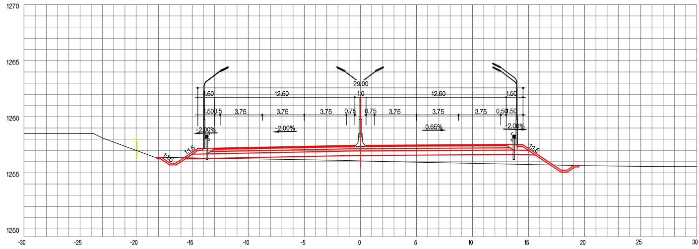
ЗАЙ / STA. 23+600.00
