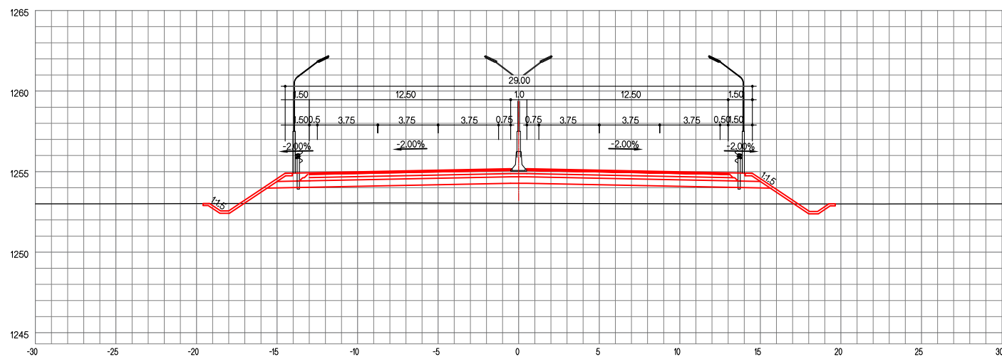
ЗАЙ / STA. 24+580.00
