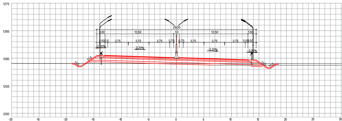
ЗАЙ / STA. 21+900.00
