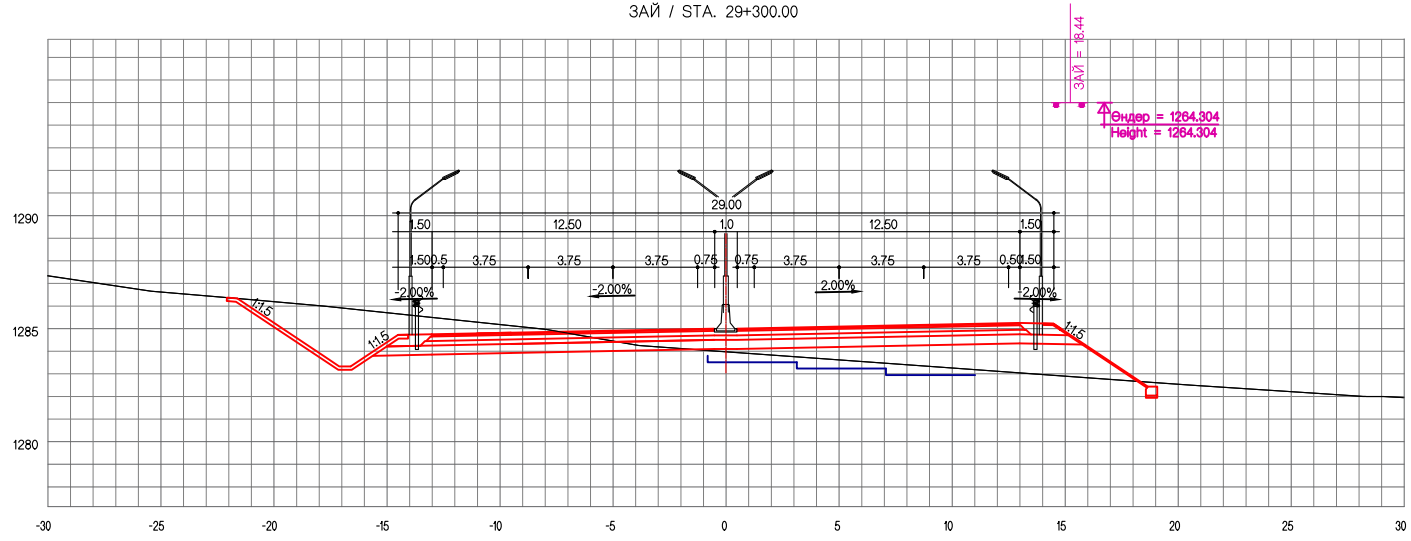
ЗАЙ / STA. 29+300.00
