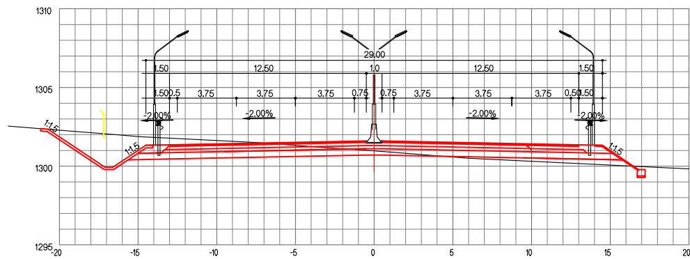
Зай / STA. 30+260.00
