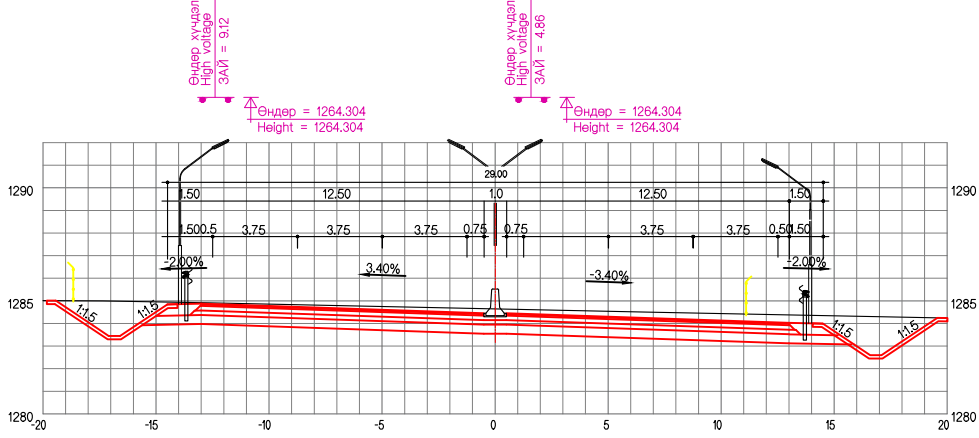
ЗАЙ / STA. 31+820.00
