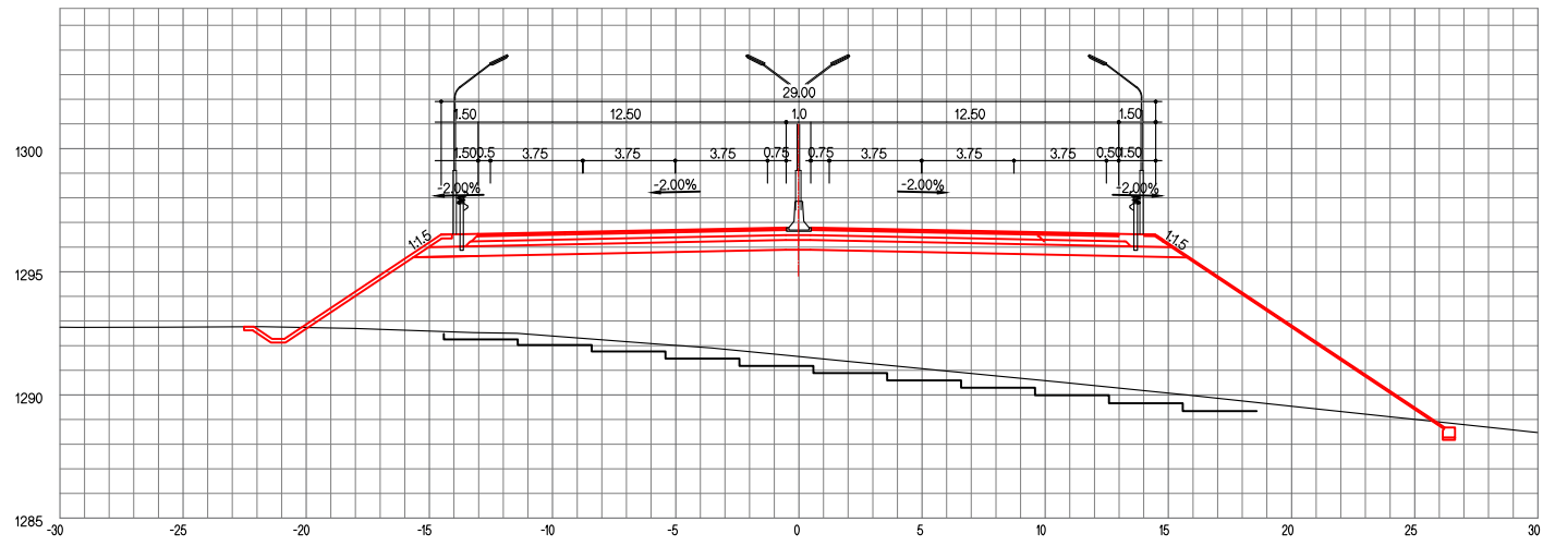
ЗАЙ / STA. 29+680.00
