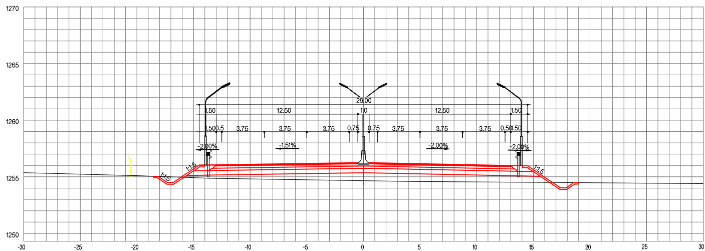
ЗАЙ / STA. 23+720.00
