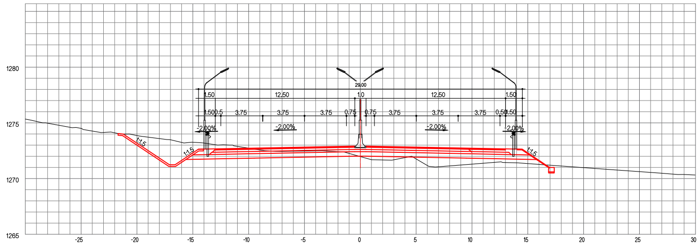
ЗАЙ / СТА. 29+040.00
