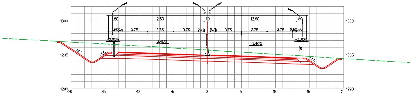
ЗАЙ / STA. 30+600.00
