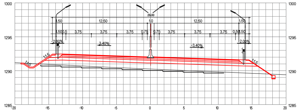
ЗАЙ / STA. 30+740.00
