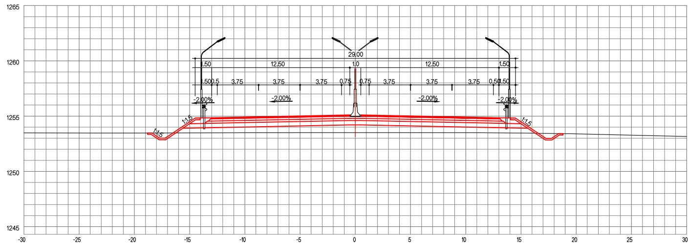
ЗАЙ / STA. 24+480.00
