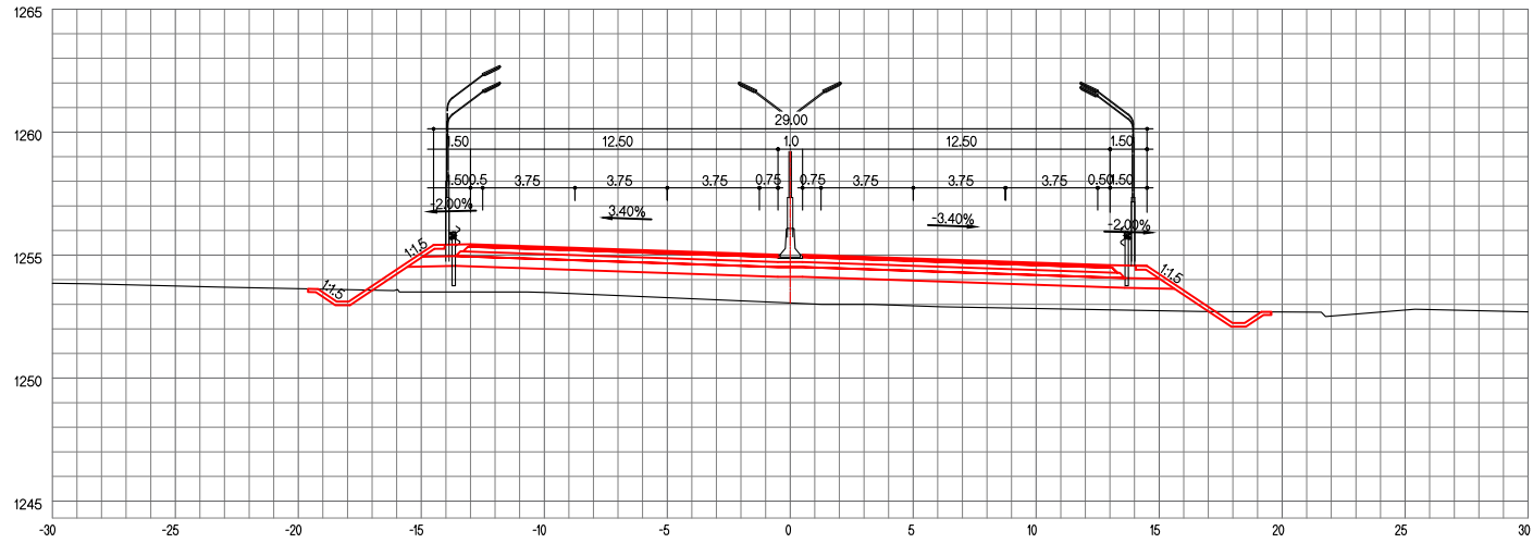
ЗАЙ / STA. 23+860.00
