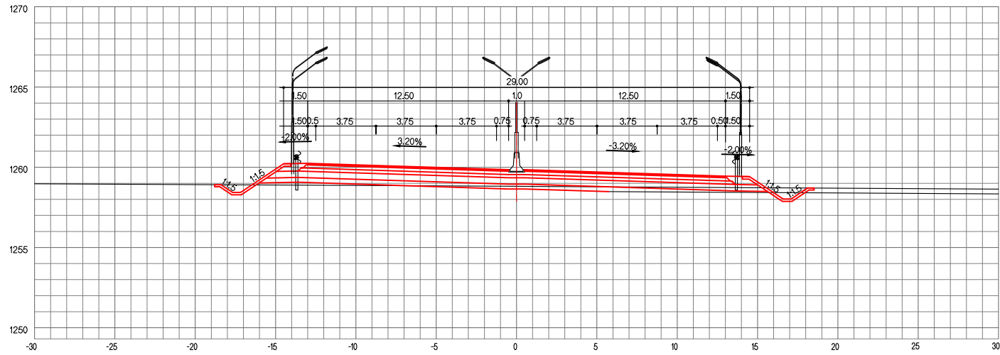
ЗАЙ / СТА. 22+020.00
