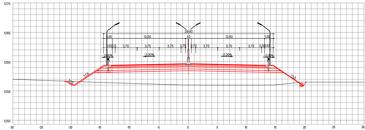
ЗАЙ / STA. 22+900.00
