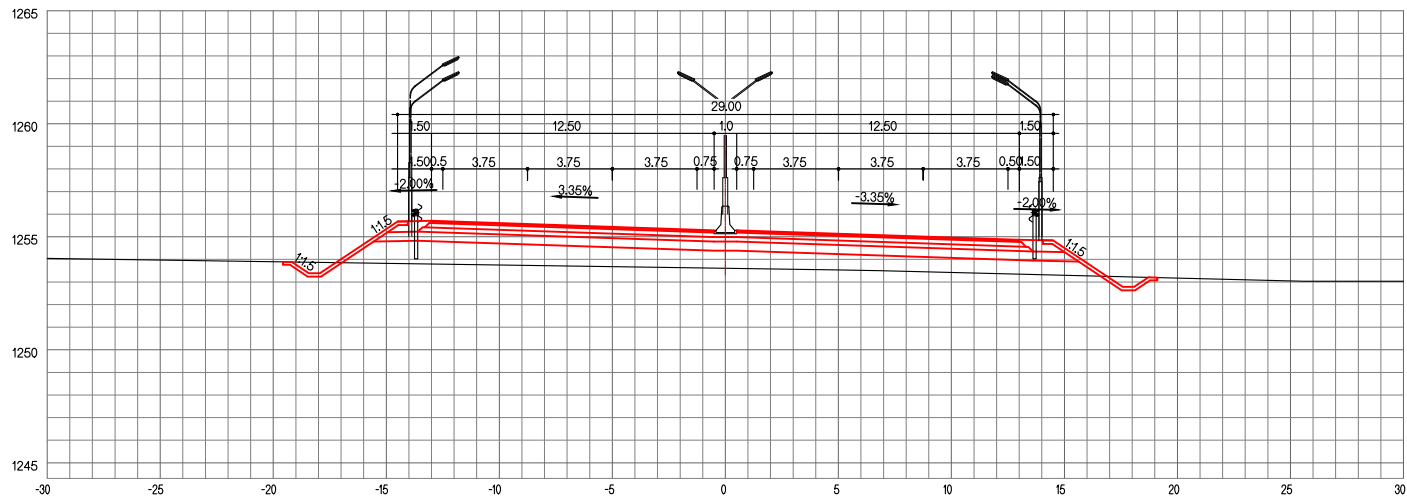
ЗАЙ / СТА. 23+820.00
