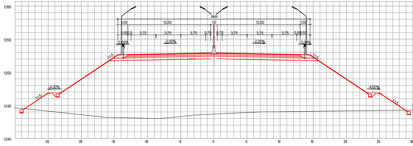
ЗАЙ / СТА. 28+480.00
