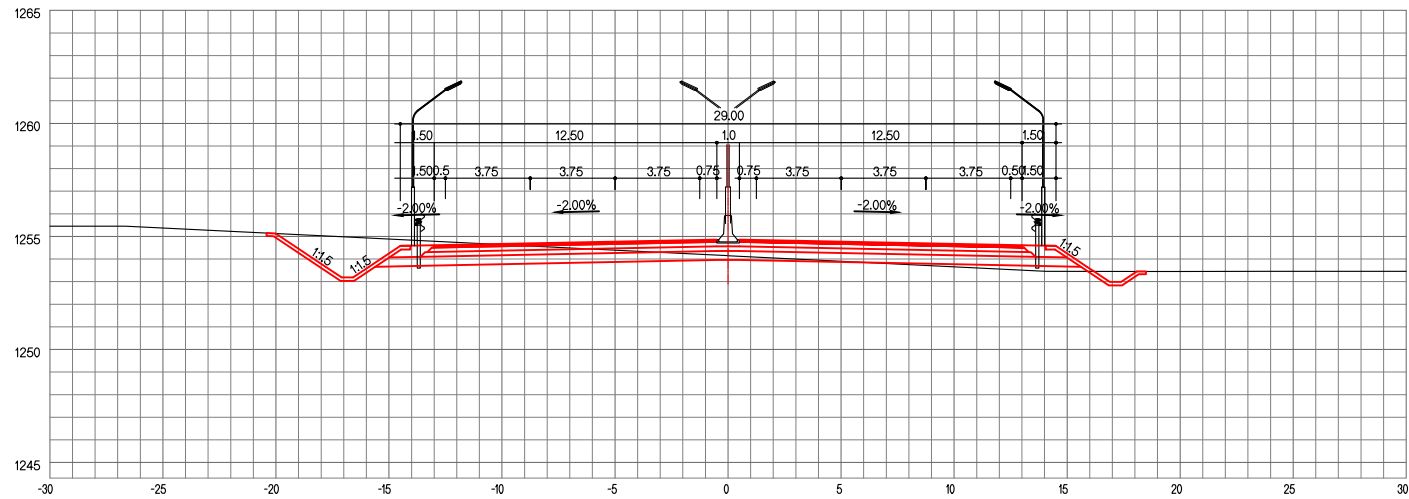
ЗАЙ / СТА. 24+220.00
