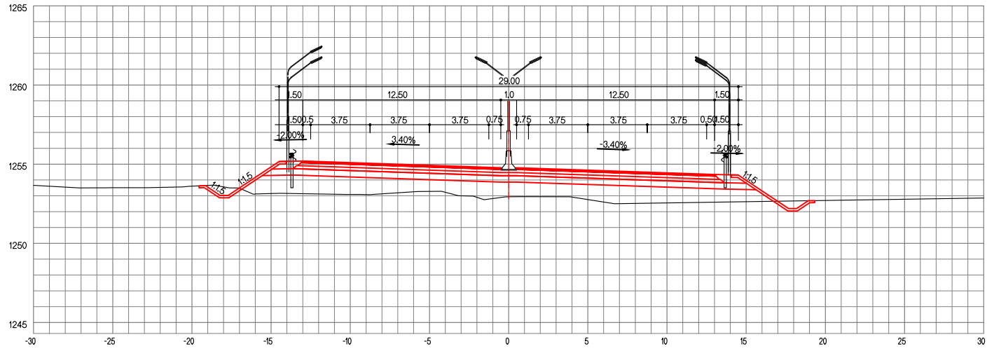
ЗАЙ / STA. 23+920.00
