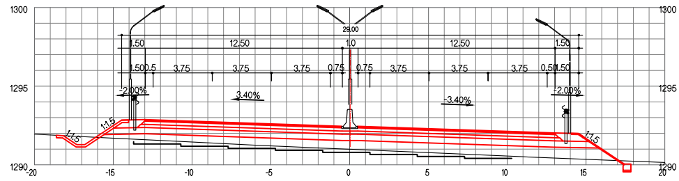
ЗАЙ / STA. 30+720.00
