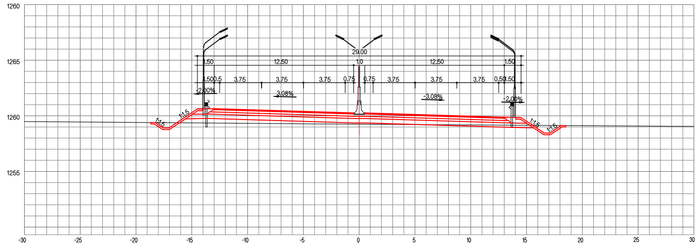
ЗАЙ / СТА. 21+840.00
