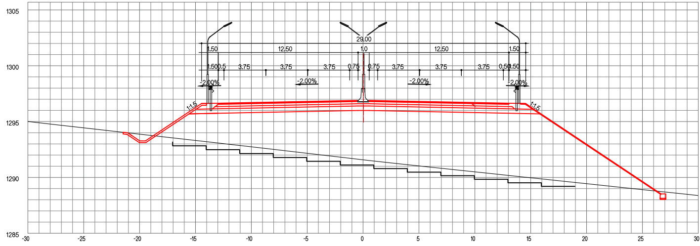
ЗАЙ / STA. 29+840.00
