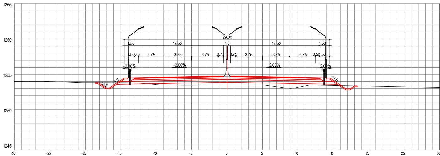
ЗАЙ / STA. 24+060.00
