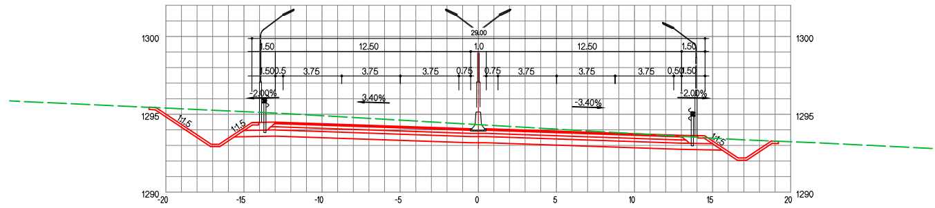
Зай / STA. 30+640.00
