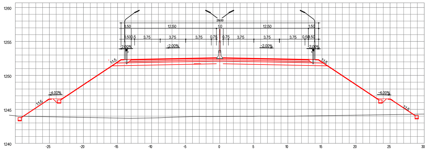
Зай / STA. 28+460.00
