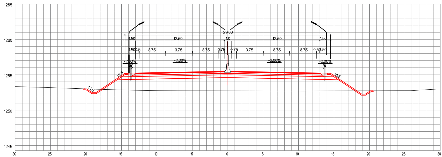
ЗАЙ / STA. 24+700.00
