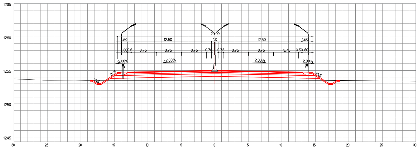
ЗАЙ / STA. 24+340.00
