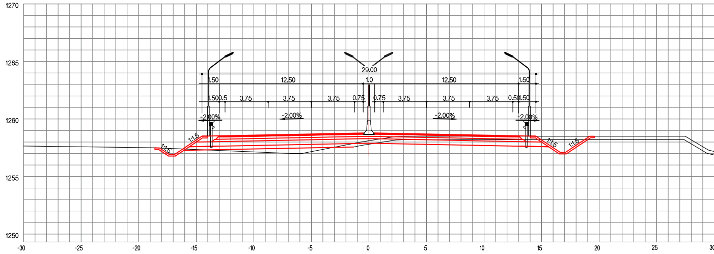
ЗАЙ / STA. 22+480.00
