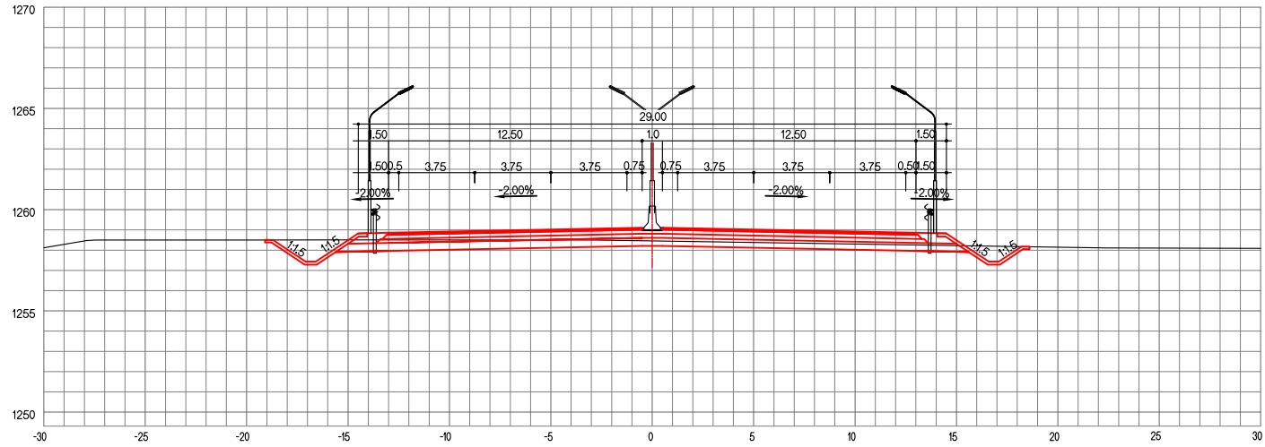
ЗАЙ / STA. 22+340.00
