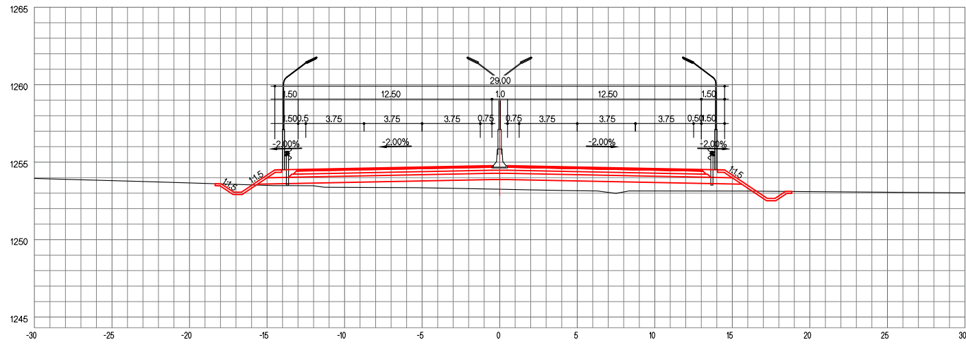
ЗАЙ / STA. 24+080.00
