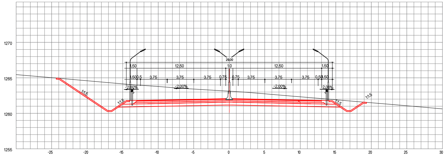
Зай / STA. 28+760.00
