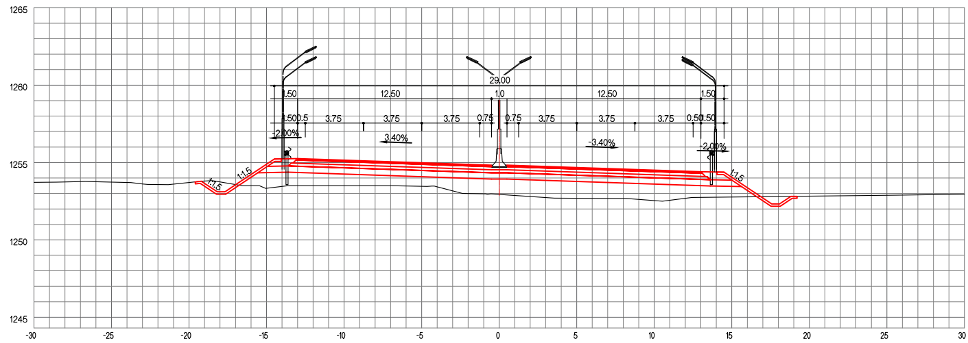
ЗАЙ / STA. 23+900.00
