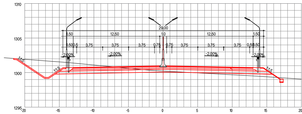
ЗАЙ / STA. 30+300.00
