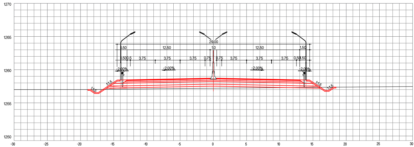
ЗАЙ / STA. 22+620.00
