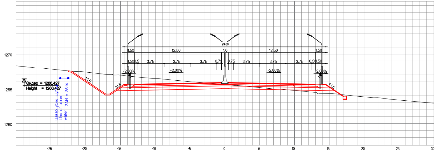
ЗАЙ / STA. 28+860.00
