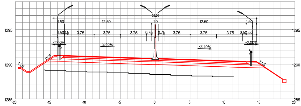
ЗАЙ / СТА. 30+800.00
