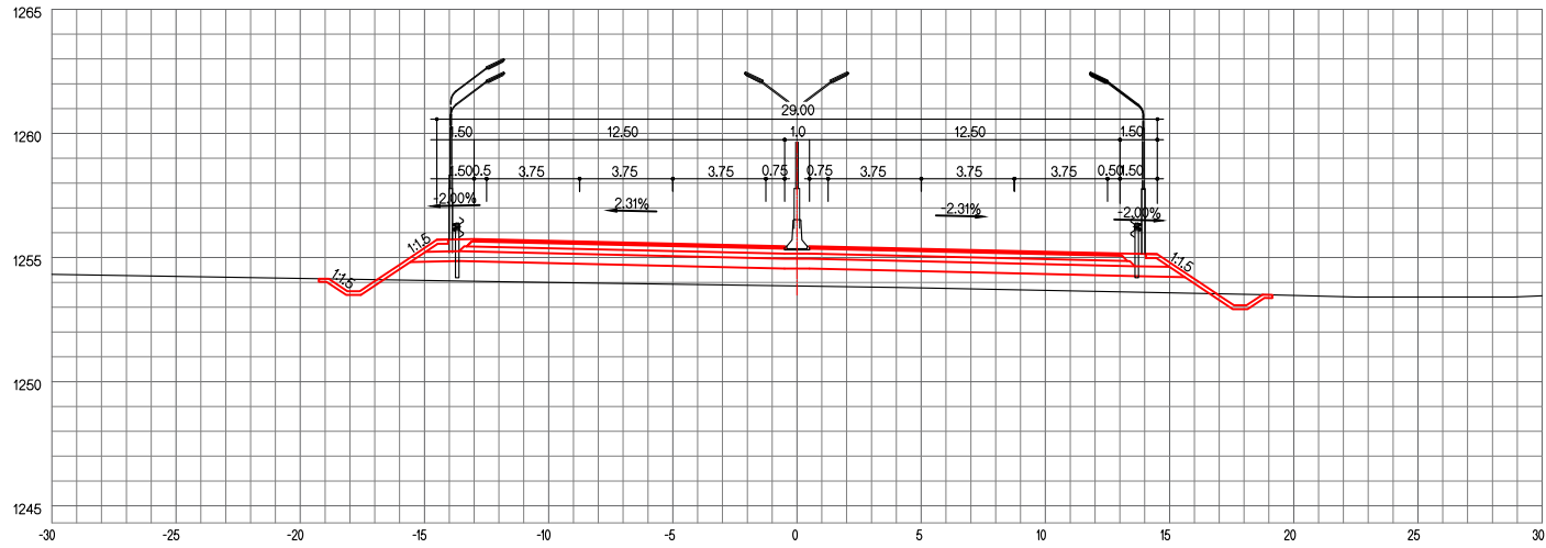
ЗАЙ / СТА. 23+800.00
