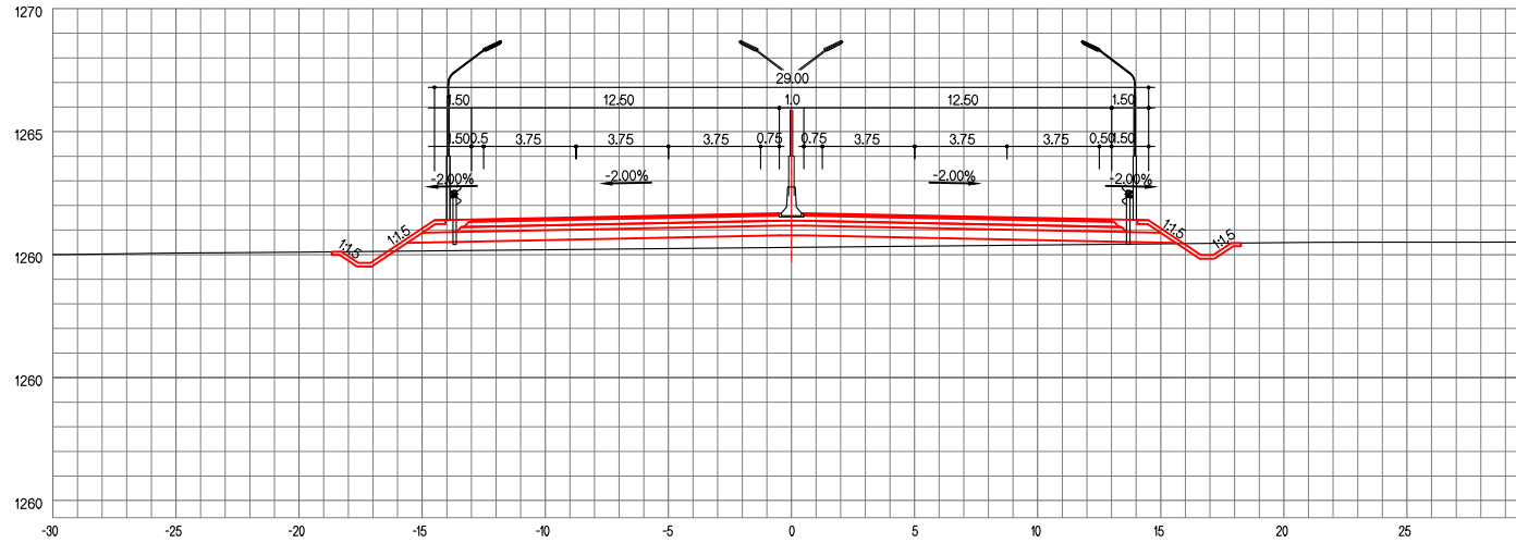
ЗАЙ / STA. 21+680.00
