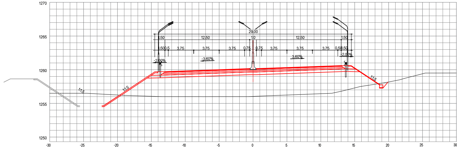
ЗАЙ / STA. 23+320.00
