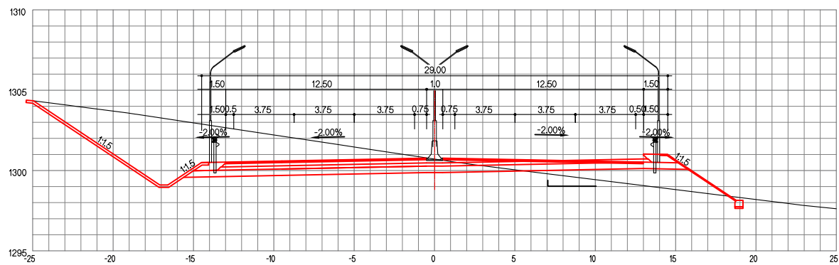
ЗАЙ / STA. 30+120.00
