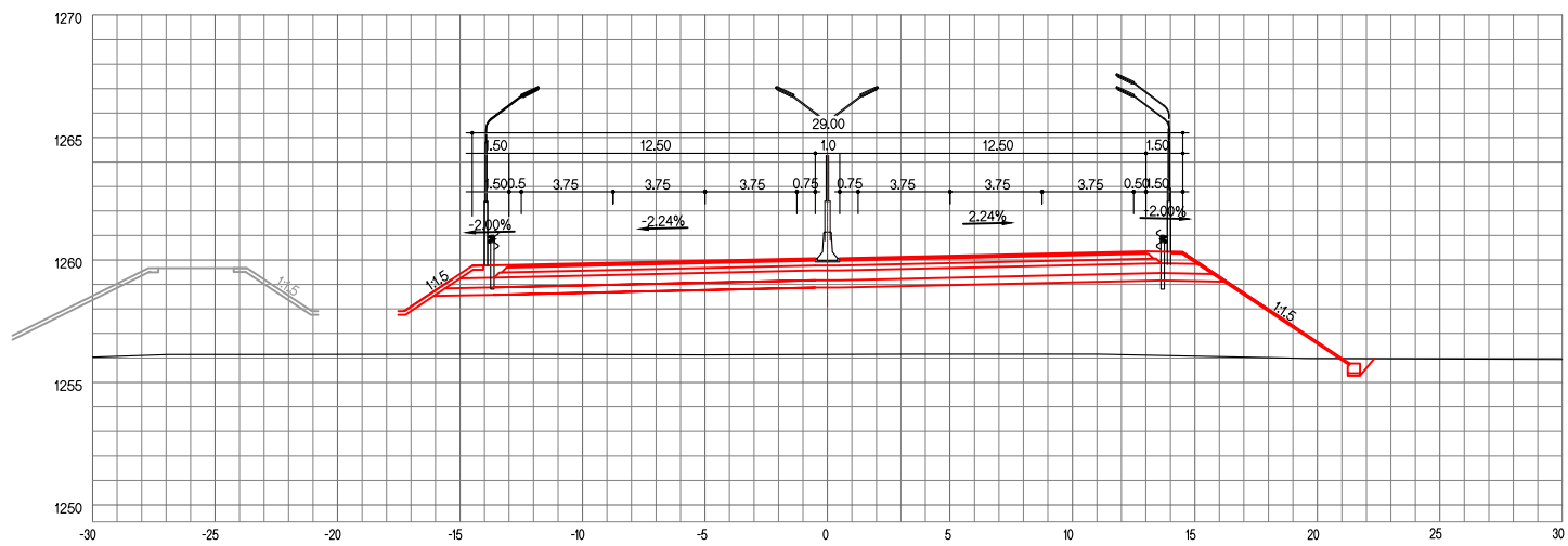
ЗАЙ / STA. 23+020.00
