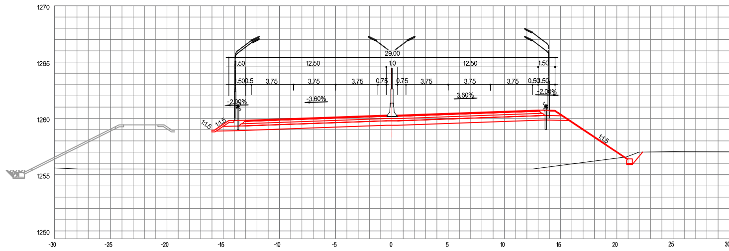
ЗАЙ / STA. 23+080.00
