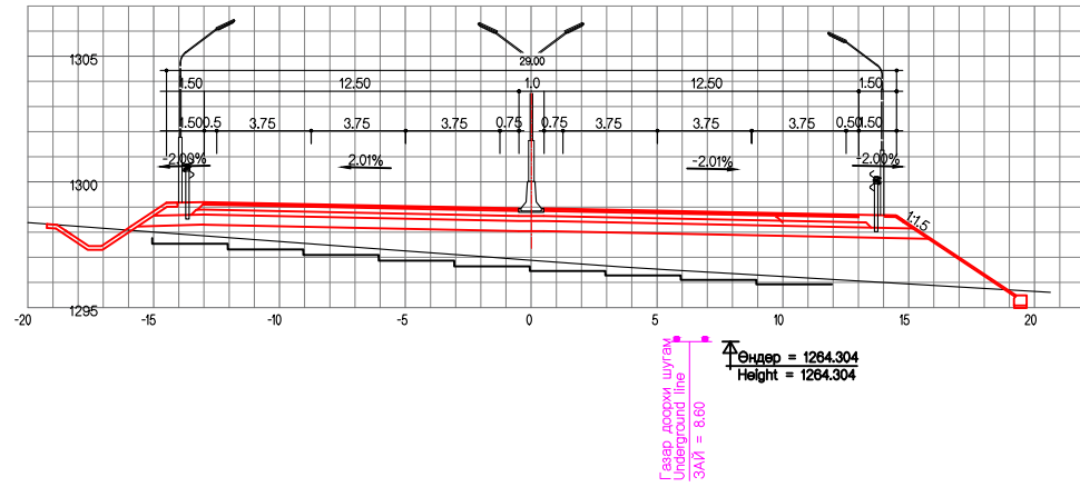
ЗАЙ / STA. 30+420.00
