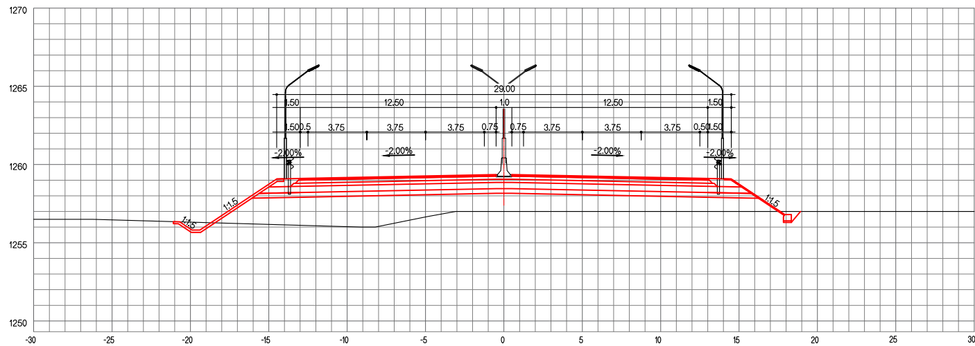
ЗАЙ / STA. 22+820.00
