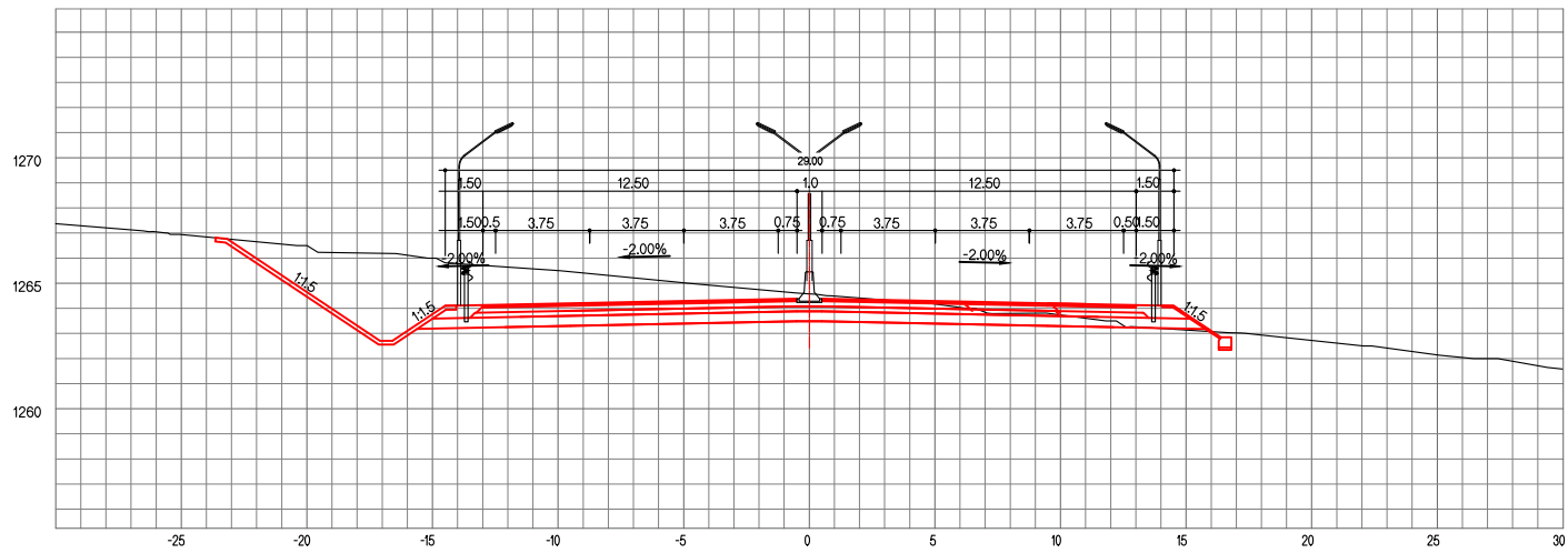
ЗАЙ / STA. 28+820.00
