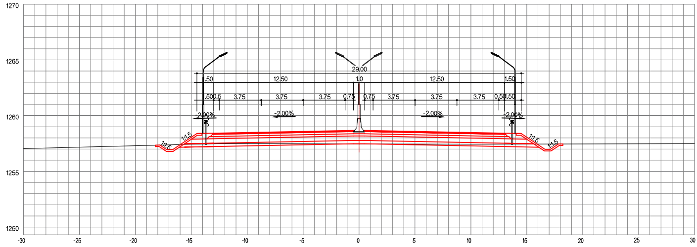
ЗАЙ / STA. 22+560.00
