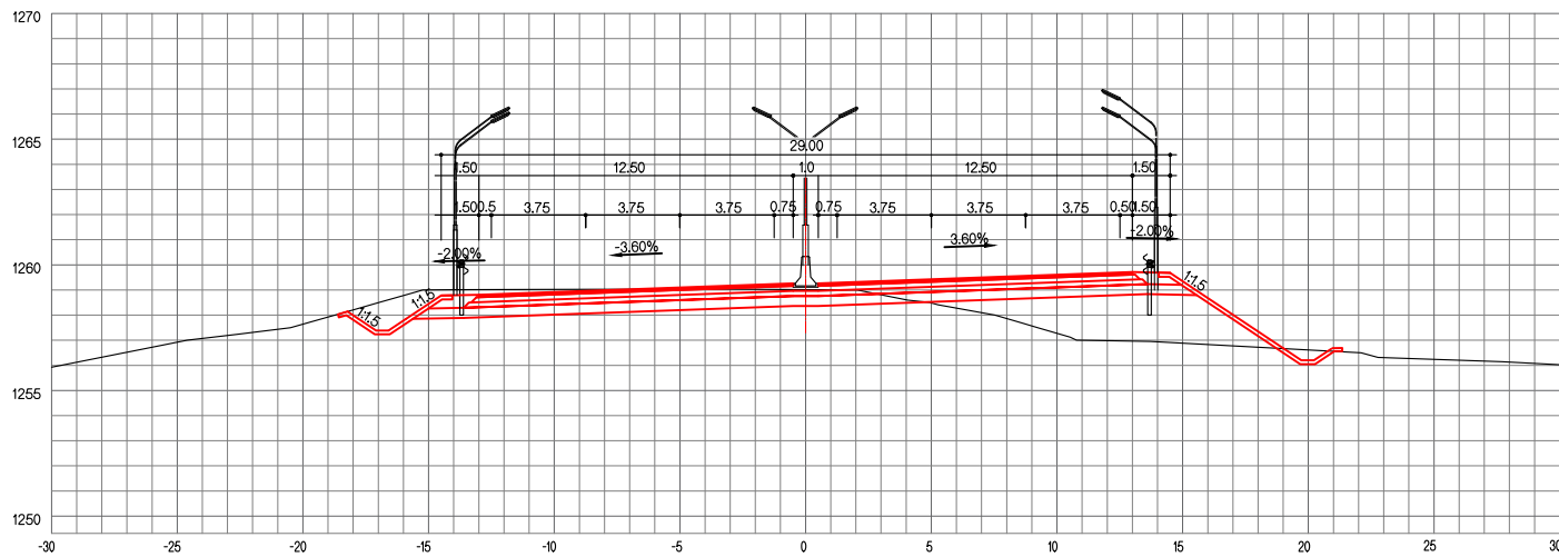
ЗАЙ / STA. 23+420.00
