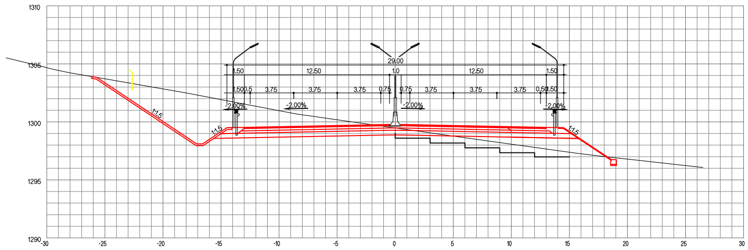
ЗАЙ / STA. 30+080.00
