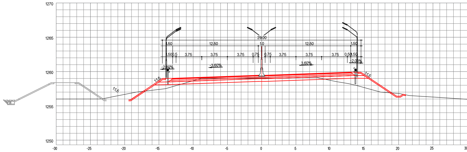
ЗАЙ / STA. 23+400.00
