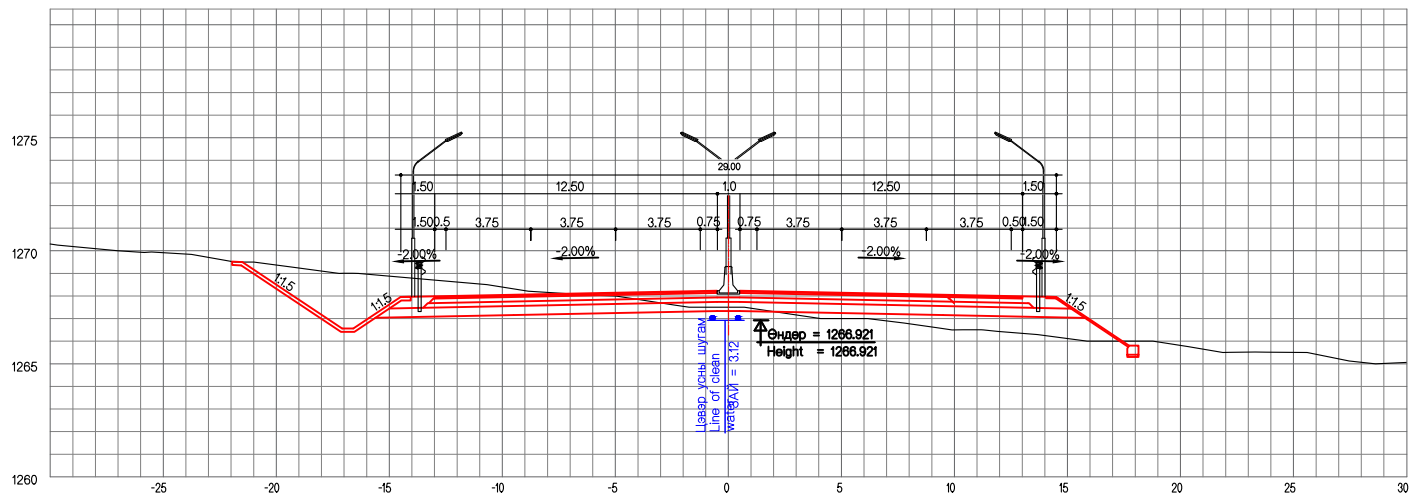
ЗАЙ / STA. 28+920.00
