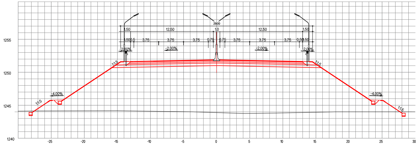
ЗАЙ / STA. 28+360.00
