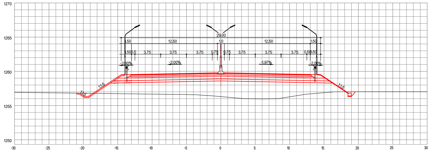
ЗАЙ / STA. 22+940.00
