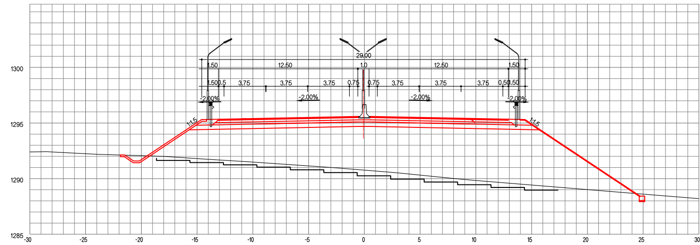
ЗАЙ / STA. 29+620.00
