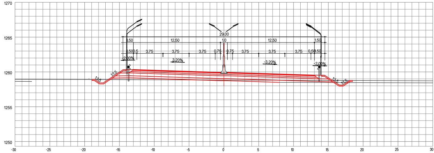
ЗАЙ / STA. 21+980.00
