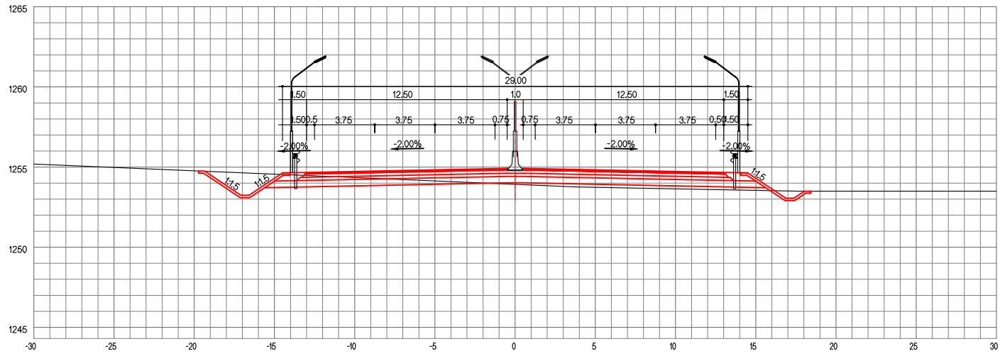
ЗАЙ / СТА. 24+240.00
