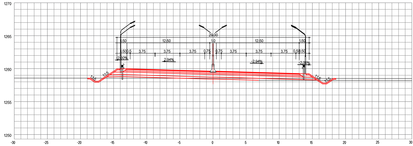
ЗАЙ / STA. 22+120.00
