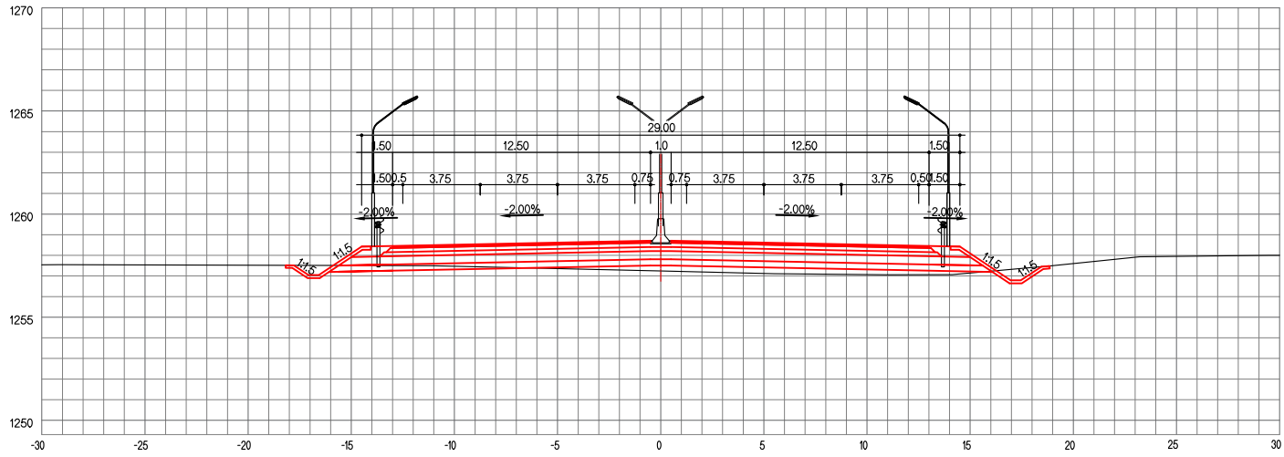
ЗАЙ / STA. 22+520.00
