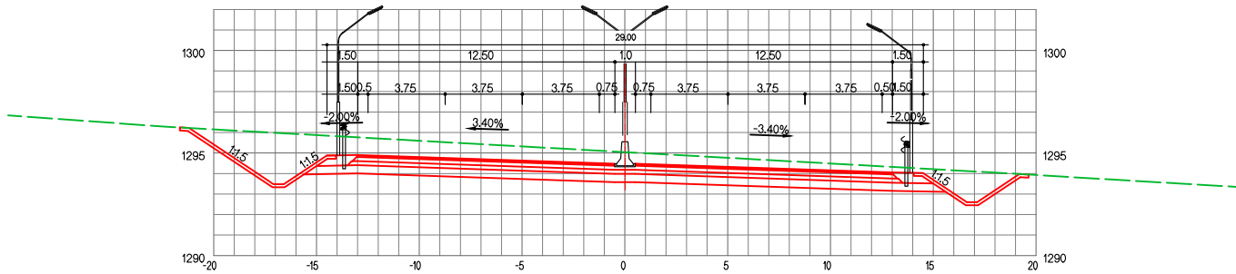
ЗАЙ / STA. 30+620.00
