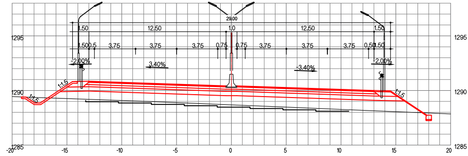
ЗАЙ / СТА. 30+820.00
