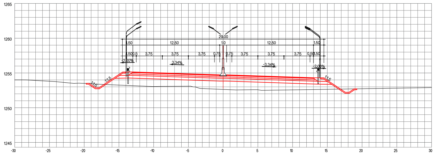
ЗАЙ / STA. 23+940.00
