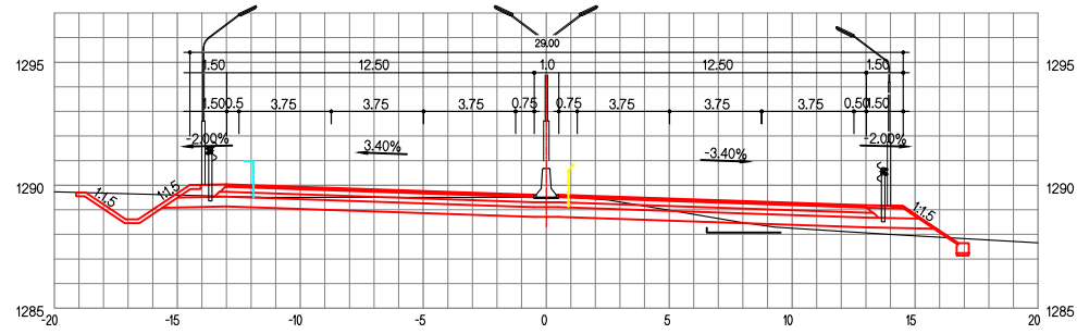
ЗАЙ / СТА. 30+860.00
