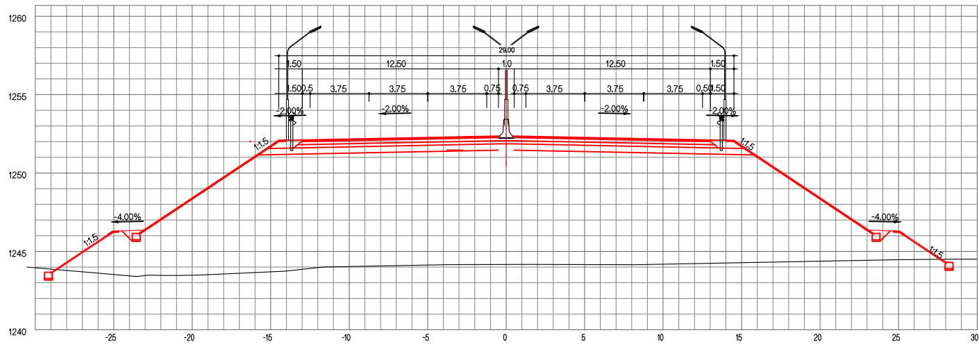
Зай / STA. 28+440.00
