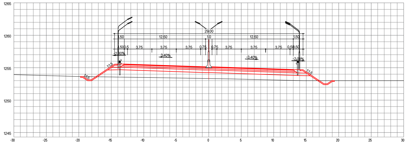
ЗАЙ / STA. 23+840.00
