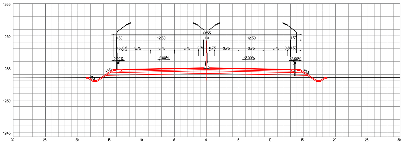
ЗАЙ / STA. 24+400.00
