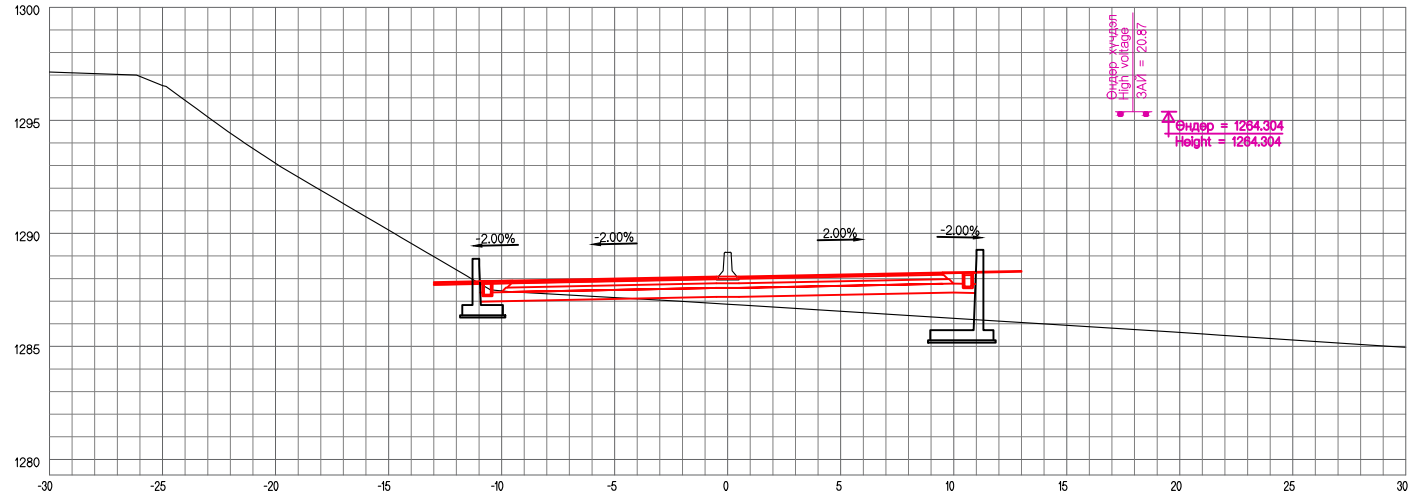
ЗАЙ / STA. 29+380.00
