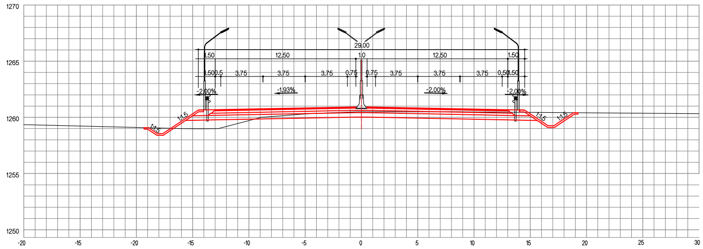
ЗАЙ / STA. 21+740.00
