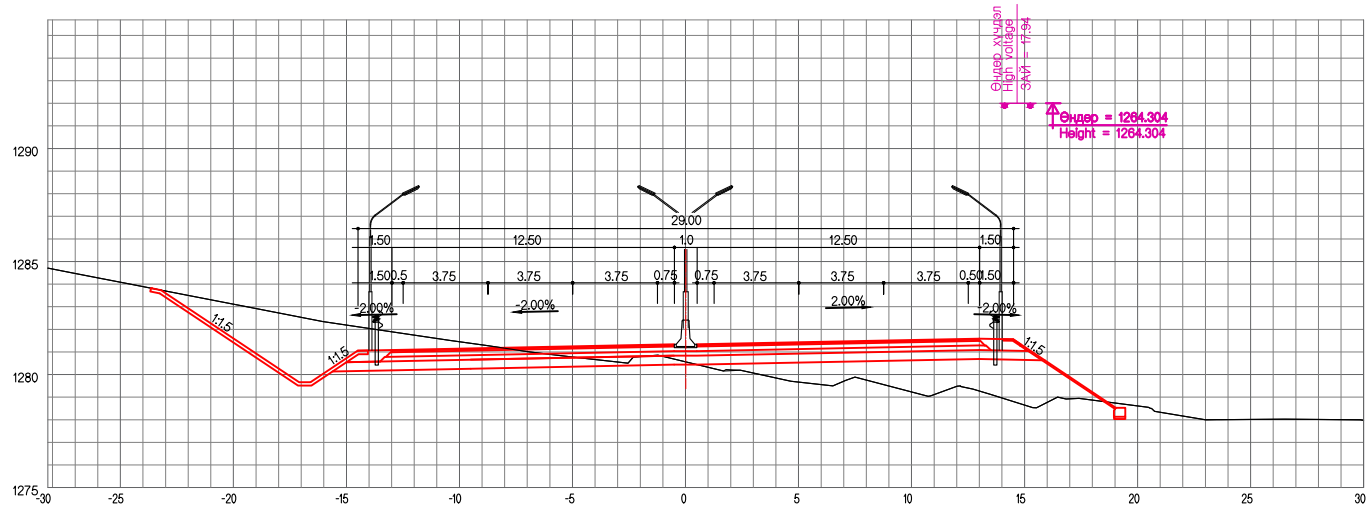
ЗАЙ / STA. 29+220.00
