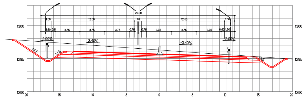
ЗАЙ / STA. 30+560.00
