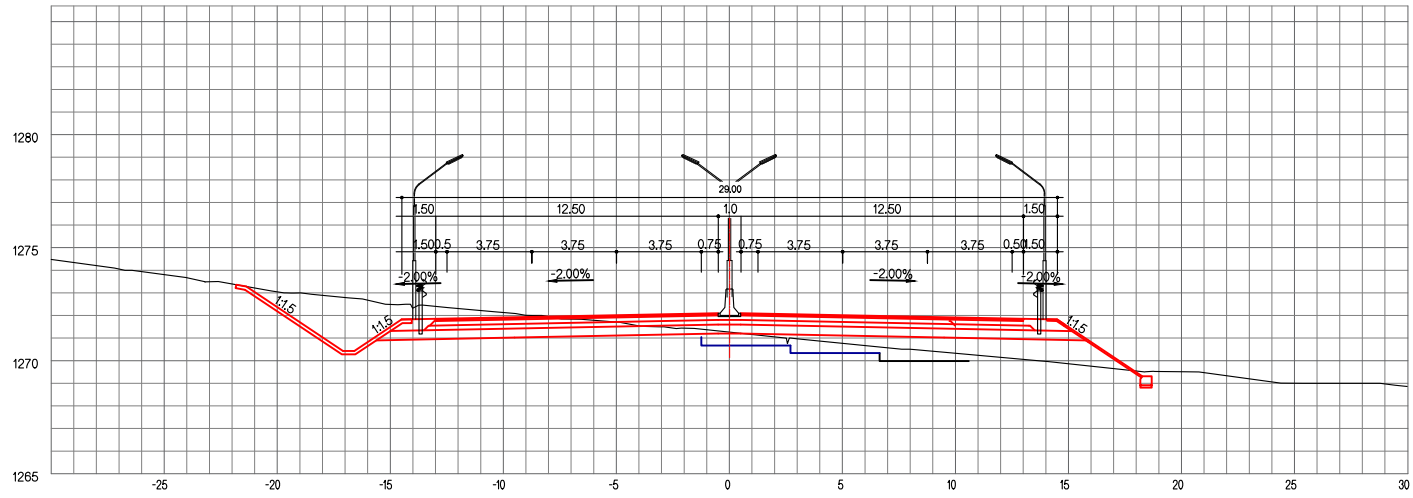
ЗАЙ / СТА. 29+040.00
