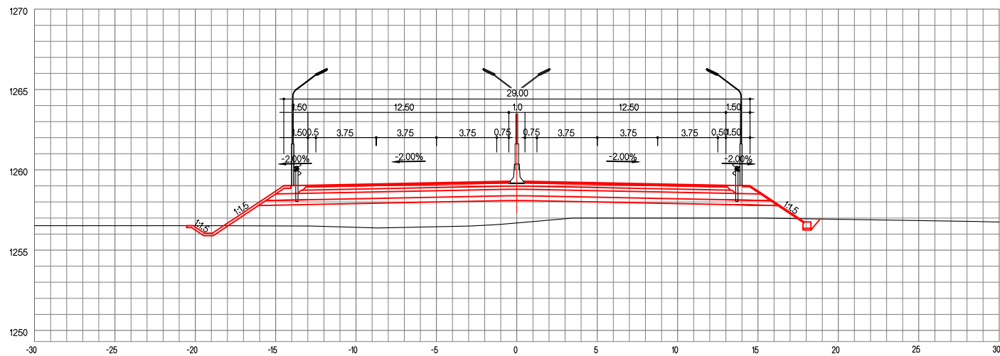
ЗАЙ / STA. 22+800.00
