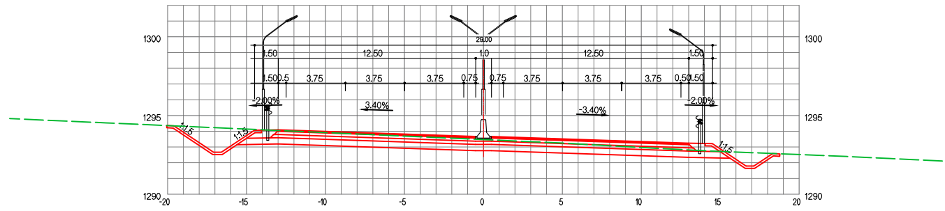
Зай / STA. 30+660.00
