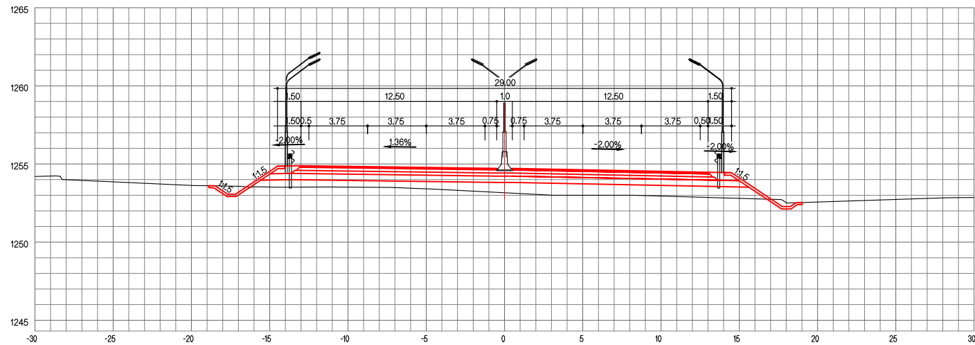
ЗАЙ / STA. 23+980.00
