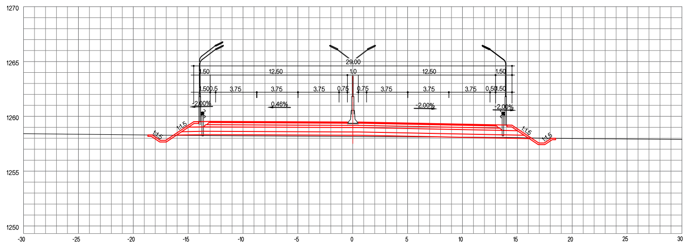
Зай / STA. 22+180.00
