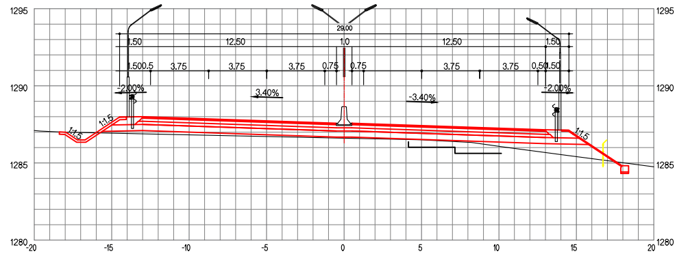
ЗАЙ / STA. 30+960.00
