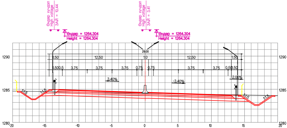
ЗАЙ / STA. 31+800.00
