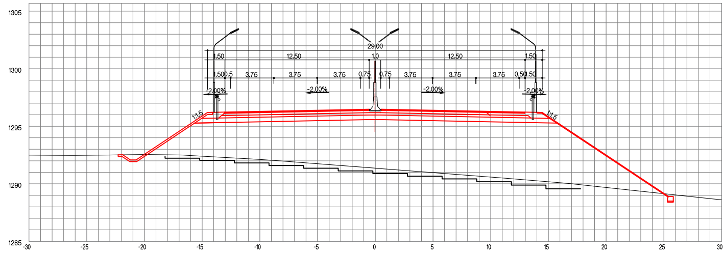
ЗАЙ / СТА. 29+660.00
