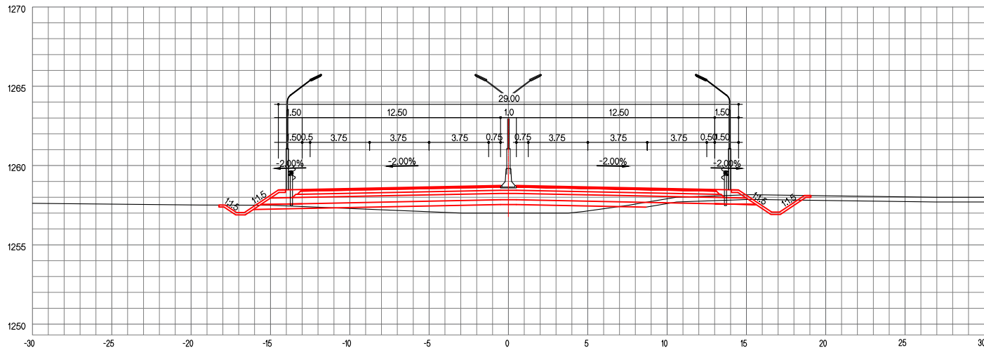
ЗАЙ / STA. 22+500.00
