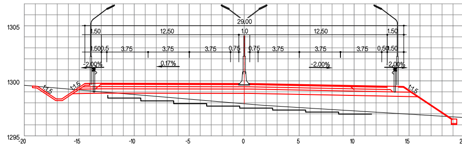
Зай / STA. 30+360.00
