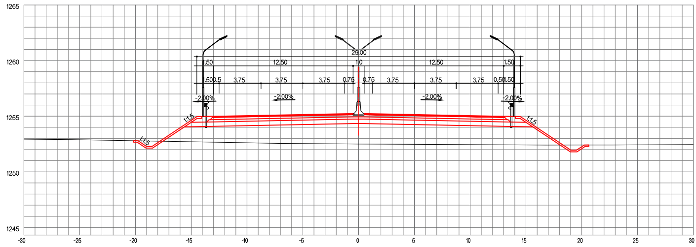
ЗАЙ / STA. 24+680.00
