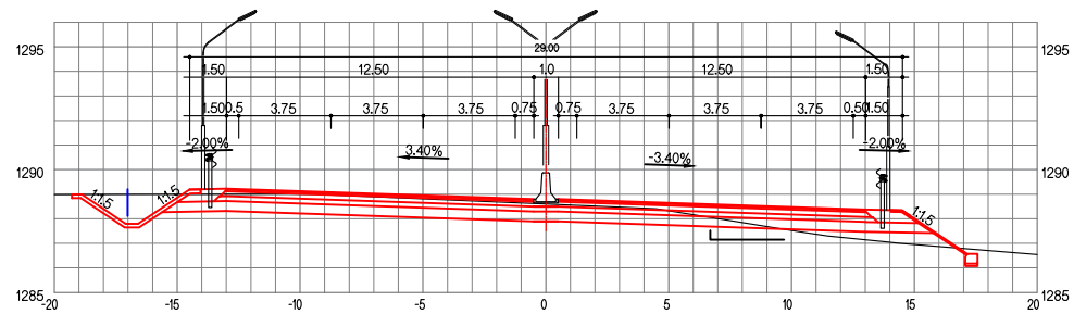
ЗАЙ / STA. 30+900.00
