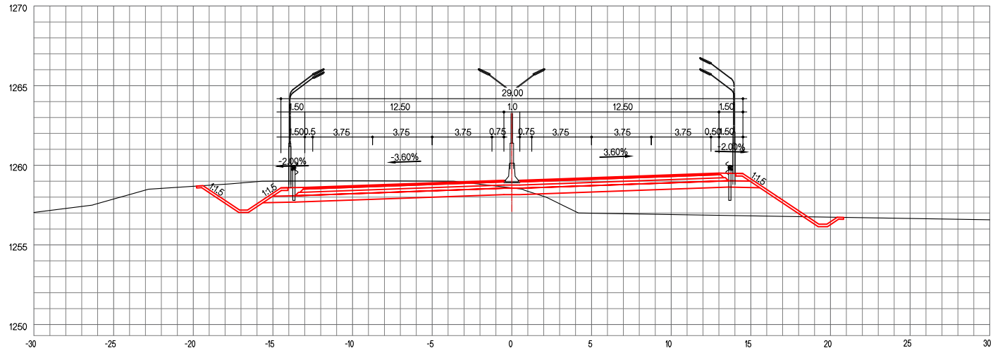
ЗАЙ / STA. 23+440.00
