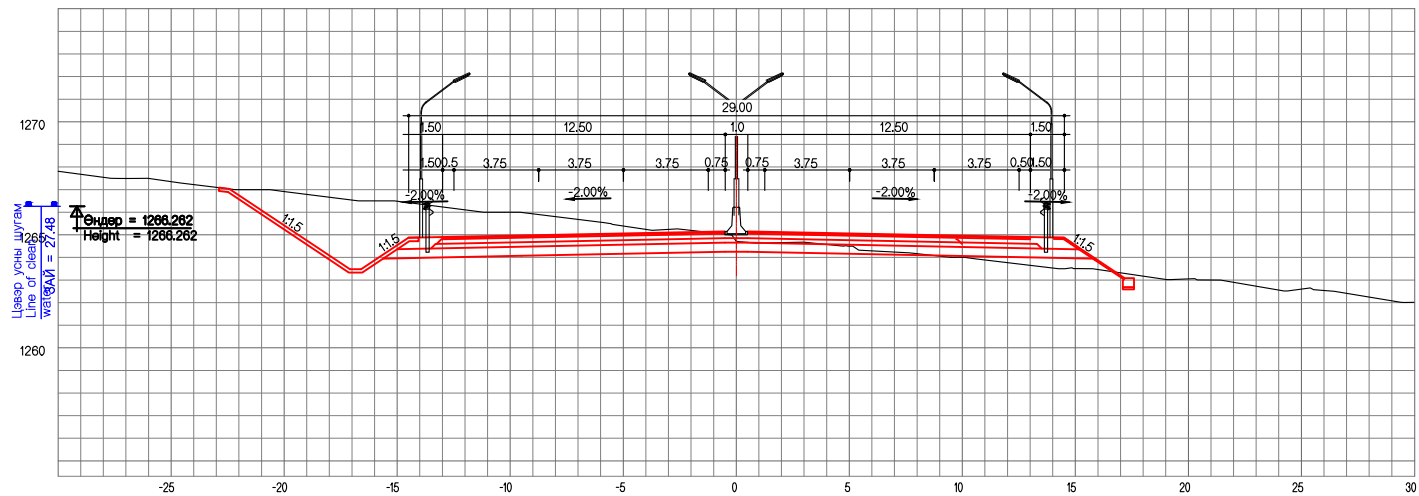
ЗАЙ / STA. 28+840.00
