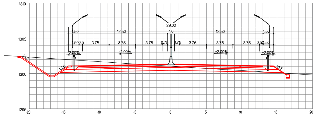
ЗАЙ / STA. 30+280.00
