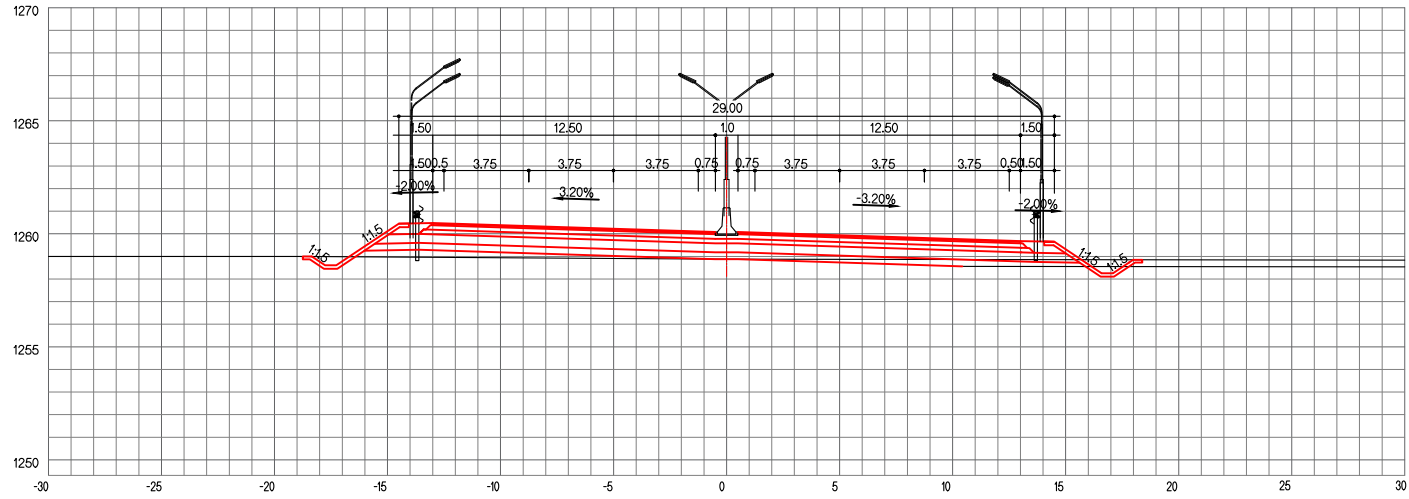
Зай / STA. 21+920.00
