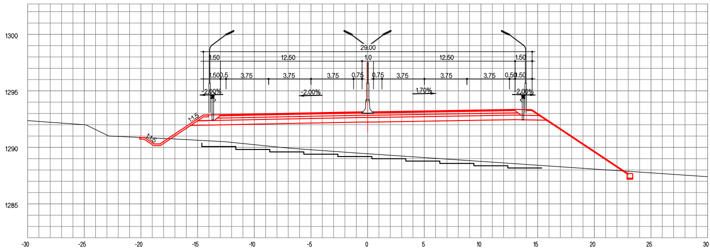
ЗАЙ / СТА. 29+540.00
