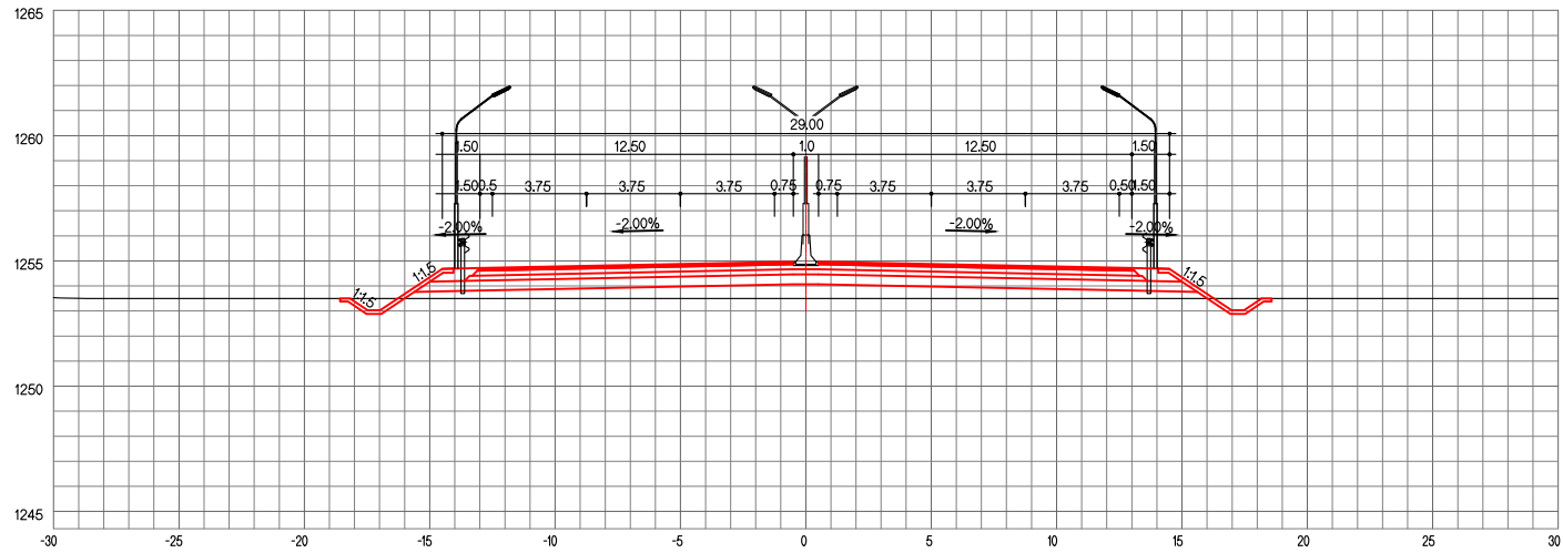
ЗАЙ / STA. 24+300.00
