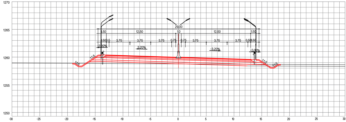
ЗАЙ / STA. 21+960.00
