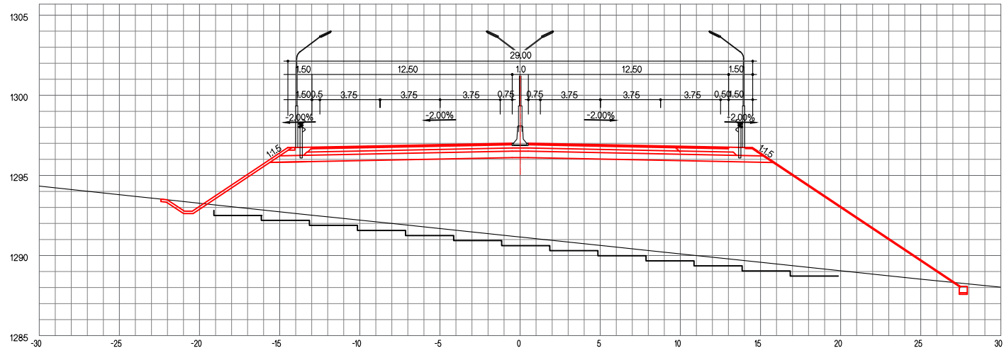
ЗАЙ / STA. 29+800.00
