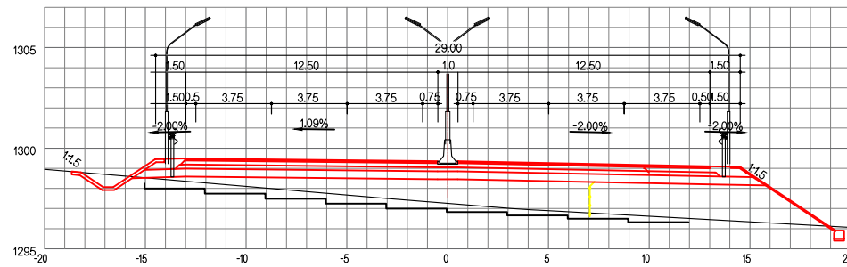
Зай / STA. 30+380.00
