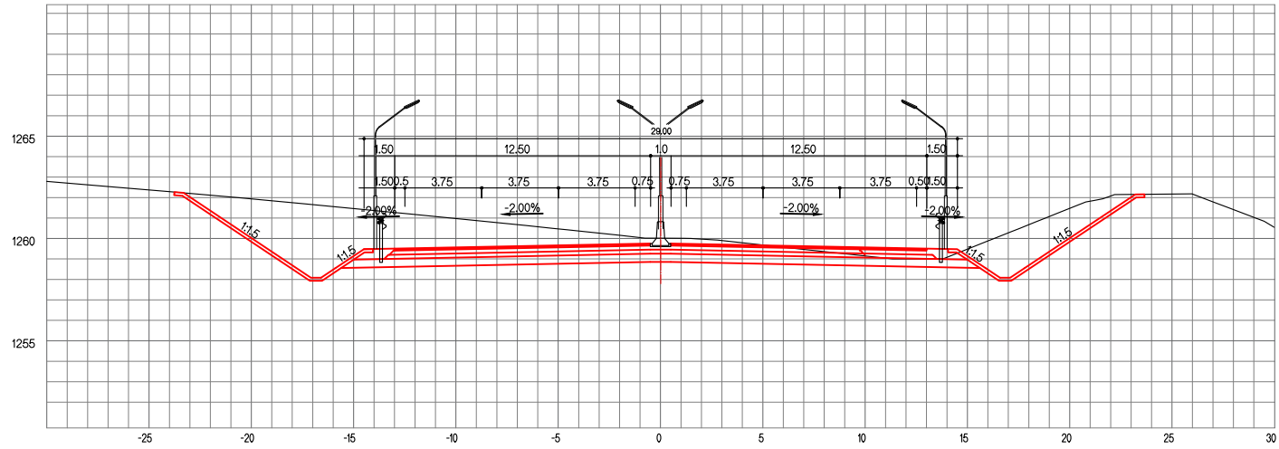
ЗАЙ / STA. 28+720.00
