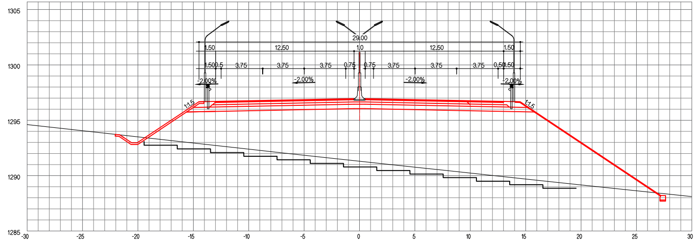
ЗАЙ / STA. 29+820.00
