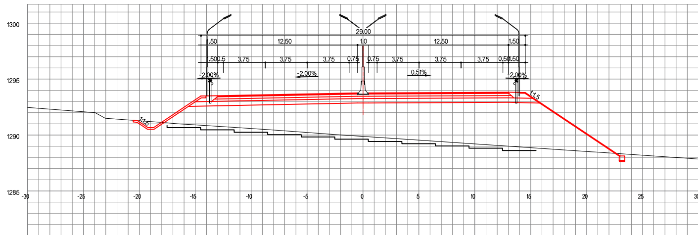
ЗАЙ / STA. 29+560.00
