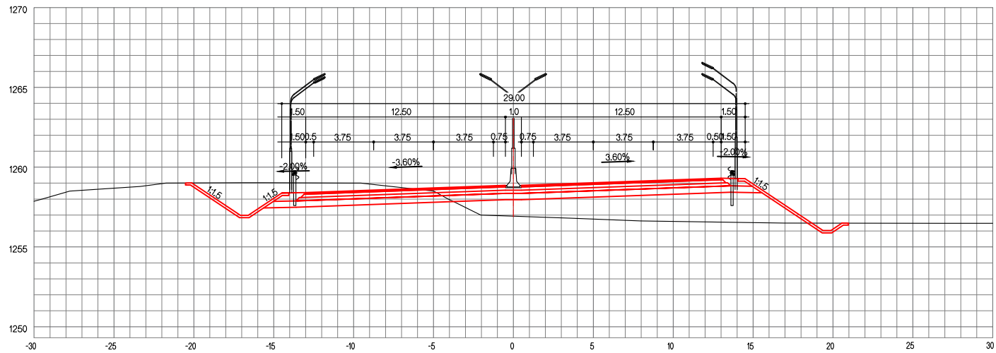
ЗАЙ / STA. 23+460.00
