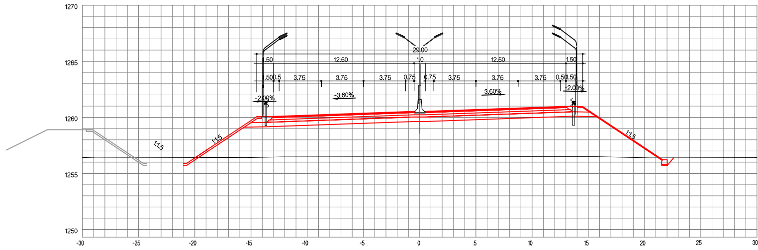
ЗАЙ / СТА. 23+240.00
