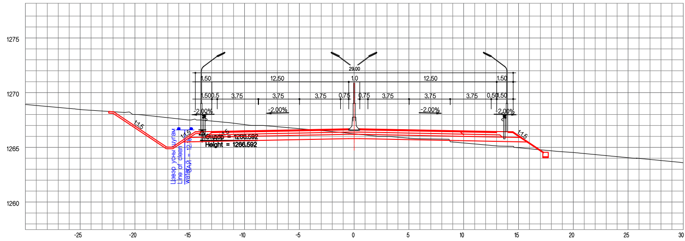
ЗАЙ / STA. 28+880.00
