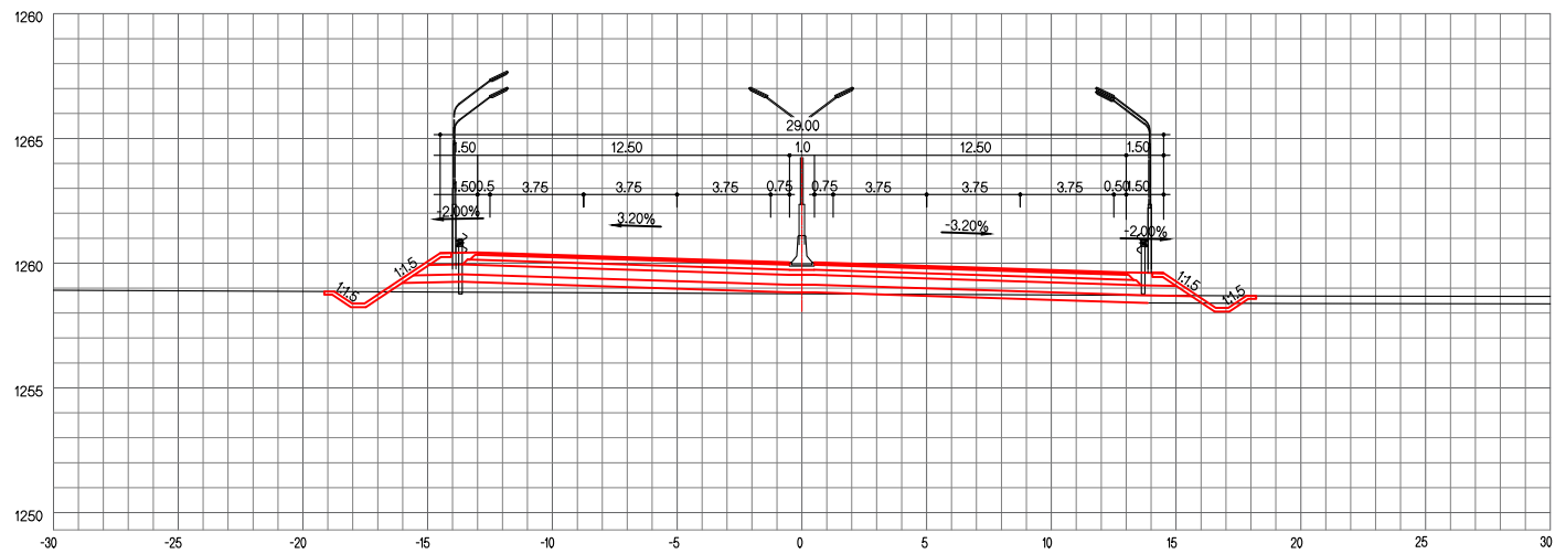
Зай / STA. 21+940.00
