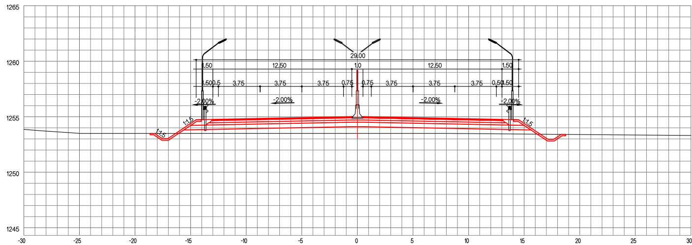
ЗАЙ / STA. 24+360.00
