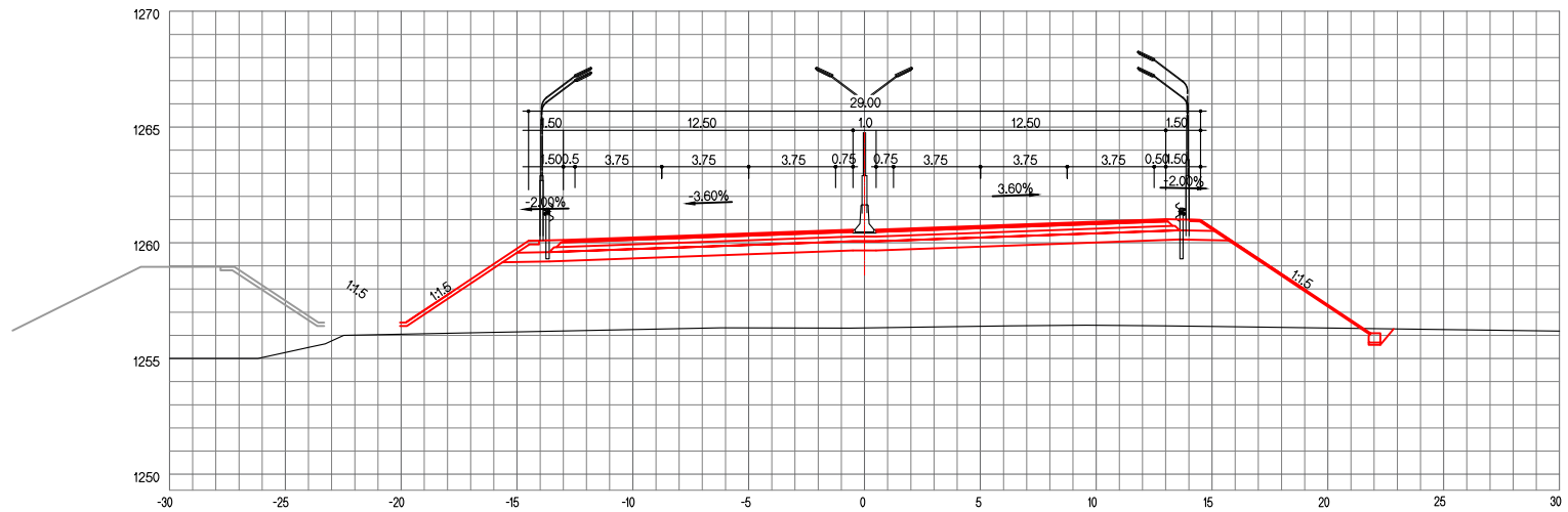
ЗАЙ / STA. 23+220.00
