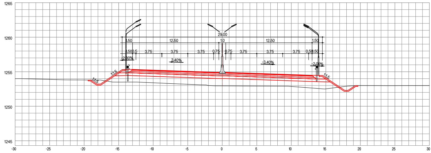
ЗАЙ / STA. 23+880.00
