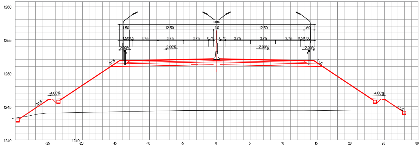
ЗАЙ / STA. 28+420.00
