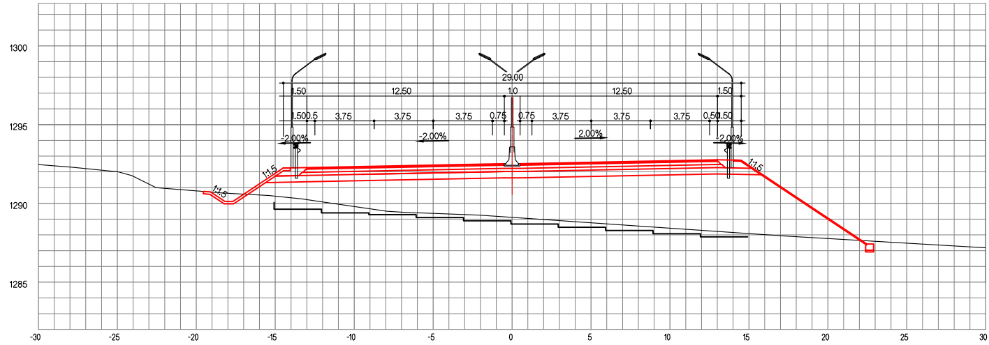
ЗАЙ / СТА. 29+520.00
