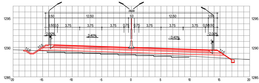
ЗАЙ / СТА. 30+840.00
