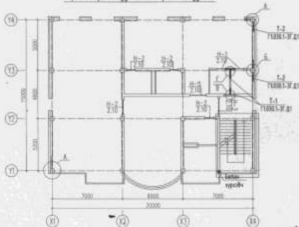
3-р давхарын ялуу ханын торны байгуулалт
