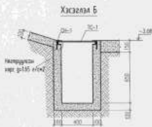
Гайна довтолго ГД-1 ийм байгуулалт
