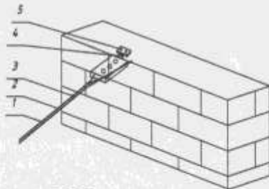
Тайлбар 1- кабель, 2- өлгөн прос, 3- кабель өлгөн бэхлэгээ, 4- гогоцоо, 5- бэхлэгээ дэвээ
