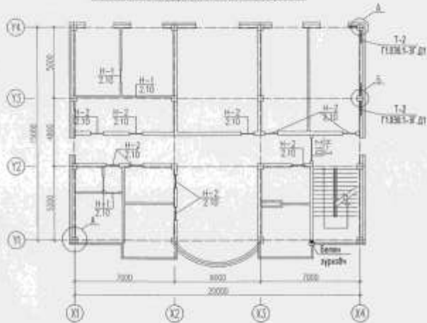
2-р давхарын ялуу ханын торны байгуулалт
