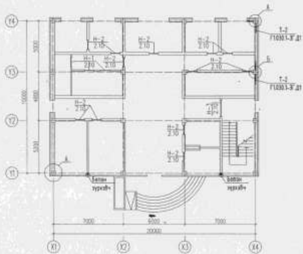
1-күбүрүмдүн аягуу канын торны байгуулалы
