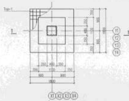
Боломн сүүрч БС-1
