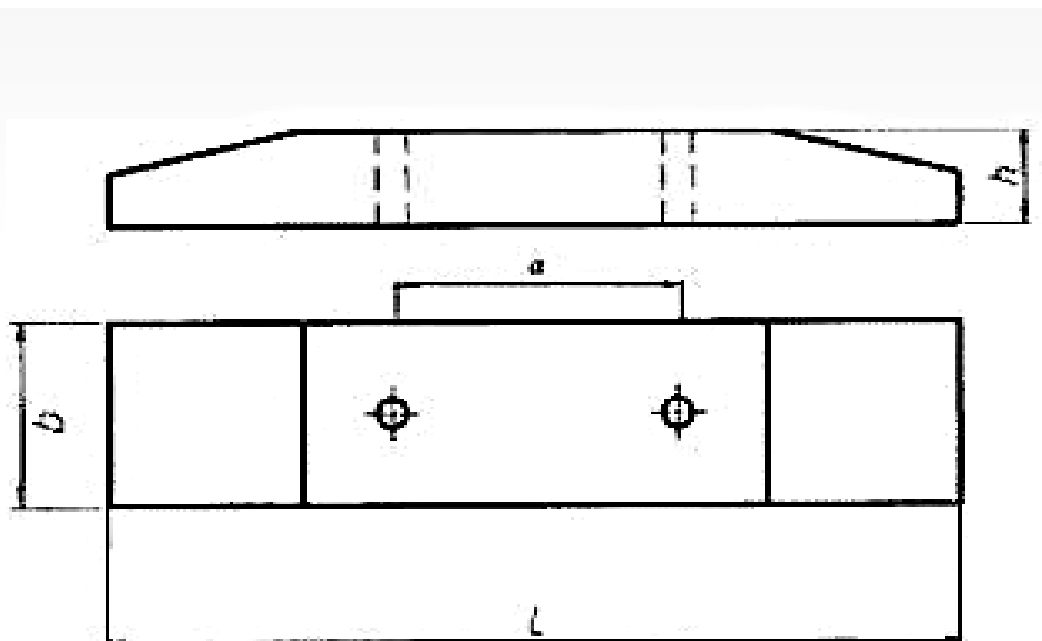
AP 5 чагт /ригель/-ийн хийцийн хэмжээсүүд
