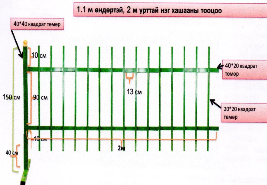
Зураг: Хашааны загварын зураг
