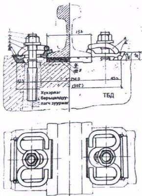
ЗУРАГТ. P-50 ЗАМ ТӨМӨРТЭЙ ГАЗРЫН ҮЕНИЙ ДУНД ХЭСГИЙН БЭХЭЛГЭЭНИЙ УГСРАГДСАН БАЙДАЛ: 1-босо боолт, 2-гайка, 3-хавтгай шайба 4-пүрш, 5-хавтгай уян даруулга, 6-уян даруулганы суудал, 7-зөөлөч, 8-хулсан нэгэс
