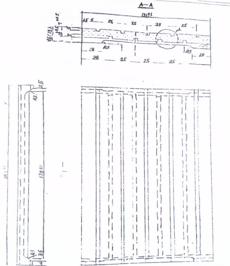
ЗУРАГ 10. Р 50 ЗАМ ТӨМӨРТ ХЭРЭГЛЭХ РЕЗИН ЗӨӨЛӨВЧ
