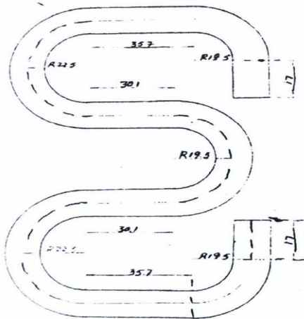
В. Дээрээс харсан зураг
