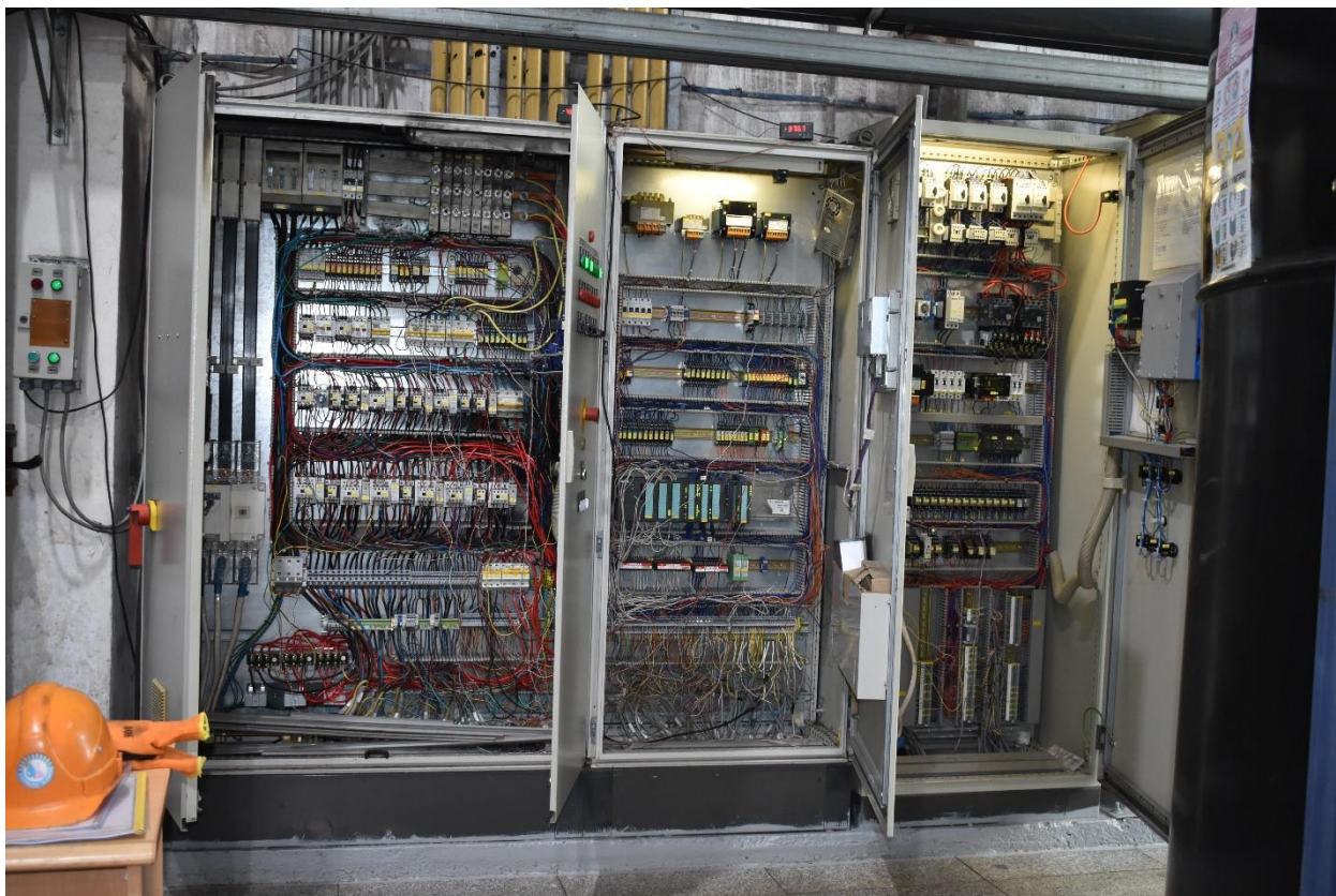
Зураг 2. Хими ус бэлтгэлийн удирдлагын хэлхээний монтаж
