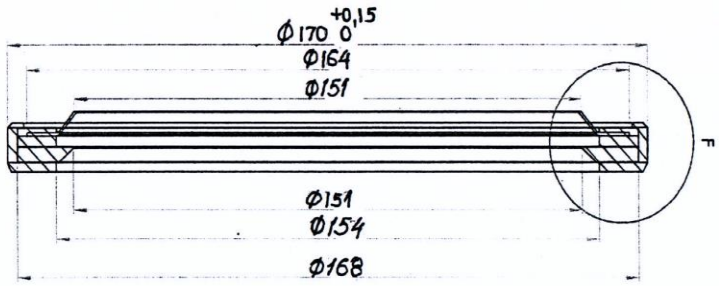
SECTION D-D SCALE 1 : 1
