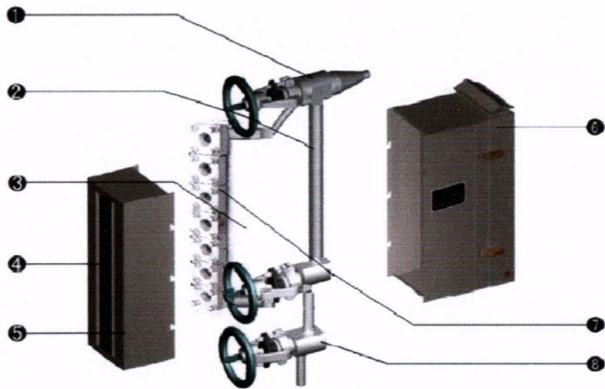
1-Уурын хаалт 2-Уур усан гэмцүүлэгч 3-Усны хаалт 4-Түвшин заагч 5-Нүүрийн гэрэлтүүлгийн хайрцаг 6-Арын гэрэлтүүлгийн хайрцаг 7-Их бие 8-Дренаж
