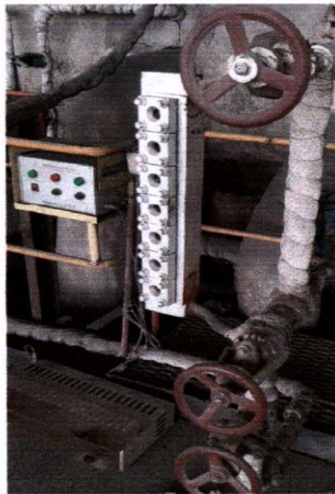
1-Уурын хаалт 2-Уур усан гэмцүүлэгч 3-Усны хаалт 4-Түвшин заагч 5-Нүүрийн гэрэлтүүлгийн хайрцаг 6-Арын гэрэлтүүлгийн хайрцаг 7-Их бие 8-Дренаж
