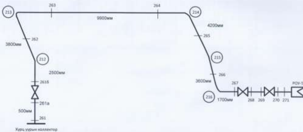
Турбин II цехийн РОУ-5-н хурц уурын шугам хоолой
