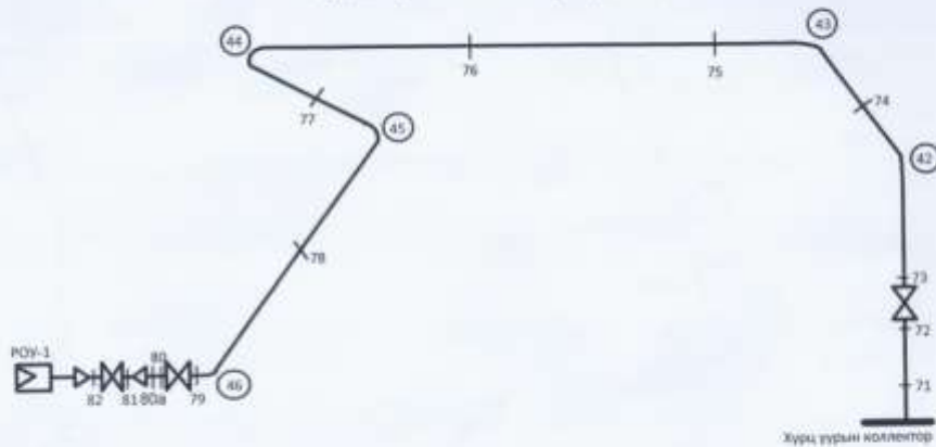
Турбин II цехийн РОУ-1-н хурц уурын шугам хоолой
