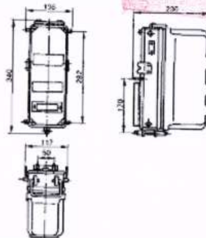
Рис. 155. Блок управления кабеля электрической оптической связи
