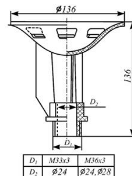
Рис. 1. Форсунка с чашечным отрожателем - для градиент капельно-пленочного типа
