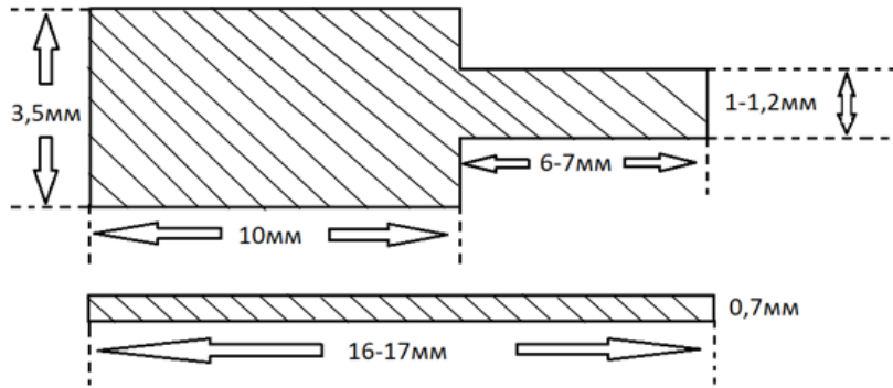
Зураг 4. Тоолуурын батарей холбогч шонгийн хэмжээ
