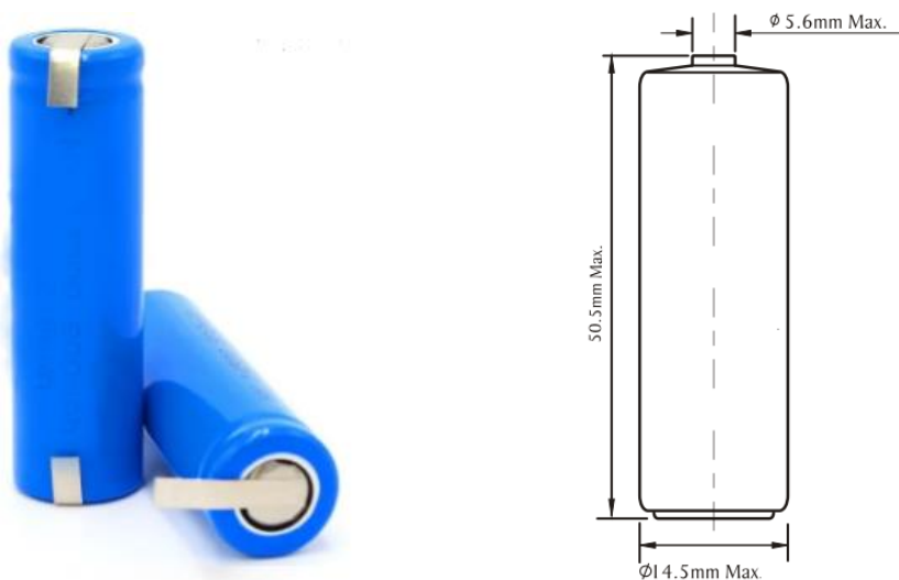
Зураг 2. AM-360 маркийн тоолуурт хэрэглэгдэх батарейны зураг
