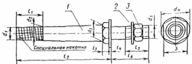
1—штырь; 2—шайба; 3—гайка.
