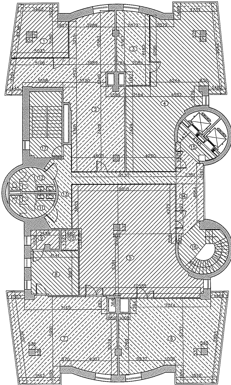
5-Р ДАВХРЫН ХЭМЖИЛТИЙН БАЙГУУЛАЛТ М1:150
