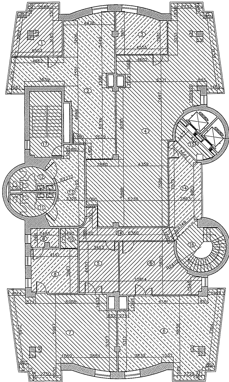
6-Р ДАВХРЫН ХЭМЖИЛТИЙН БАЙГУУЛАЛТ /ОДОО БАЙГАА/ М1:150
