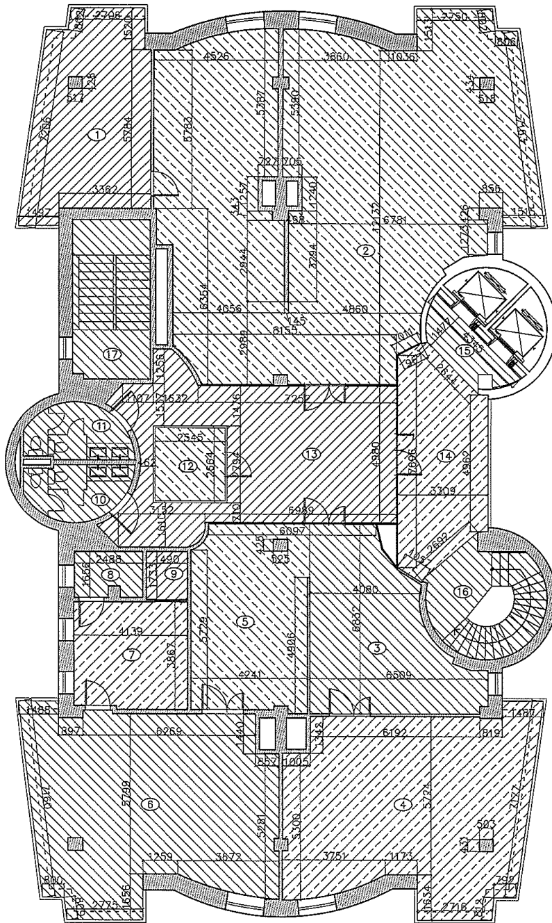
7-Р ДАВХРЫН ХЭМЖИЛТИЙН БАЙГУУЛАЛТ М1:150
