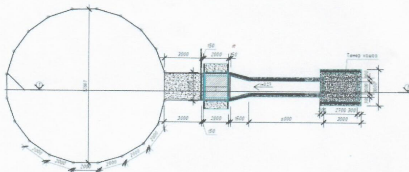
9.2 Ванны арматурын зураг
